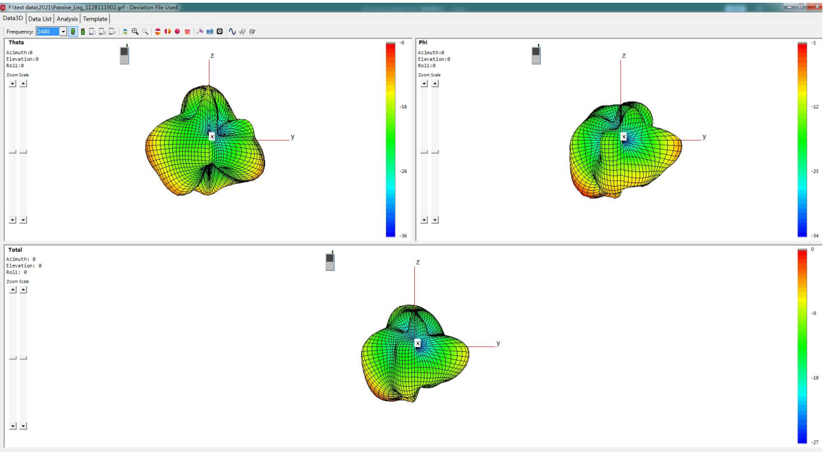
3D辐射图（3D radiation chart）
