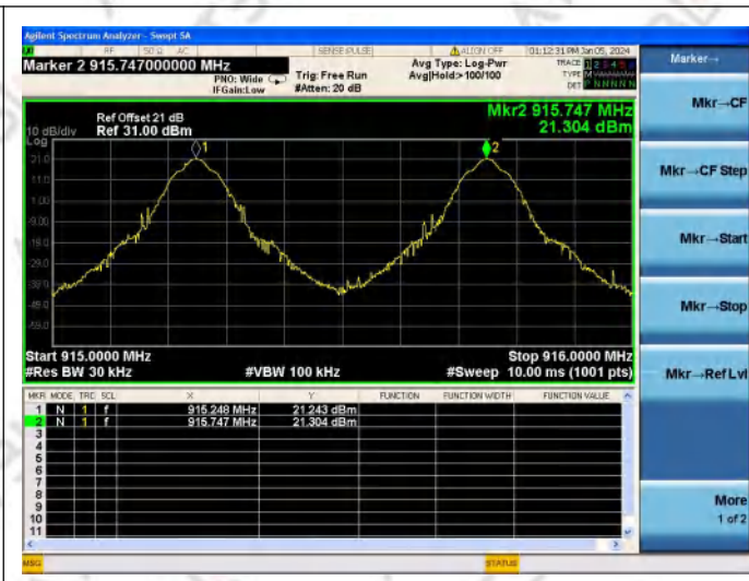
CH25
