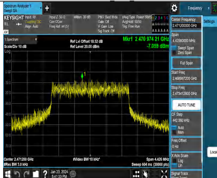
3MCA MIMO_Ant3_2471.2
