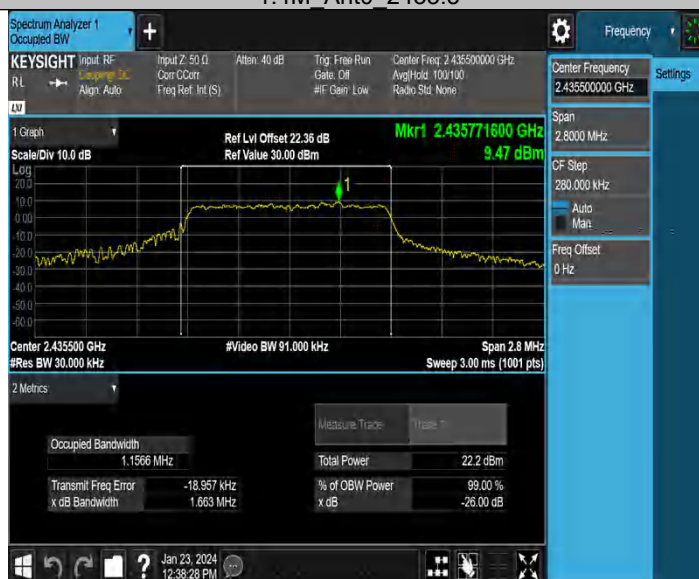
1.4M Ant0 2435.5
