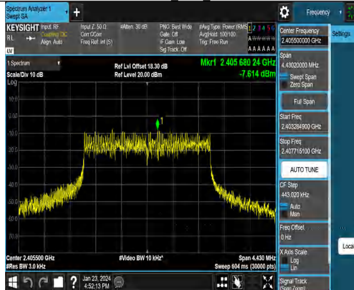
3M MIMO_Ant3_2405.5
