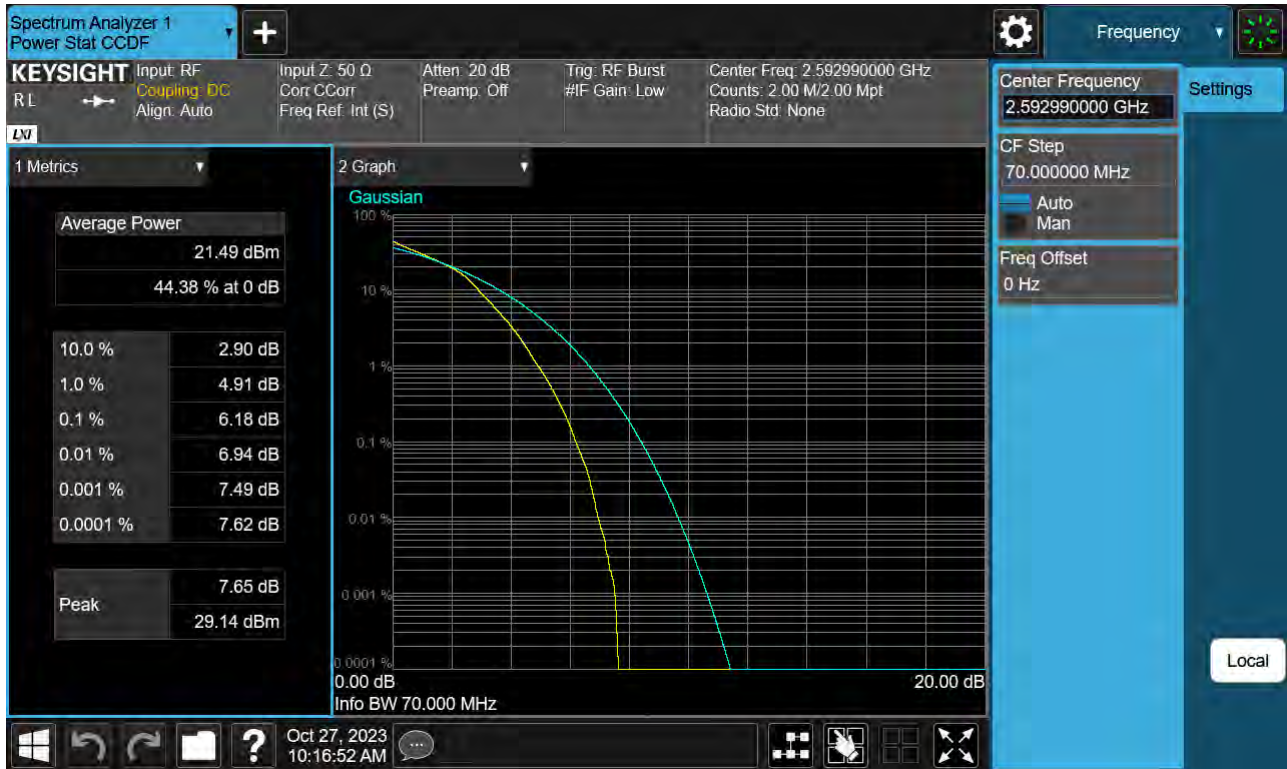
Sub6 n41. PAR Plot (70 M BW_Ch.518598_16QAM)
