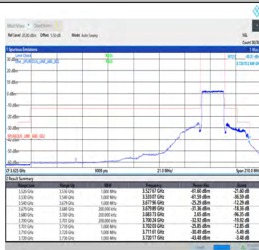
Band43_20MHz_QPSK_43690_100RB#0
