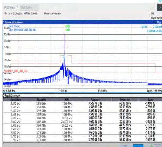
Band43 5MHz QPSK 43615 1RB#0
