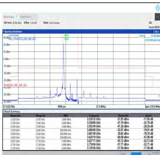
Band43_20MHz_QPSK_43690_1RB#0
