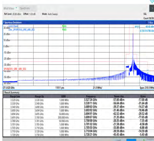
Band43 5MHz QPSK 44565 1RB#24
