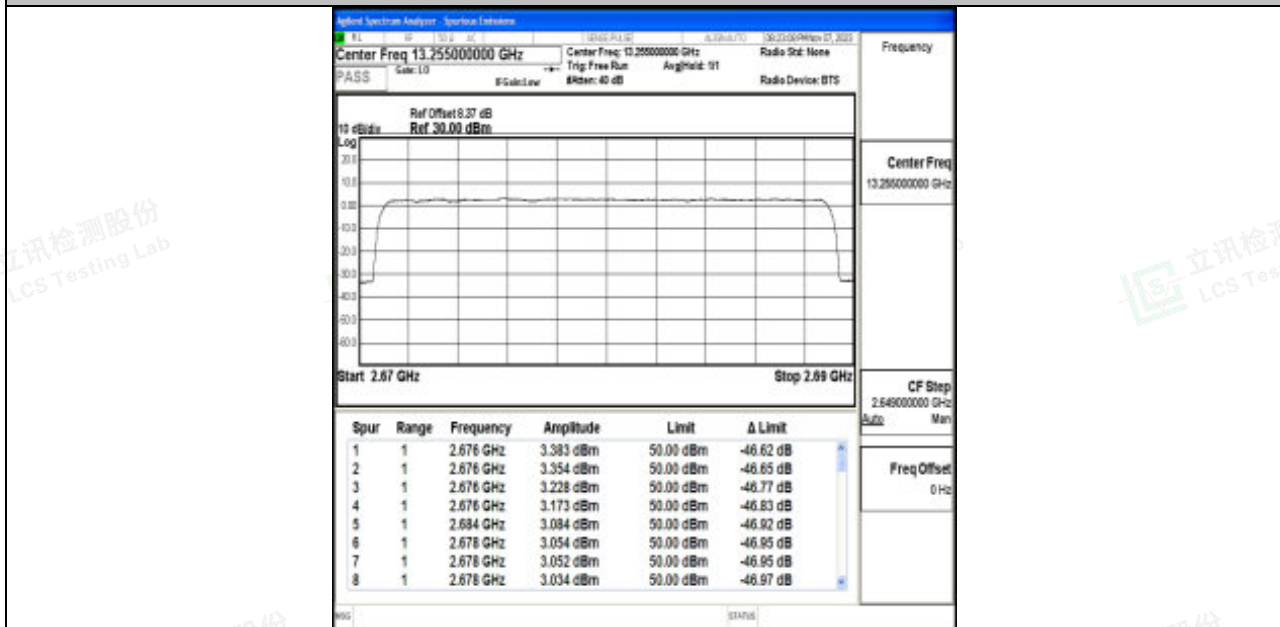
Band41_20MHz_QPSK_41490_100RB#0
