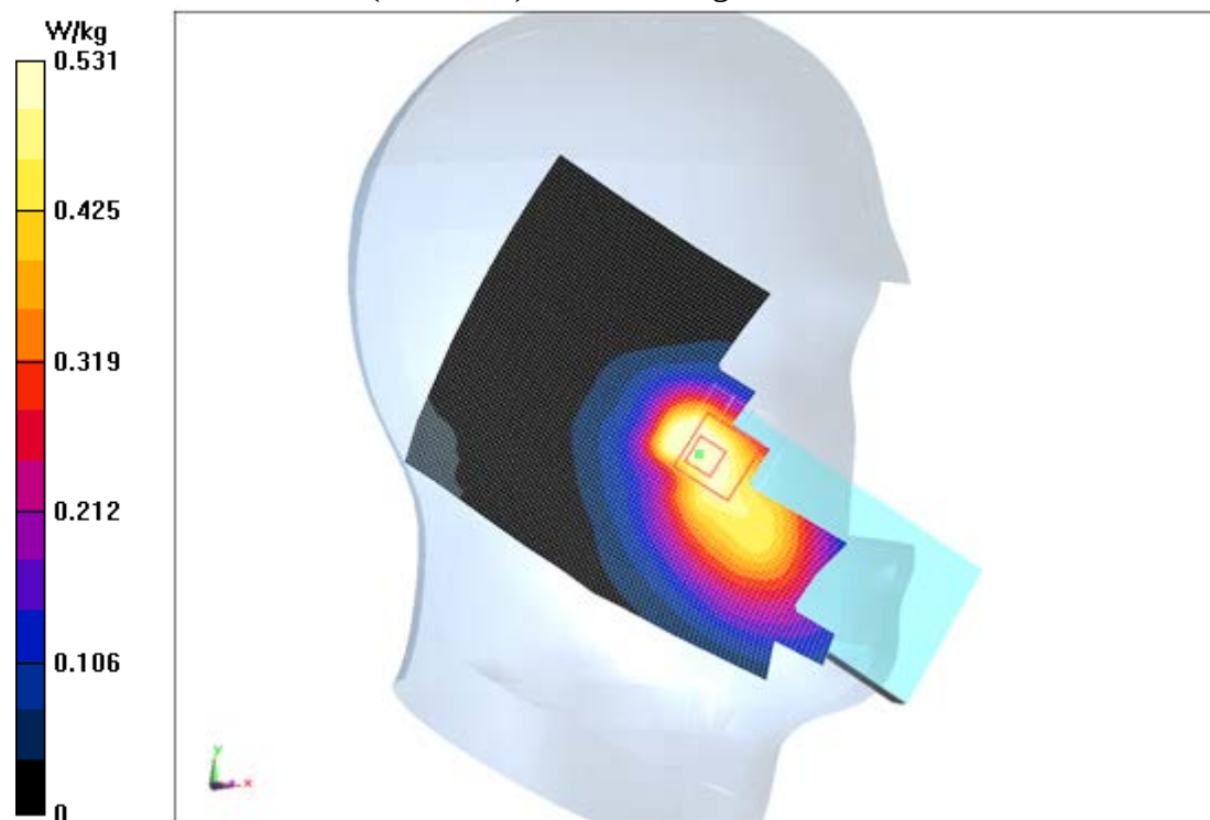
Fig.5 WCDMA 850
