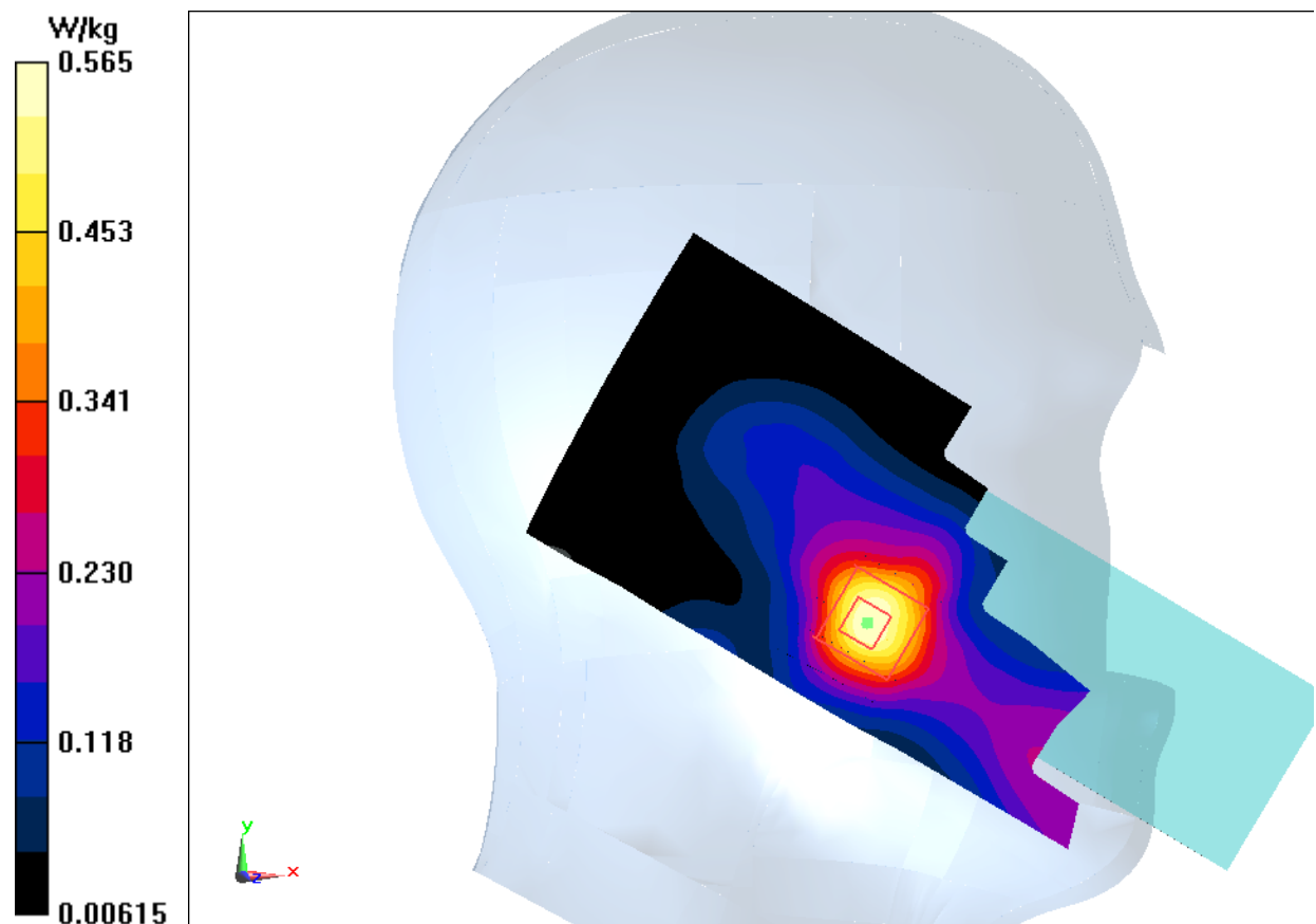
Fig.7 WCDMA1700
