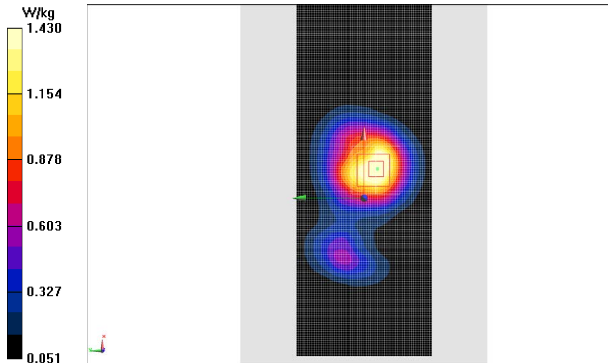
Fig.8 WCDMA1700
