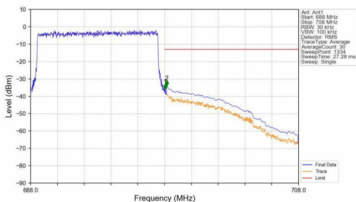
Band71 10MHz 16QAM HCH 693MHz RB 50 0 NTV
