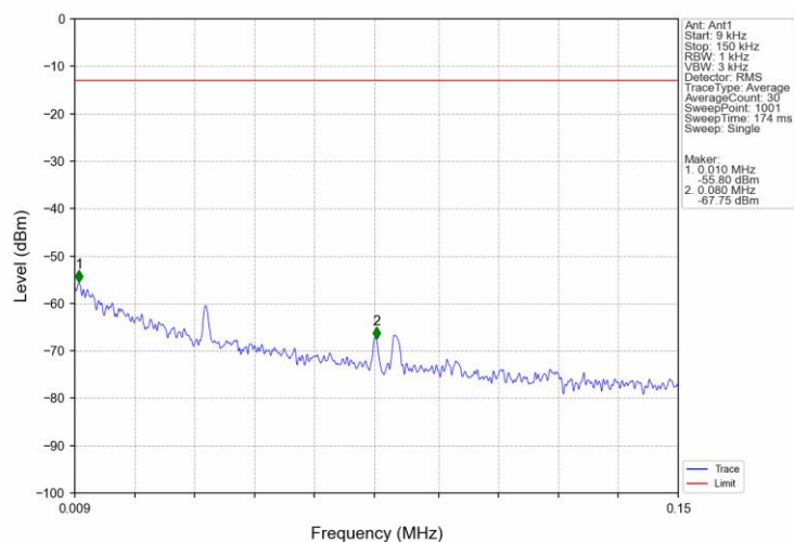
Band71 20MHz QPSK MCH 683MHz RB 1 0 NTN
