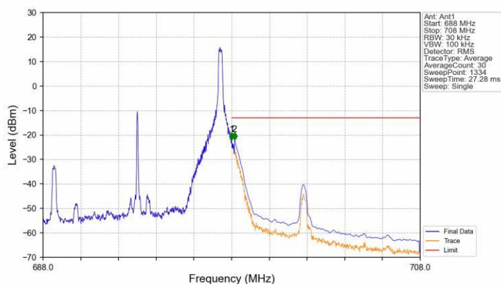
Band71 10MHz 16QAM HCH 693MHz RB 1 49 NTV
