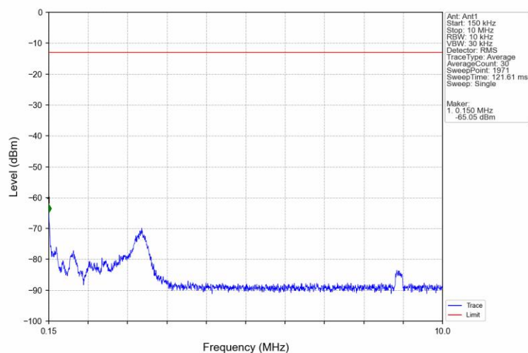
Band71_20MHz_QPSK_LCH_673MHz_RB_1_0 NTN
