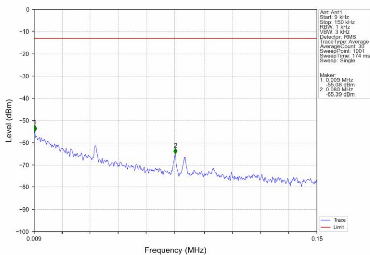
Band71_10MHz_QPSK_LCH_668MHz_RB_1_0_NTNV
