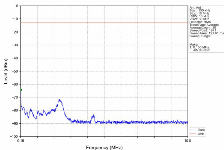
Band71_10MHz_QPSK_LCH_668MHz_RB_1_0_NTNV
