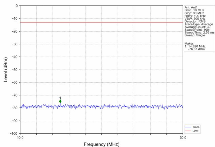
Band71_10MHz_QPSK_LCH_668MHz_RB_1_0_NTNV
