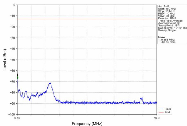
Band71 20MHz QPSK MCH 683MHz RB 1 0 NTN
