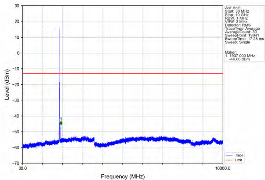
Band2_10MHz_QPSK_LCH_1855MHz_RB_1_0_NTNV
