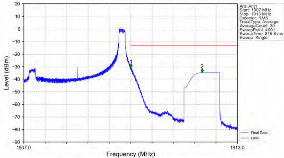
Band2_3MHz_QPSK_HCH_1908.5MHz_RB_1_14_NTNV
