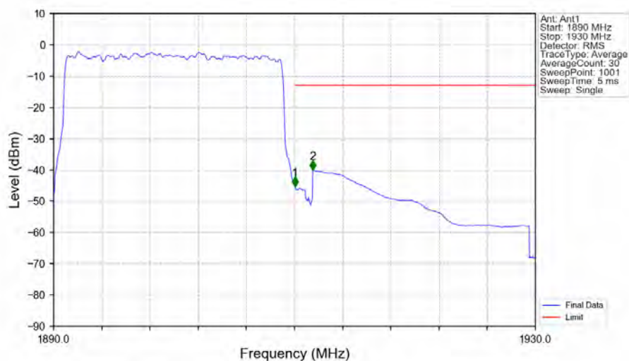
Band2_20MHz_QPSK_HCH_1900MHz_RB_100_0_NTNV
