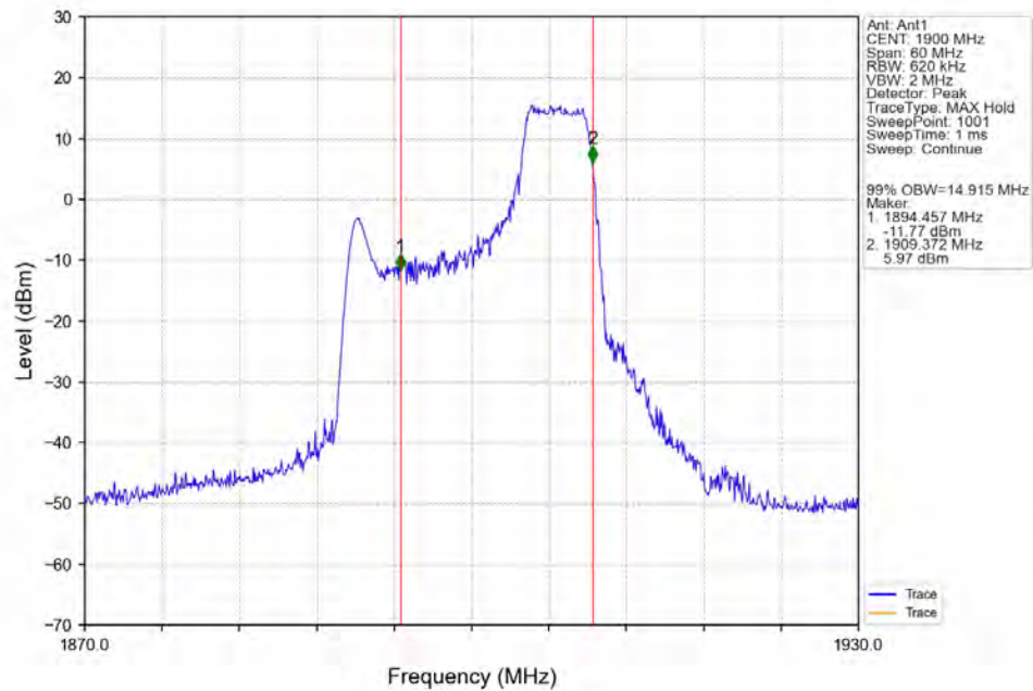
Band2_20MHz_16QAM_HCH_1900MHz_RB_27_73_NTNV
