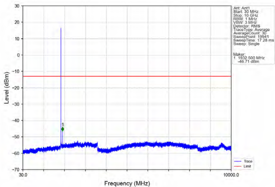
Band2_3MHz_QPSK_LCH_1851.5MHz_RB_1_0_NTNV
