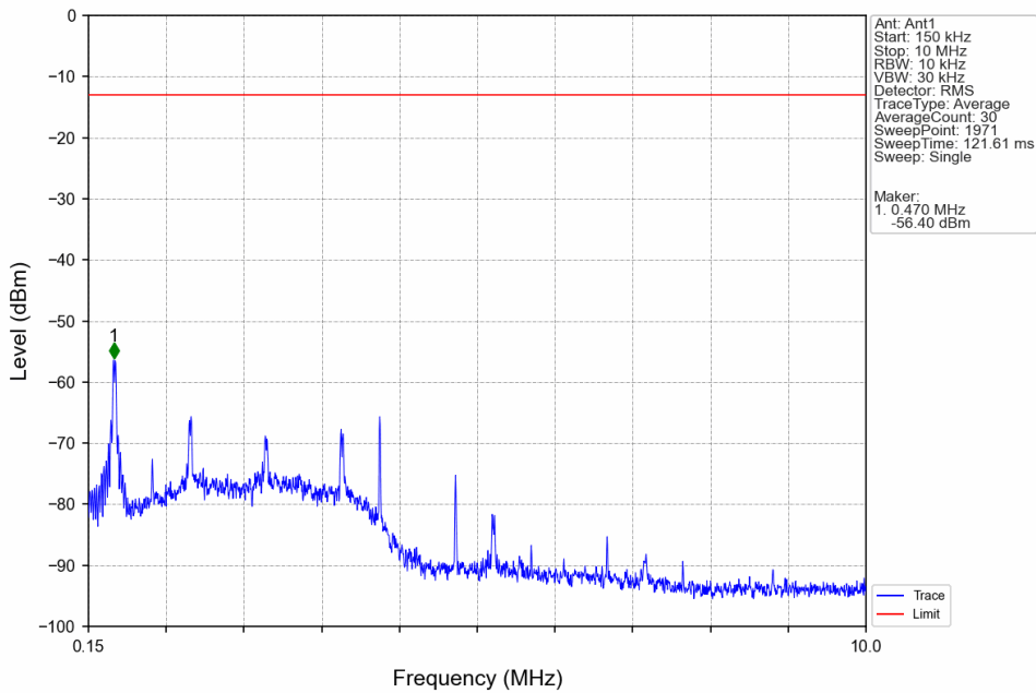
Band5_HSUPA_MCH_836.6MHz_Subtest 1_NTNV
