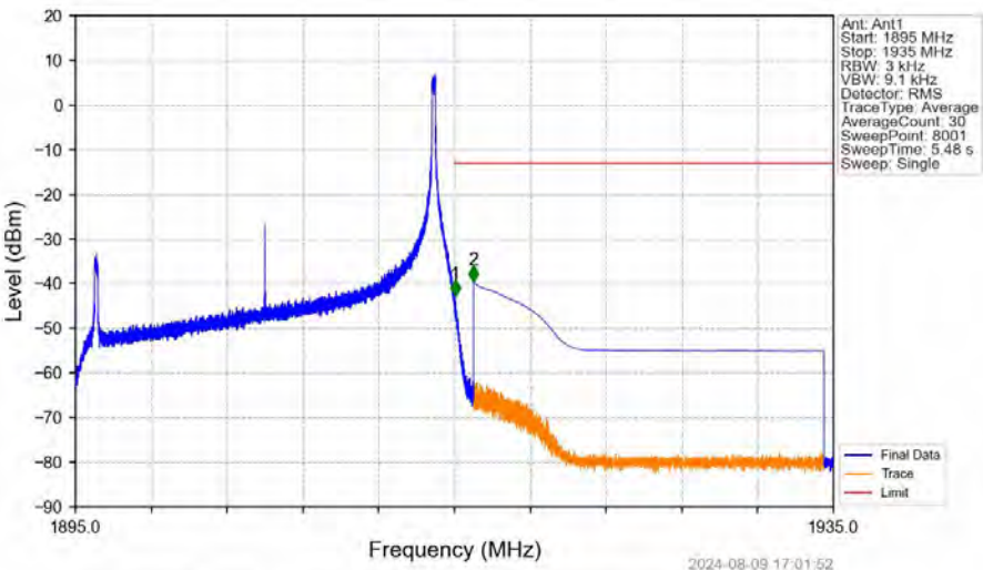
Band25_20MHz_QPSK_HCH_1905MHz_RB_1_99_NTNV
