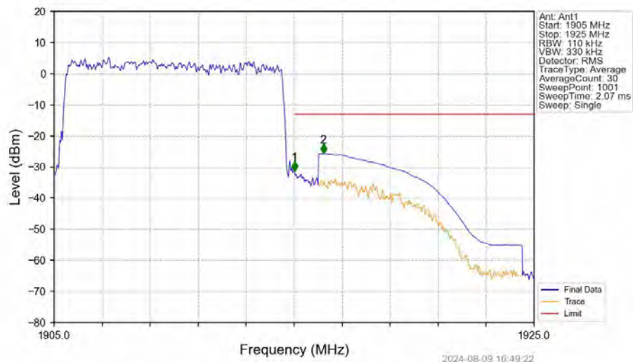
Band25_10MHz_QPSK_HCH_1910MHz_RB_50_0_NTNV
