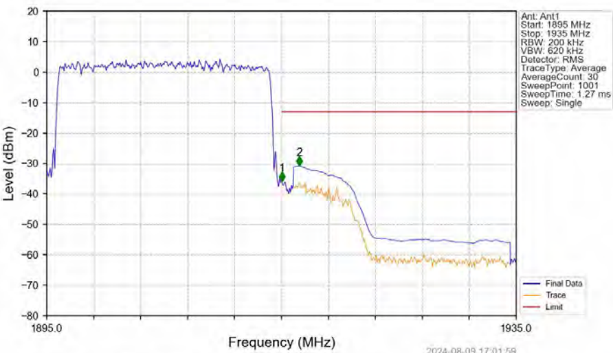
Band25_20MHz_QPSK_HCH_1905MHz_RB_100_0_NTNV
