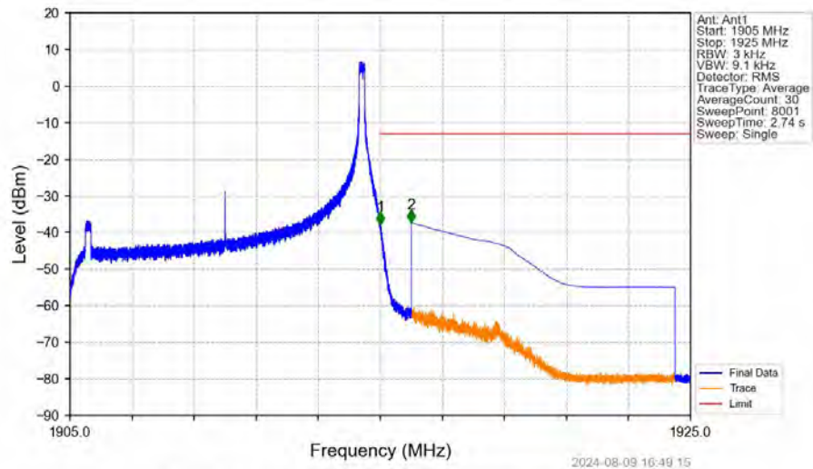
Band25_10MHz_QPSK_HCH_1910MHz_RB_1_49_NTNV
