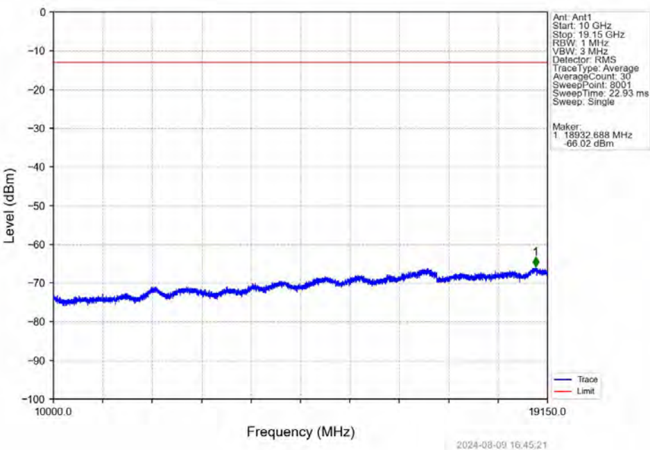
Band25_10MHz_QPSK_LCH_1855MHz_RB_50_0_NTNV
