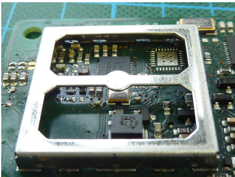
170664eut7: EUT detail view 2
