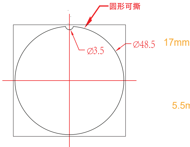
标贴尺寸图
