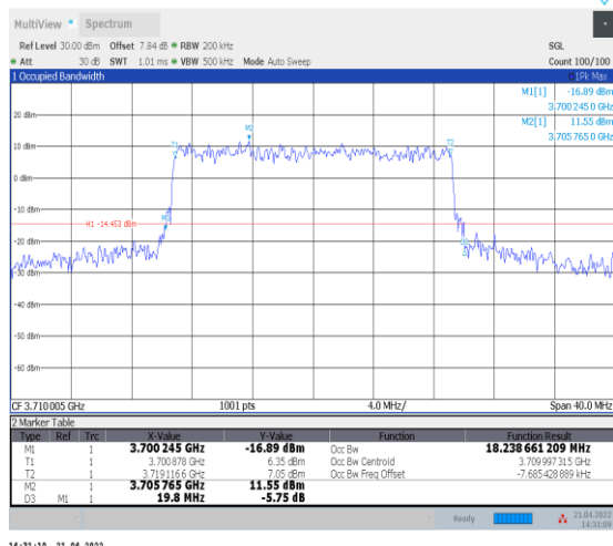
1-N77-3700-3980--30-20-L-7-CP-16QAM-Outer_Full -51@0-Ant0-18.239-19.800≤20-PASS
