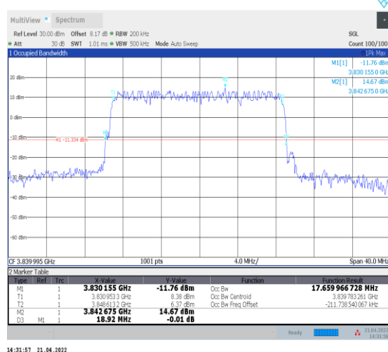
1-N77-3700-3980--30-20-M-1-DFT-QPSK-Outer_Full -50@0-Ant0-17.66-18.920-≤20-PASS
