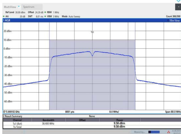
11N40MIMO_Ant3_5670
