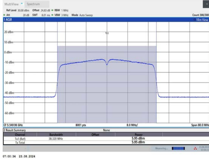
11AC40MIMO_Ant1_5550
