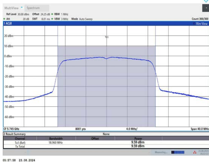
11AC20MIMO_Ant2_5745
