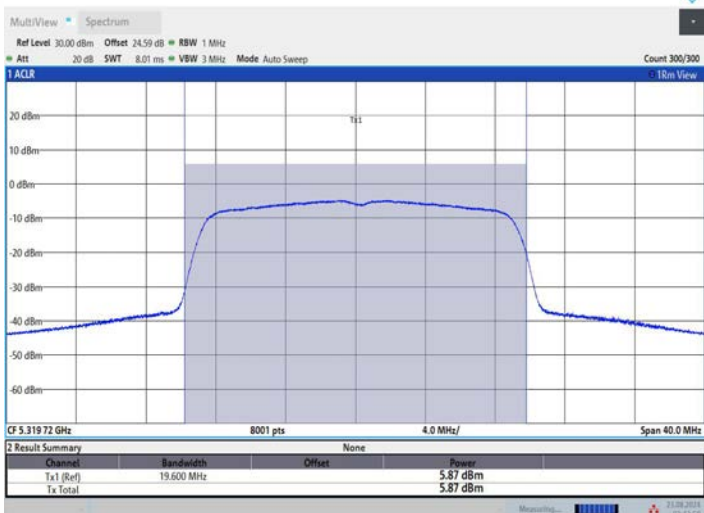
11AC20MIMO_Ant3_5320
