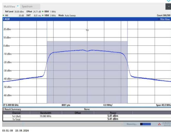
11AC20MIMO_Ant2_5500
