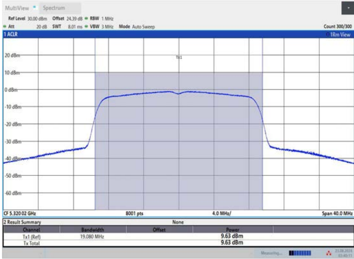
11AC20MIMO_Ant3_5320
