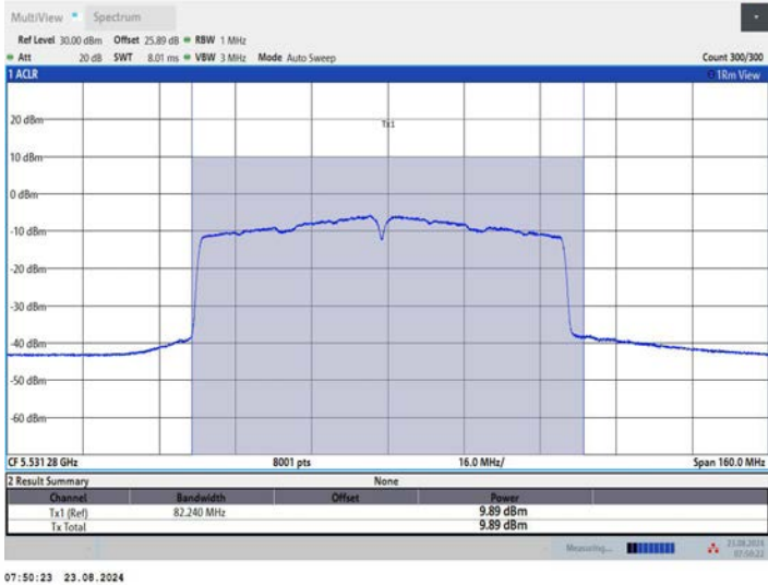
11AC80MIMO_Ant3_5530
