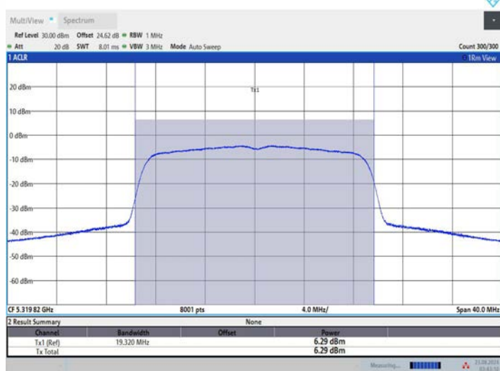
11AC20MIMO_Ant1_5320
