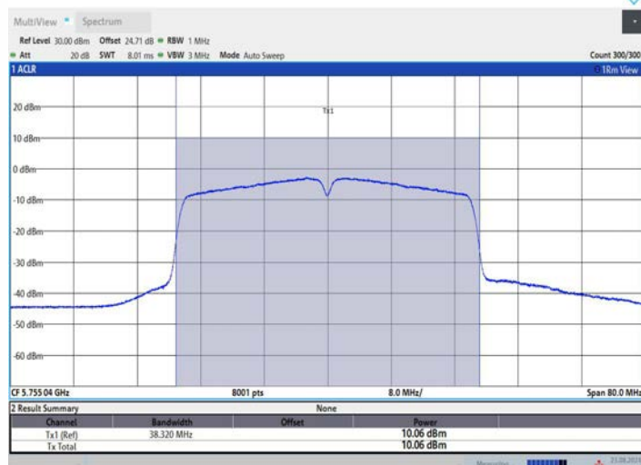
11AC40MIMO_Ant3_5755
