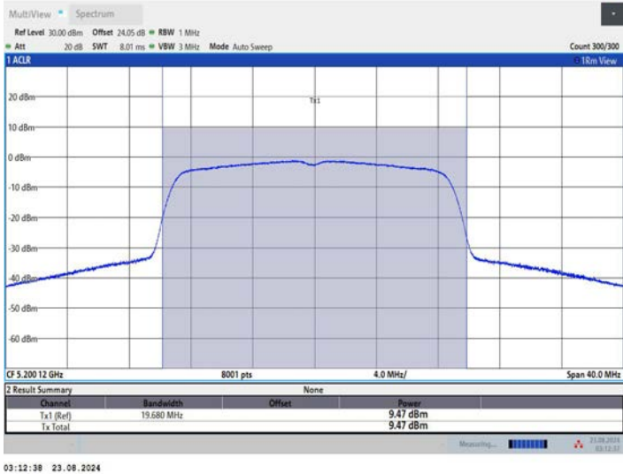
11AC20MIMO_Ant3_5200
