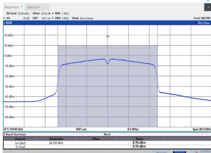
11N40MIMO_Ant3_5755
