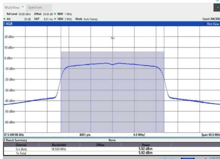
11AC20MIMO_Ant3_5500
