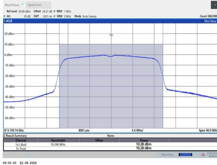
11AC20MIMO_Ant3_5745
