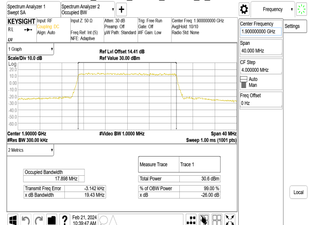
Band2_20MHz_QPSK_RB100_0_CH19100
