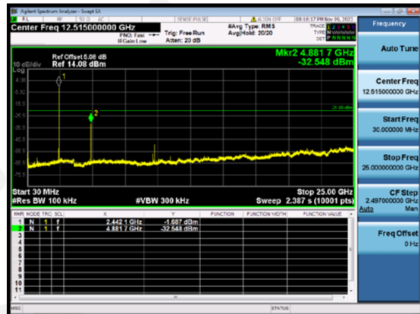
GFSK 2441MHz
