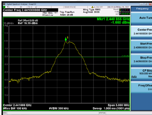
GFSK 2441MHz
