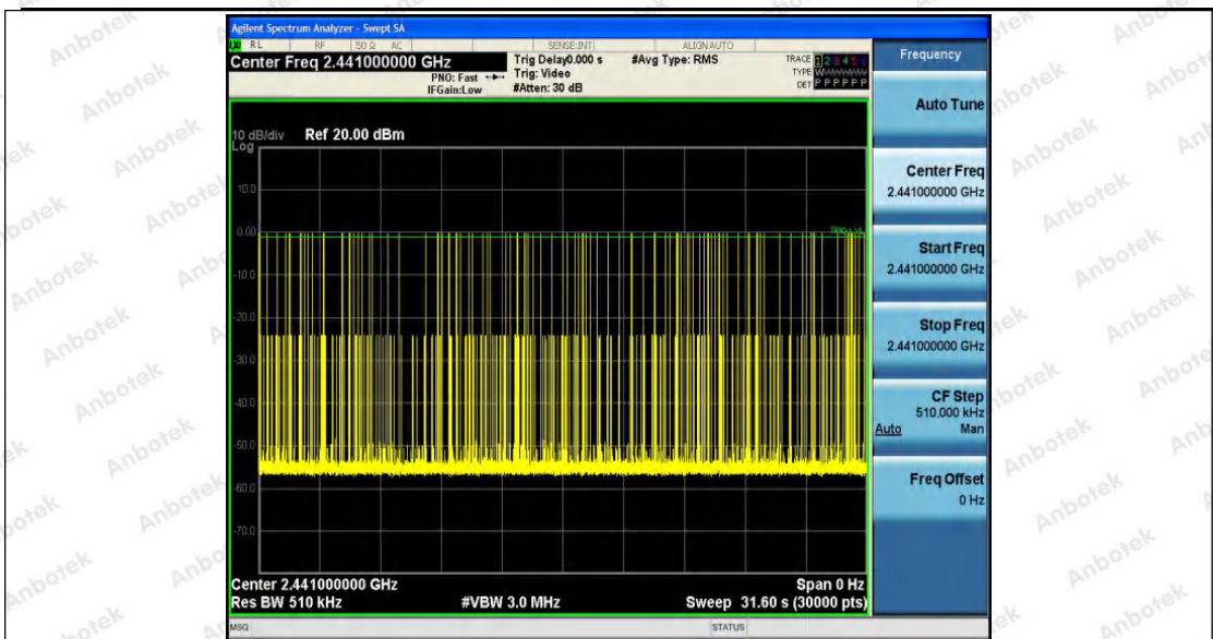
2DH1_Ant1_Hop
