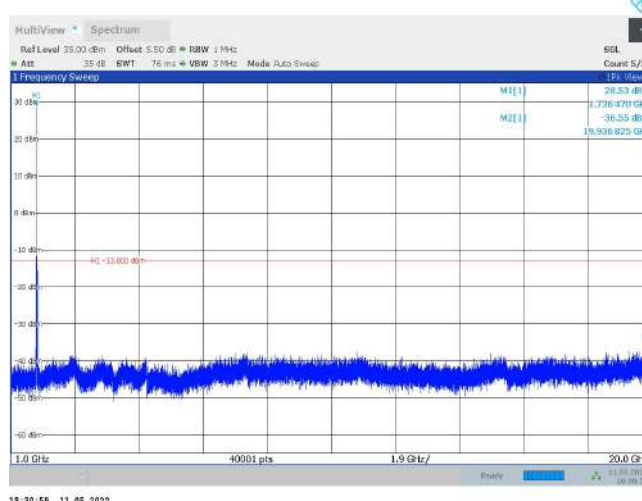
Band4-20MHz-QPSK-20300-1RB#0-Range4:1000~20000MHz
