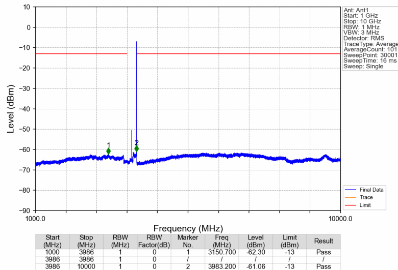
3780MHz-3980MHz_3979.9MHz_GMSK_SISO_Ant1_NTNV
