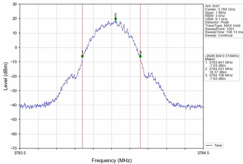
3780MHz-3980MHz_3784MHz_GMSK_SISO_Ant1_NTNV_AGC
