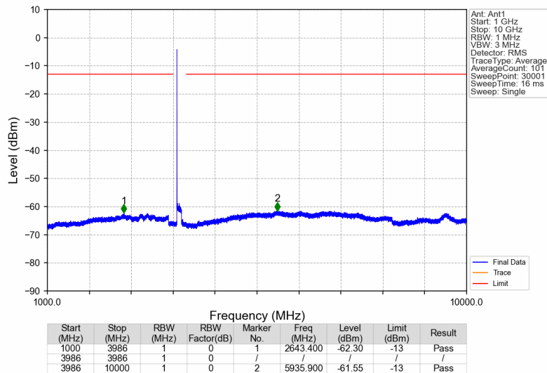
3780MHz-3980MHz_3780.1MHz_GMSK_SISO_Ant1_NTNV
