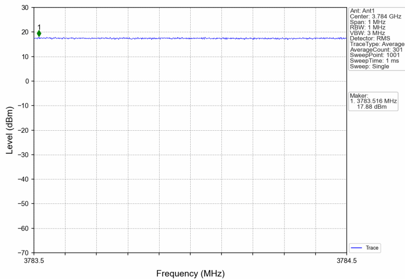
3780MHz-3980MHz_3784MHz_GMSK_SISO_Ant1_NTNV_AGC+3
