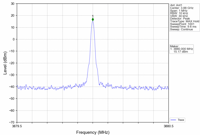
3780MHz-3980MHz_3880MHz_CW_SISO_Ant1_NTNV
