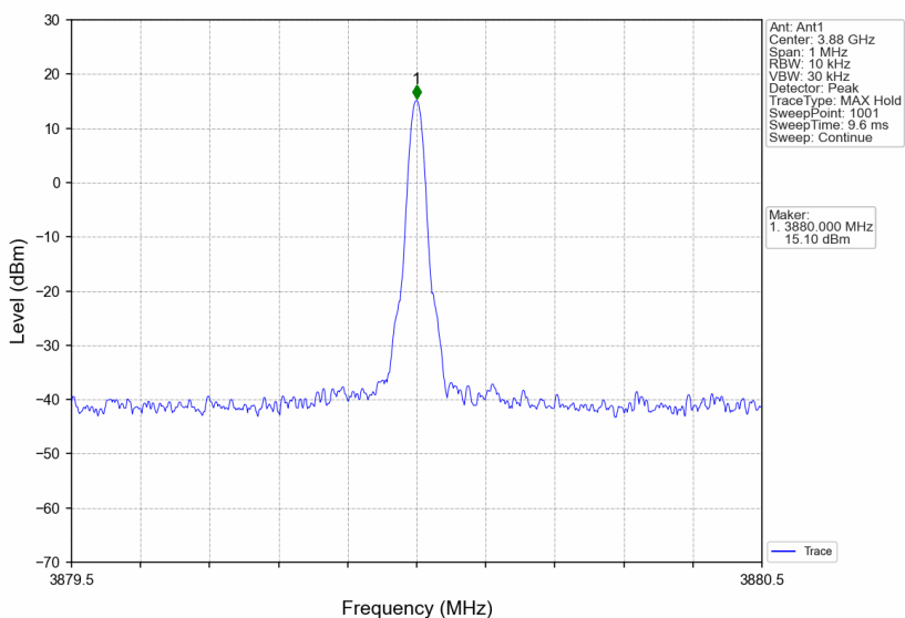
3780MHz-3980MHz_3880MHz_CW_SISO_Ant1_NTNV
