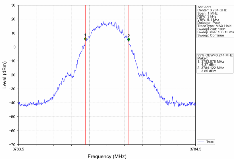
3780MHz-3980MHz_3784MHz_GMSK_SISO_Ant1_NTNV_AGC+3
