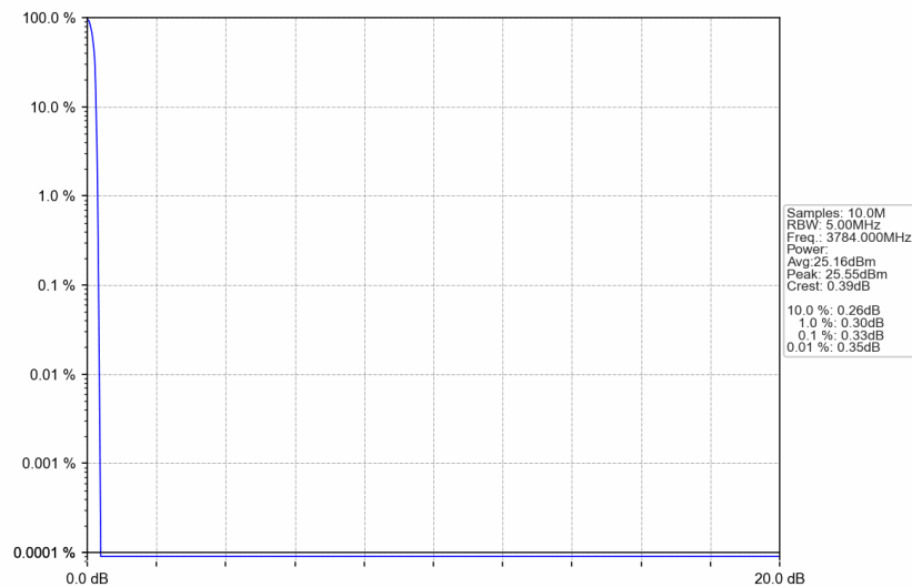
3780MHz-3980MHz_3784MHz_GMSK_SISO_Ant1_NTNV_AGC
