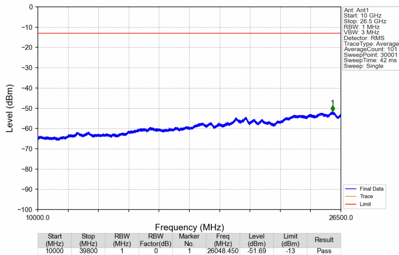
3780MHz-3980MHz_3780.1MHz_GMSK_SISO_Ant1_NTNV
