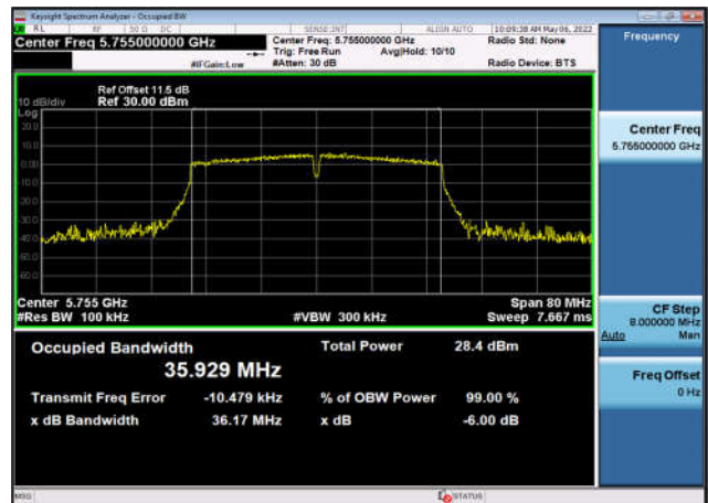
U-NII-3 6dB Bandwidth-802.11ax(40MHz) ,5755MHz,Ant0
