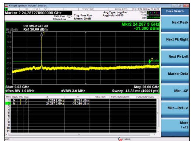
U-NII-1 ,802.11ac-VHT40, 5190MHz, Ant0
