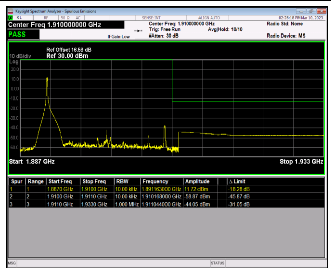
Band2-20MHz-QPSK-19100-100RB#0
