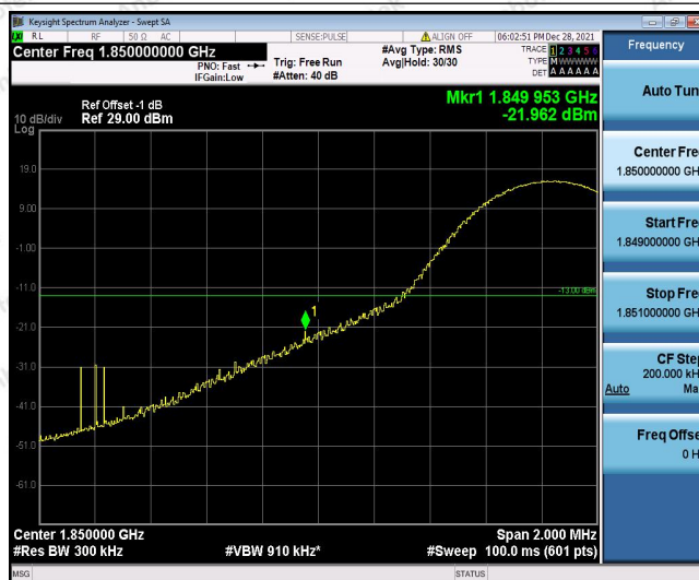
Band2-15MHz-QPSK-18675-1RB#74
