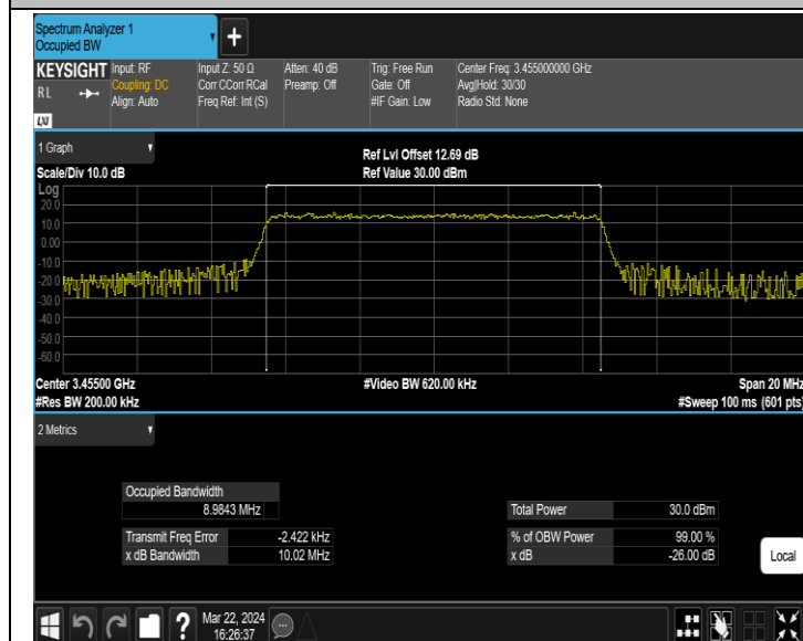
42(3450-3550)-10MHz-16QAM-42140-50RB#0-PASS
