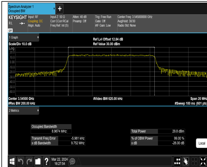
42(3450-3550)-10MHz-16QAM-43040-50RB#0-PASS
