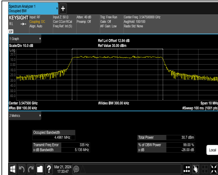
42(3450-3550)-5MHz-QPSK-43065-25RB#0-PASS
