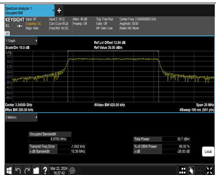
42(3450-3550)-10MHz-QPSK-43040-50RB#0-PASS
