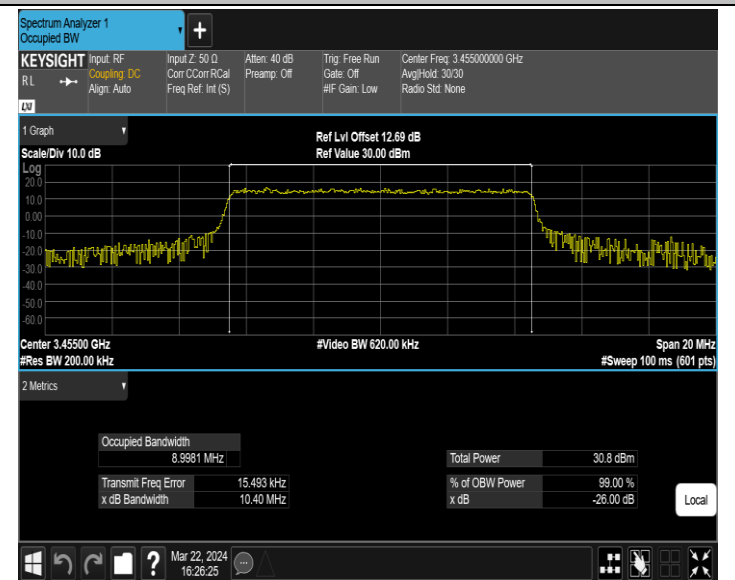
42(3450-3550)-10MHz-QPSK-42140-50RB#0-PASS
