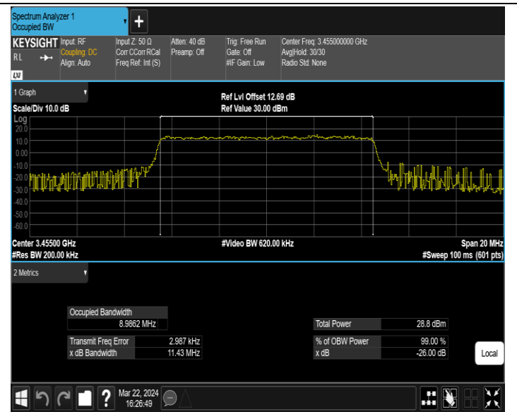
42(3450-3550)-10MHz-64QAM-42140-50RB#0-PASS
