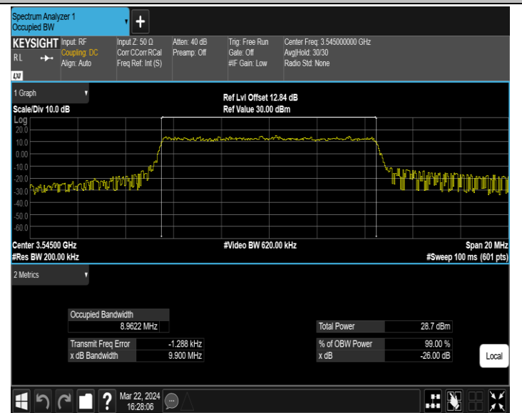
42(3450-3550)-10MHz-64QAM-43040-50RB#0-PASS
