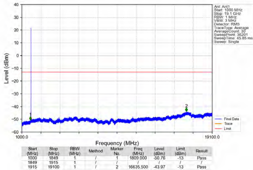
n2_15kHz_SISO_NTNV_30MHz_DFT-s-OFDM_PI/2_BPSK_1880MHz_Edge_1RB_Left
