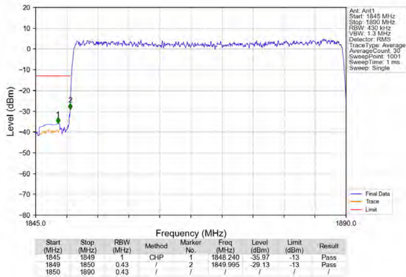
n2_15kHz_SISO_NTNV_40MHz_DFT-s-OFDM_PI/2_BPSK_1870MHz_Outer_Full
