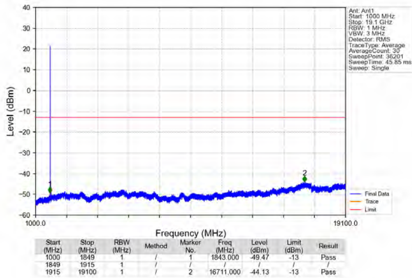
n2_15kHz_SISO_NTNV_40MHz_DFT-s-OFDM_PI/2_BPSK_1870MHz_Edge_1RB_Left
