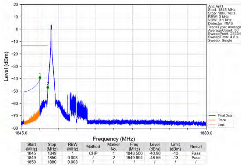
n2_15kHz_SISO_NTNV_30MHz_CP-OFDM_QPSK_1865MHz_Edge_1RB_Left
