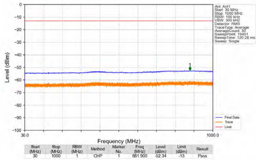
n2_15kHz_SISO_NTNV_40MHz_DFT-s-OFDM_PI/2_BPSK_1880MHz_Edge_1RB_Left
