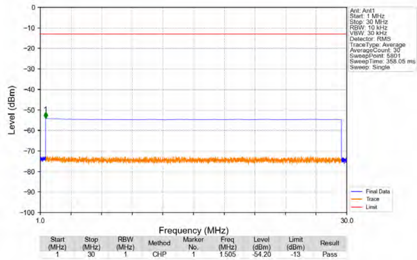
n2_15kHz_SISO_NTNV_40MHz_DFT-s-OFDM_PI/2_BPSK_1870MHz_Edge_1RB_Left
