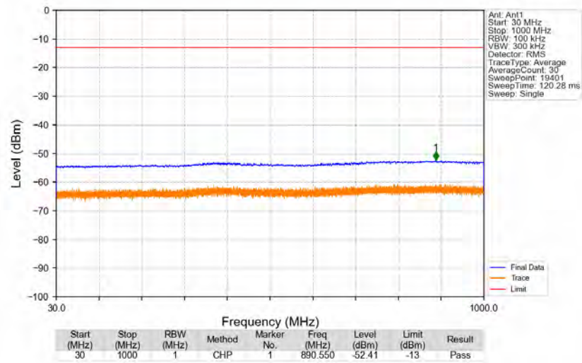
n2_15kHz_SISO_NTNV_40MHz_DFT-s-OFDM_QPSK_1870MHz_Edge_1RB_Left
