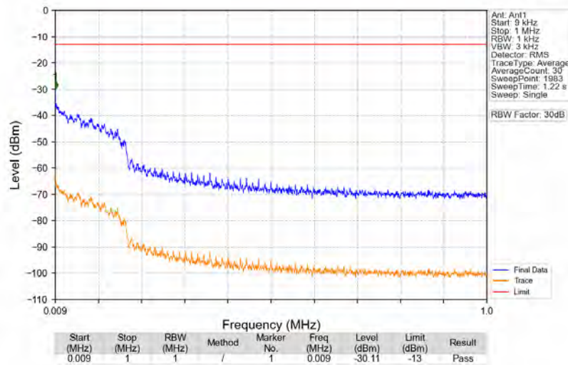
n2_15kHz_SISO_NTNV_40MHz_CP-OFDM_QPSK_1870MHz_Edge_1RB_Left
