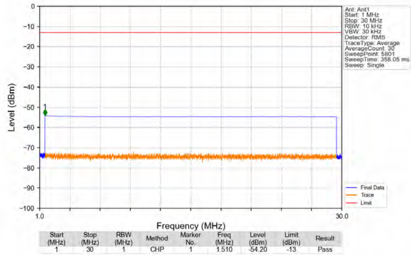
n2_15kHz_SISO_NTNV_40MHz_CP-OFDM_QPSK_1870MHz_Edge_1RB_Left
