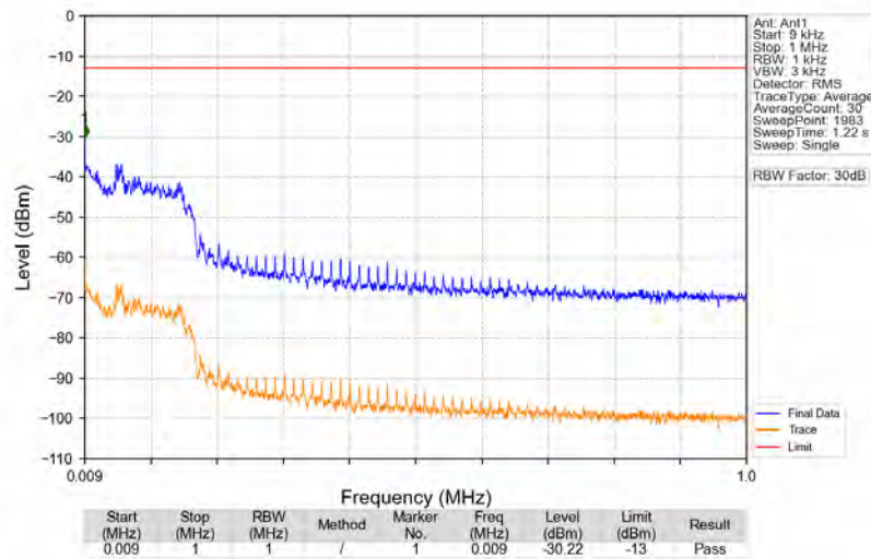
n2_15kHz_SISO_NTNV_30MHz_DFT-s-OFDM_QPSK_1865MHz_Edge_1RB_Left
