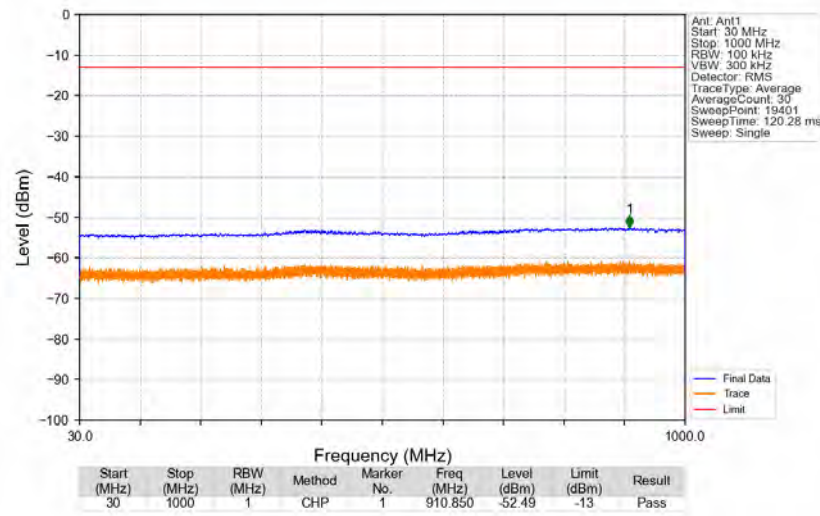
n2_15kHz_SISO_NTNV_40MHz_CP-OFDM_QPSK_1880MHz_Edge_1RB_Left
