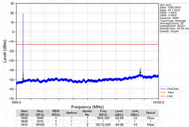
n2_15kHz_SISO_NTNV_40MHz_CP-OFDM_QPSK_1880MHz_Edge_1RB_Left
