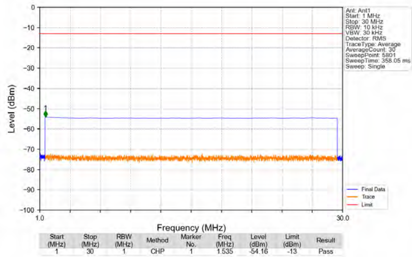
n2_15kHz_SISO_NTNV_30MHz_DFT-s-OFDM_PI/2_BPSK_1865MHz_Edge_1RB_Left
