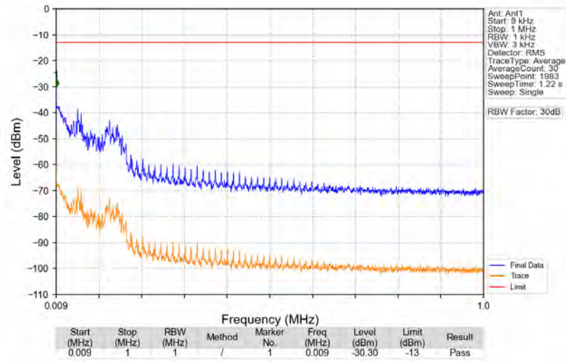
n2_15kHz_SISO_NTNV_40MHz_DFT-s-OFDM_PI/2_BPSK_1880MHz_Edge_1RB_Left
