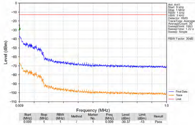
n2_15kHz_SISO_NTNV_40MHz_CP-OFDM_QPSK_1880MHz_Edge_1RB_Left
