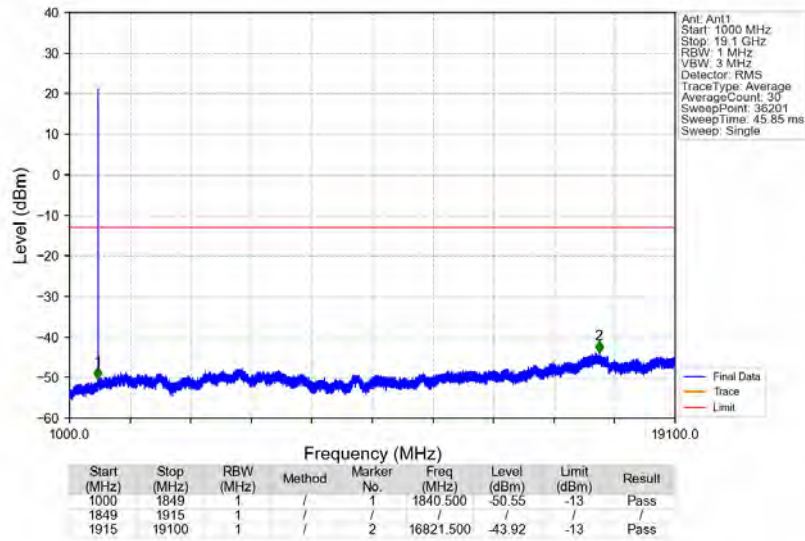
n2_15kHz_SISO_NTNV_40MHz_DFT-s-OFDM_QPSK_1870MHz_Edge_1RB_Left
