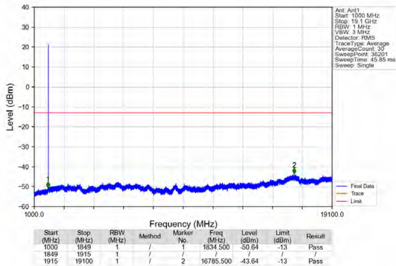
n2_15kHz_SISO_NTNV_40MHz_DFT-s-OFDM_PI/2_BPSK_1880MHz_Edge_1RB_Left
