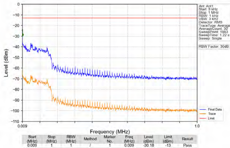
n2_15kHz_SISO_NTNV_40MHz_DFT-s-OFDM_QPSK_1870MHz_Edge_1RB_Left
