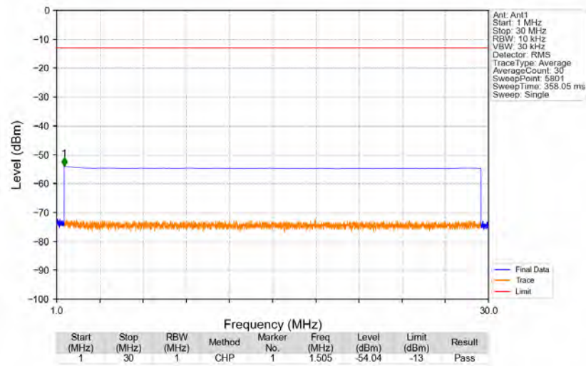
n2_15kHz_SISO_NTNV_30MHz_DFT-s-OFDM_PI/2_BPSK_1880MHz_Edge_1RB_Left
