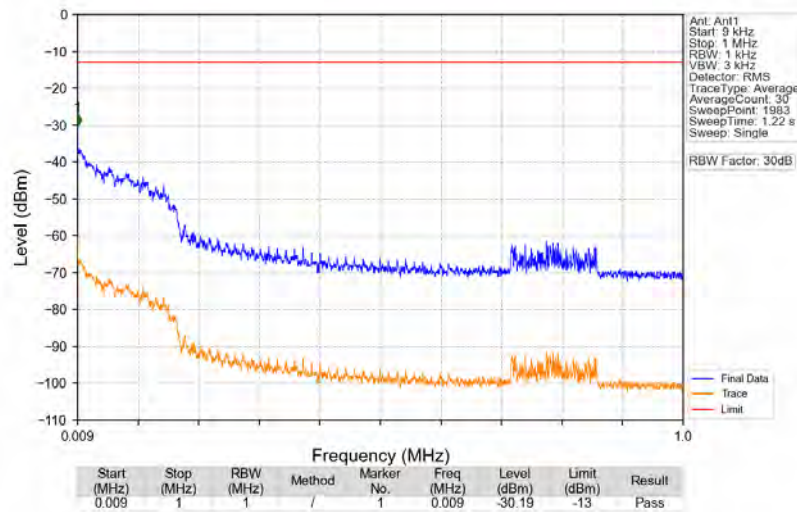
n2_15kHz_SISO_NTNV_30MHz_CP-OFDM_QPSK_1865MHz_Edge_1RB_Left
