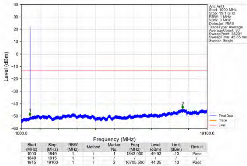
n2_15kHz_SISO_NTNV_30MHz_DFT-s-OFDM_PI/2_BPSK_1865MHz_Edge_1RB_Left
