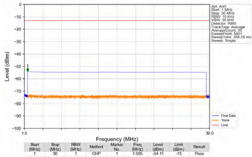
n2_15kHz_SISO_NTNV_30MHz_CP-OFDM_QPSK_1865MHz_Edge_1RB_Left
