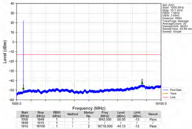
n2_15kHz_SISO_NTNV_30MHz_DFT-s-OFDM_QPSK_1865MHz_Edge_1RB_Left
