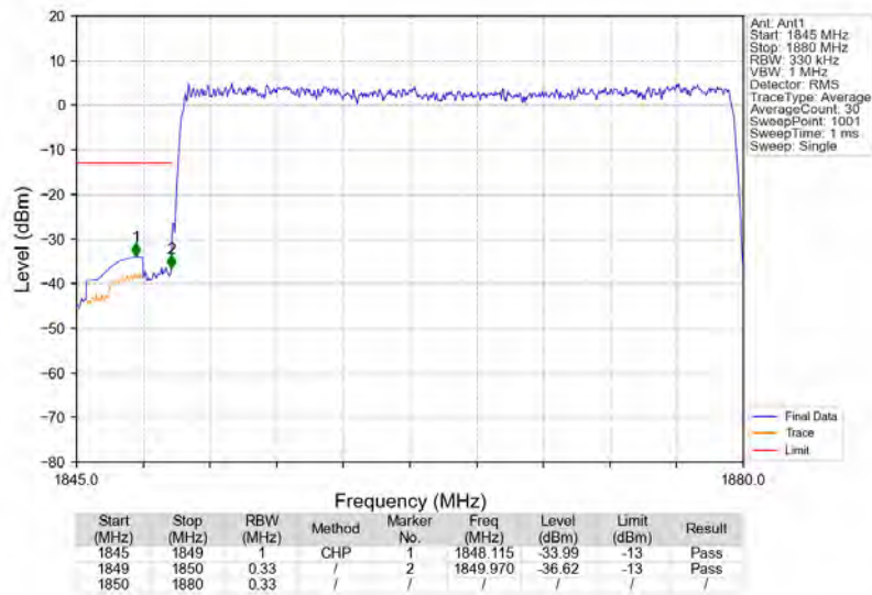
n2_15kHz_SISO_NTNV_30MHz_DFT-s-OFDM_PI/2_BPSK_1865MHz_Outer_Full
