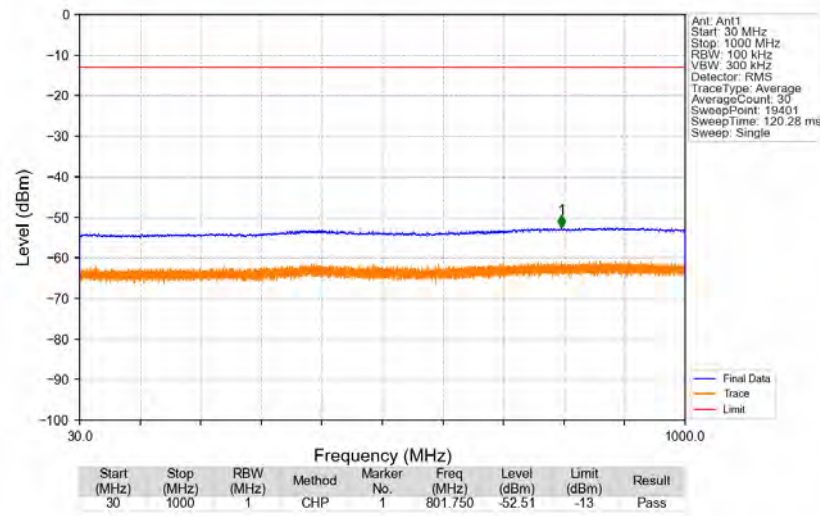
n2_15kHz_SISO_NTNV_30MHz_DFT-s-OFDM_PI/2_BPSK_1880MHz_Edge_1RB_Left
