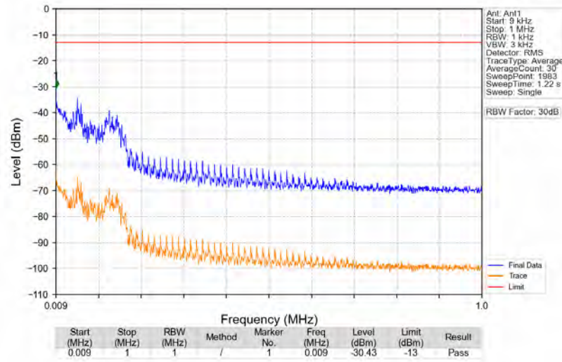
n2_15kHz_SISO_NTNV_30MHz_DFT-s-OFDM_PI/2_BPSK_1880MHz_Edge_1RB_Left
