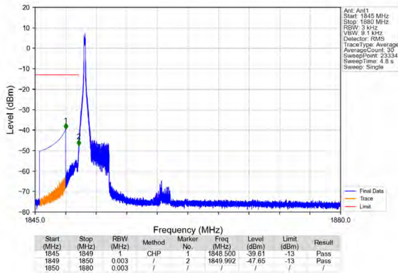
n2_15kHz_SISO_NTNV_30MHz_DFT-s-OFDM_QPSK_1865MHz_Edge_1RB_Left
