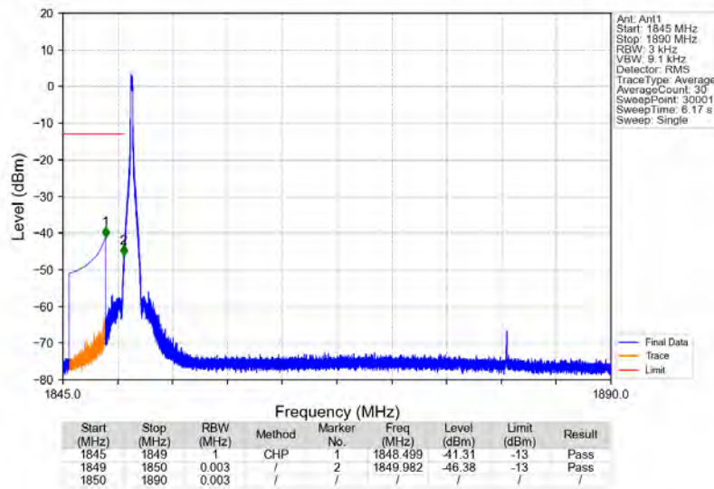
n2_15kHz_SISO_NTNV_40MHz_CP-OFDM_QPSK_1870MHz_Edge_1RB_Left
