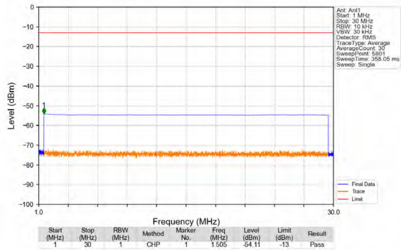
n2_15kHz_SISO_NTNV_30MHz_DFT-s-OFDM_QPSK_1865MHz_Edge_1RB_Left
