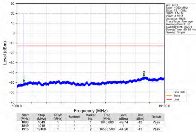
n2_15kHz_SISO_NTNV_30MHz_CP-OFDM_QPSK_1865MHz_Edge_1RB_Left
