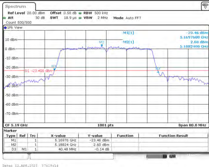
11AC40MIMO_Ant1_5190
