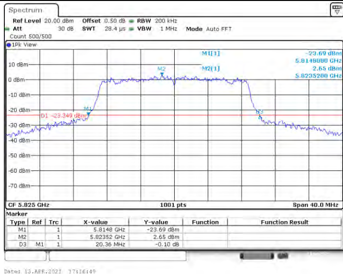
11AC20MIMO_Ant2_5825
