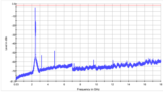
802.11n (HT20) CH1 30MHz to 18GHz
