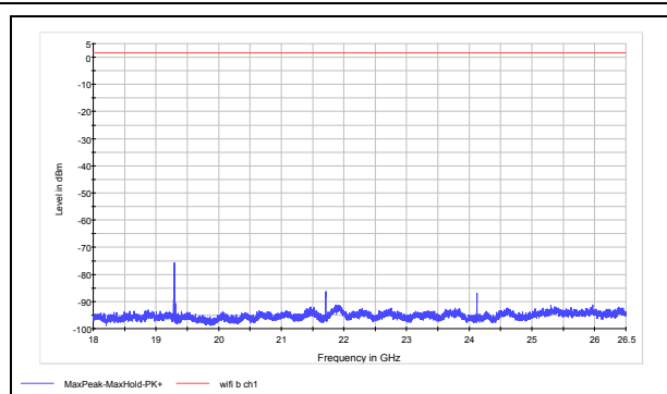
802.11b CH1 18GHz to 26.5GHz
