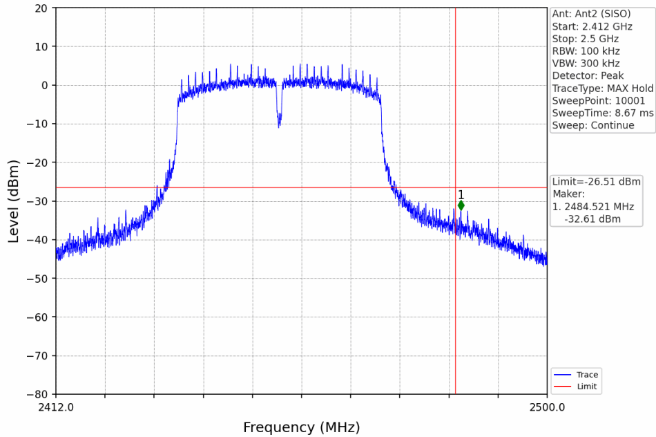
802.11n(HT40)_HCH_2452MHz_Ant2 (SISO)_NTNV
