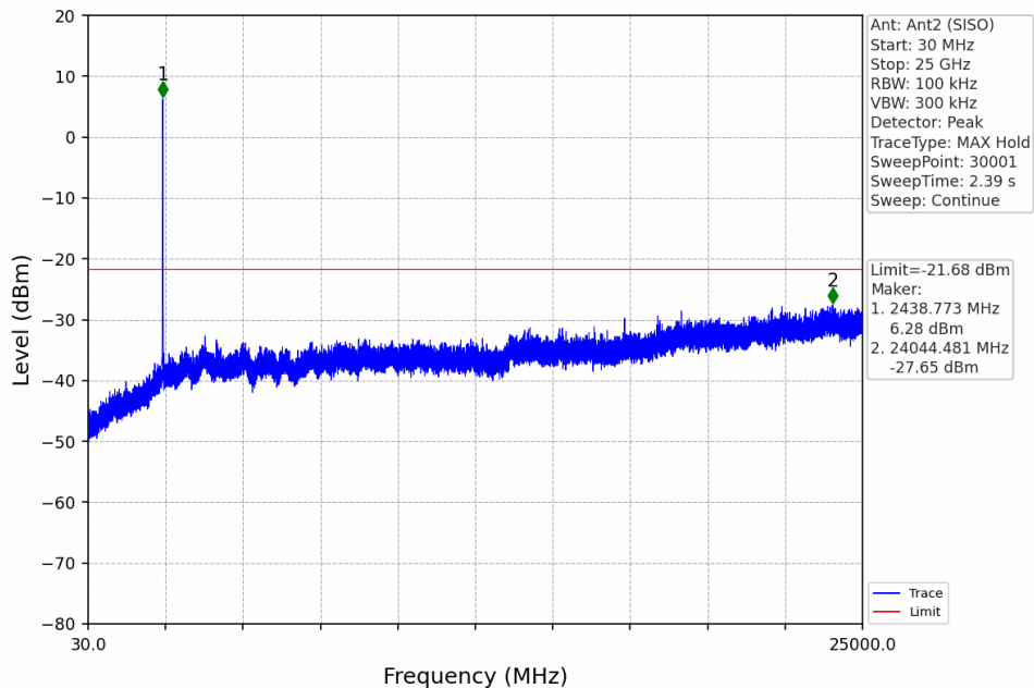
802.11n(HT20)_MCH_2437MHz_Ant2 (SISO)_NTNV
