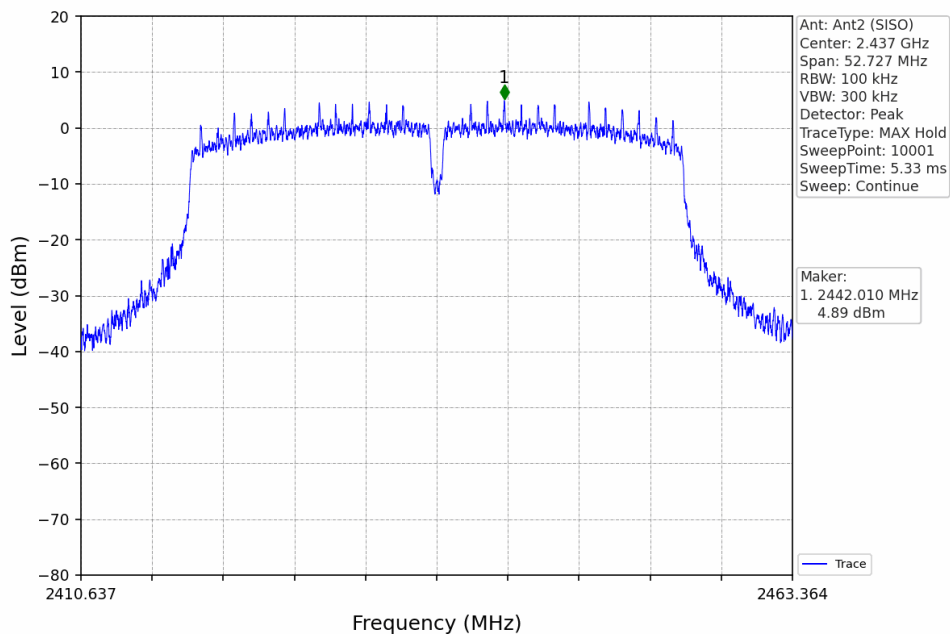
802.11n(HT40)_MCH_2437MHz_Ant2 (SISO)_NTNV
