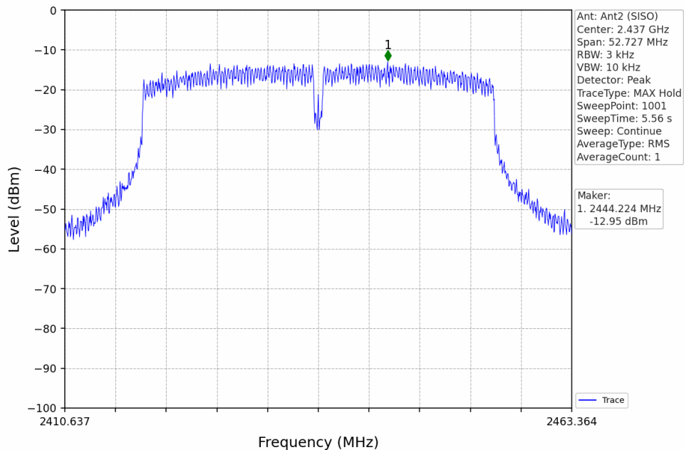
802.11n(HT40)_MCH_2437MHz_Ant2 (SISO)_NTNV
