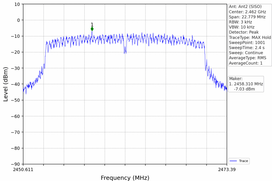
802.11n(HT20)_HCH_2462MHz_Ant2 (SISO)_NTNV
