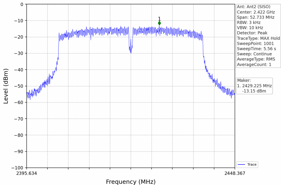
802.11n(HT40)_LCH_2422MHz_Ant2 (SISO)_NTNV
