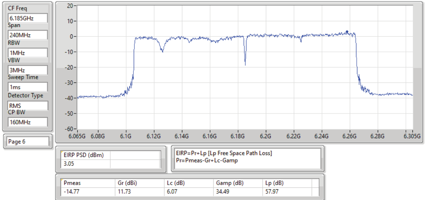
EIRP PSD;Band:6.2G;ax160,BF;BWch:160MHz;Nss:1,(M0);Nant:4;Ch:6185MHz;TX
