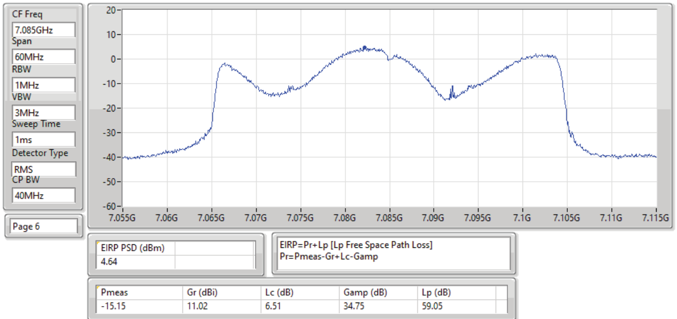
EIRP PSD;Band:7.0G;ax40;BWch:40MHz;Nss:1,(M0);Nant:4;Ch:7085MHz;TX
