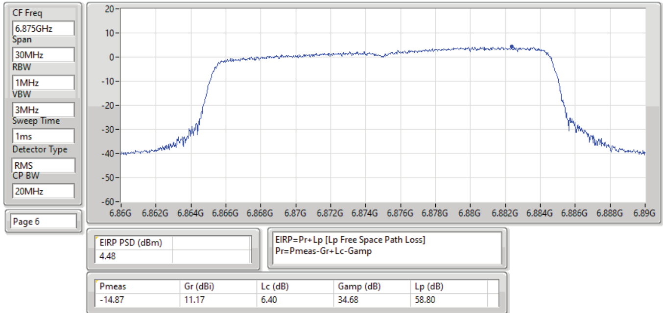
EIRP PSD;Band:6.7G;ax20,BF;BWch:20MHz;Nss:1,(M0);Nant:4;Ch:6875MHz;TX
