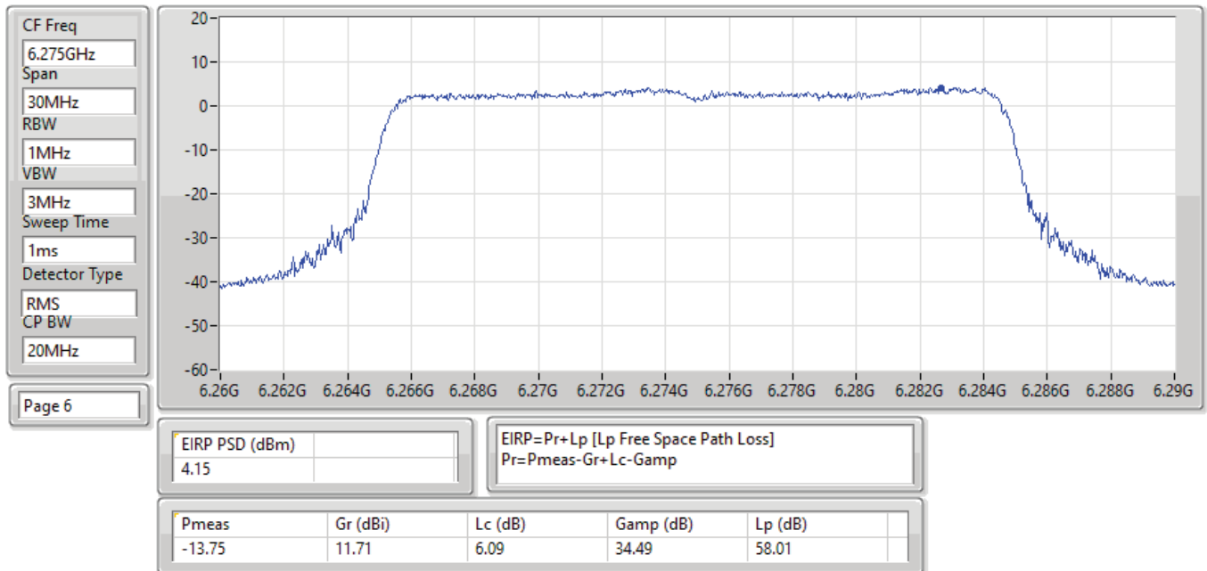
EIRP PSD;Band:6.2G;ax20,BF;BWch:20MHz;Nss:1,(M0);Nant:4;Ch:6275MHz;TX
