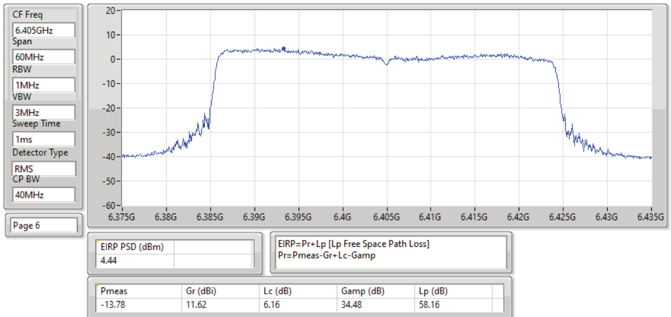
EIRP PSD;Band:6.2G;ax40,BF;BWch:40MHz;Nss:1,(M0);Nant:4;Ch:6405MHz;TX
