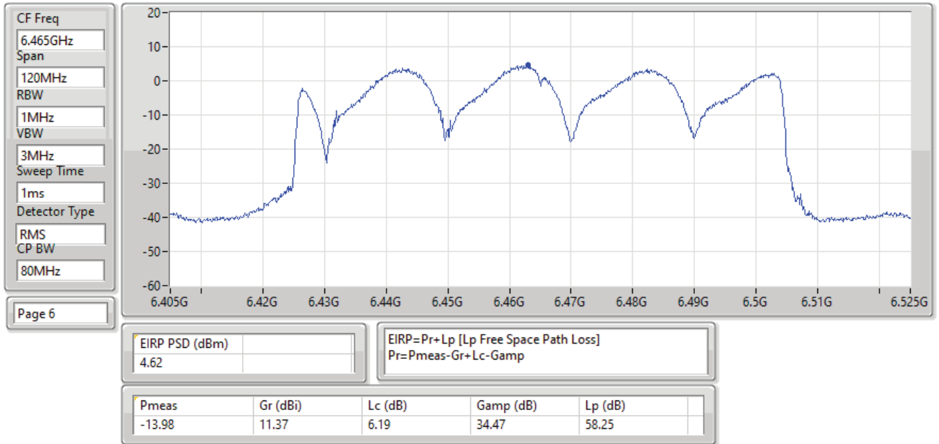
EIRP PSD;Band:6.4G;ax80;BWch:80MHz;Nss:1,(M0);Nant:4;Ch:6465MHz;TX
