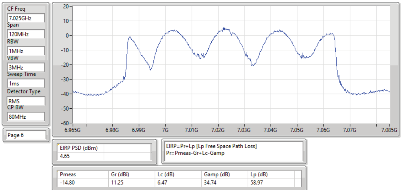
EIRP PSD;Band:7.0G;ax80;BWch:80MHz;Nss:1,(M0);Nant:4;Ch:7025MHz;TX
