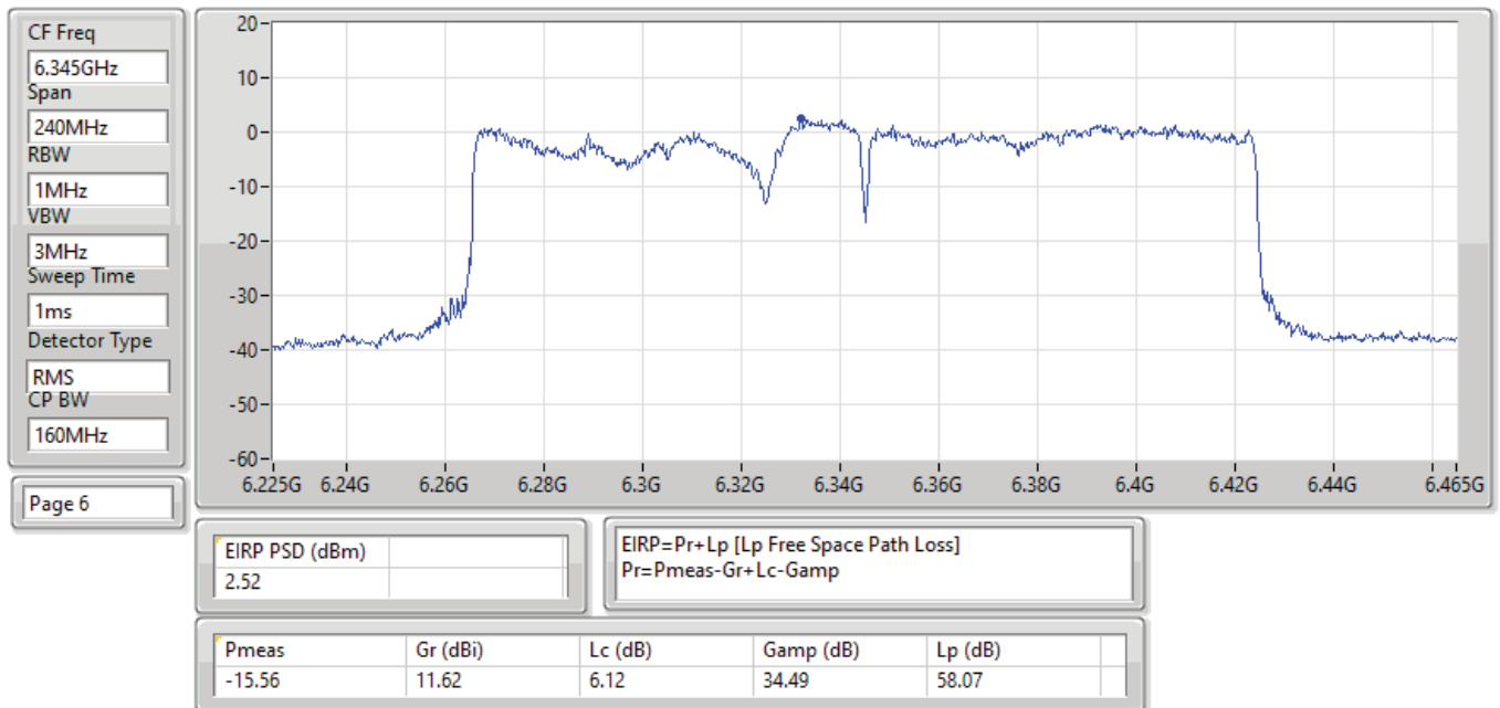
EIRP PSD;Band:6.2G;ax160,BF;BWch:160MHz;Nss:1,(M0);Nant:4;Ch:6345MHz;TX
