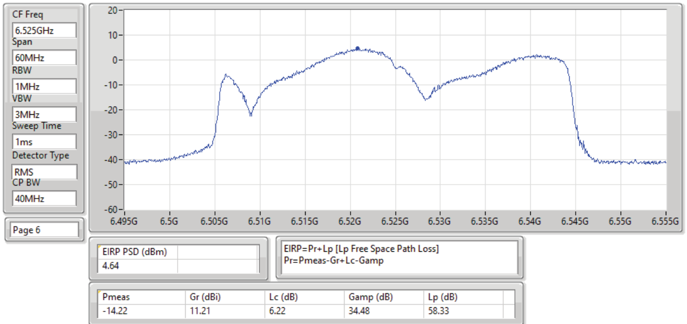
EIRP PSD;Band:6.4G;ax40;BWch:40MHz;Nss:1,(M0);Nant:4;Ch:6525MHz;TX
