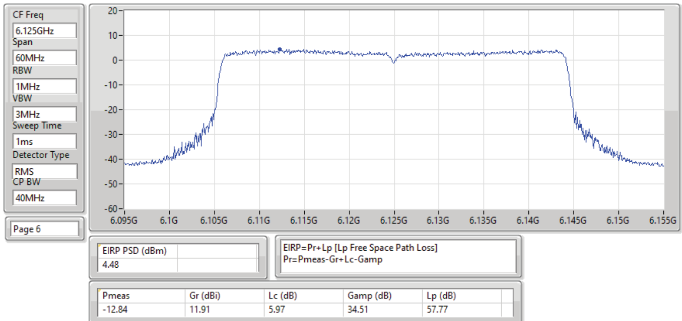
EIRP PSD;Band:6.2G;ax40,BF;BWch:40MHz;Nss:1,(M0);Nant:4;Ch:6125MHz;TX
