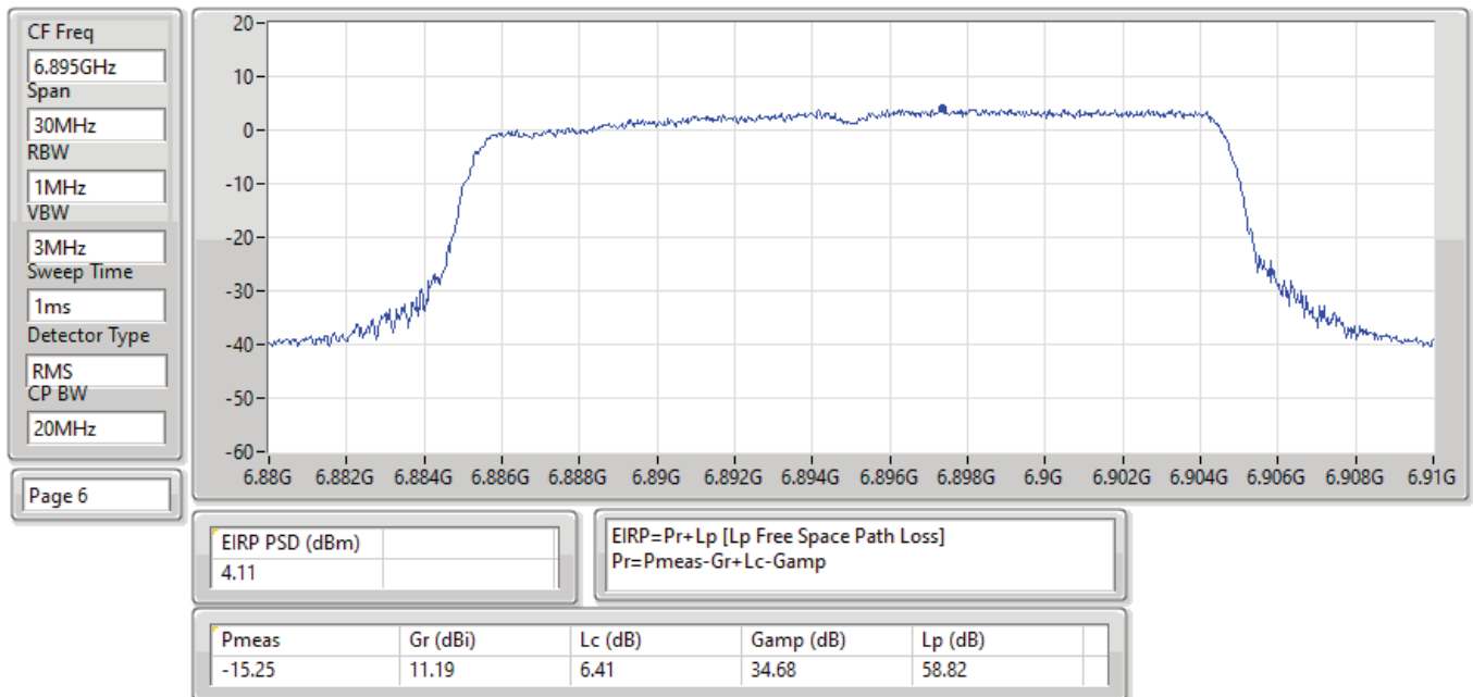
EIRP PSD;Band:7.0G;ax20,BF;BWch:20MHz;Nss:1,(M0);Nant:4;Ch:6895MHz;TX
