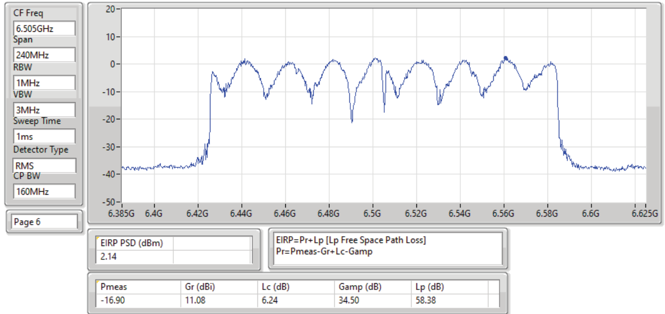
EIRP PSD;Band:6.4G;ax160,BF;BWch:160MHz;Nss:1,(M0);Nant:4;Ch:6505MHz;TX
