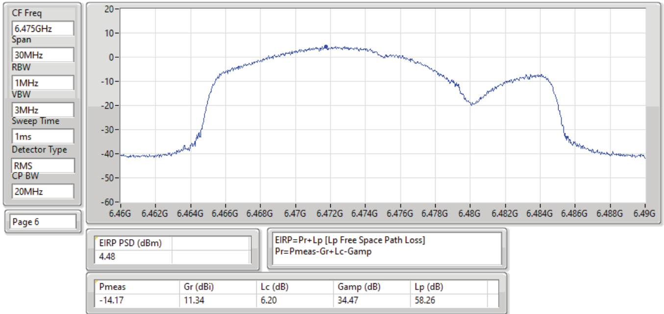
EIRP PSD;Band:6.4G;ax20;BWch:20MHz;Nss:1,(M0);Nant:4;Ch:6475MHz;TX
