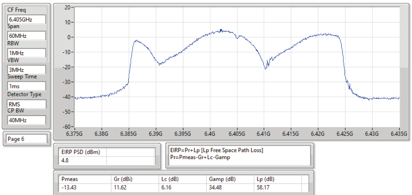
EIRP PSD;Band:6.2G;ax40;BWch:40MHz;Nss:1,(M0);Nant:4;Ch:6405MHz;TX
