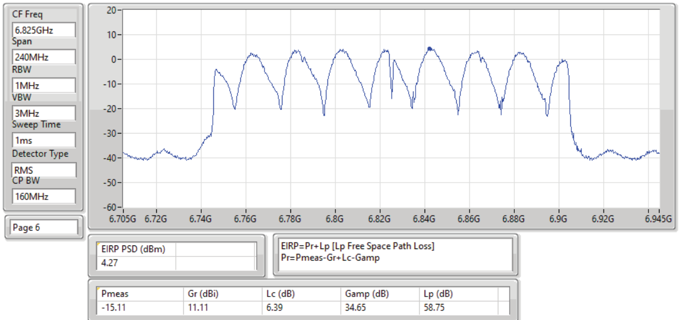
EIRP PSD;Band:6.7G;ax160;BWch:160MHz;Nss:1,(M0);Nant:4;Ch:6825MHz;TX
