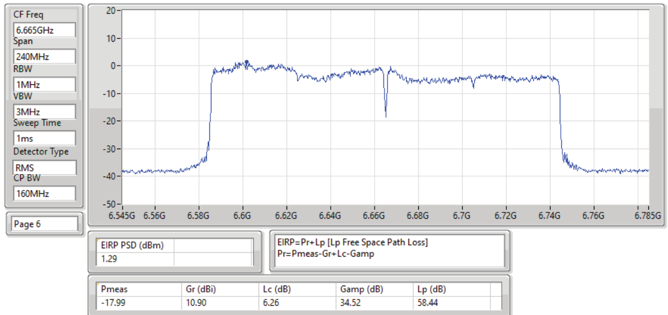
EIRP PSD;Band:6.7G;ax160,BF;BWch:160MHz;Nss:1,(M0);Nant:4;Ch:6665MHz;TX
