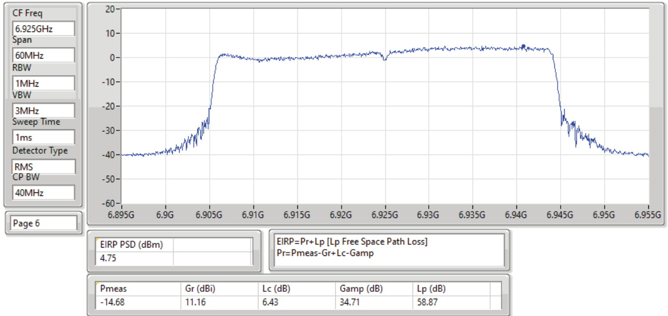
EIRP PSD;Band:7.0G;ax40,BF;BWch:40MHz;Nss:1,(M0);Nant:4;Ch:6925MHz;TX
