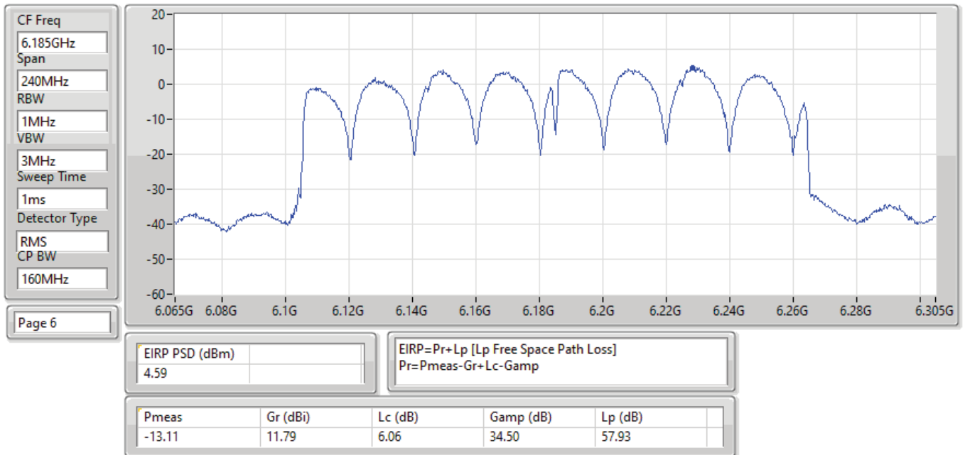
EIRP PSD;Band:6.2G;ax160;BWch:160MHz;Nss:1,(M0);Nant:4;Ch:6185MHz;TX
