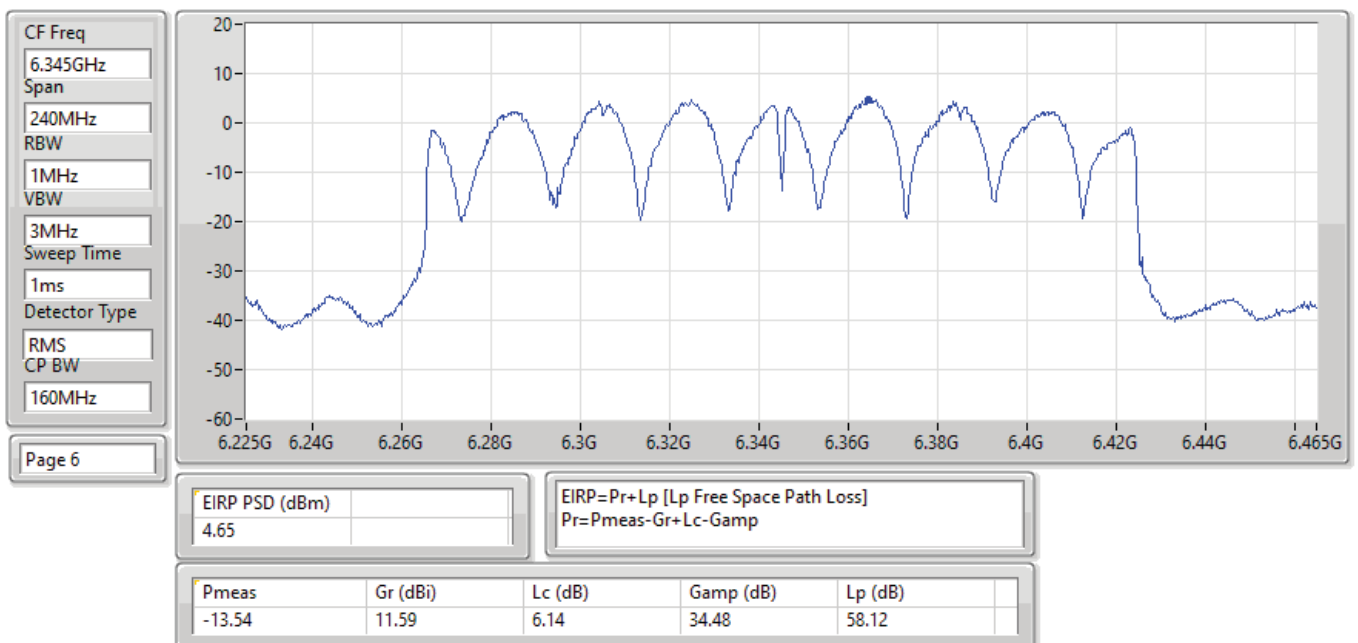
EIRP PSD;Band:6.2G;ax160;BWch:160MHz;Nss:1,(M0);Nant:4;Ch:6345MHz;TX
