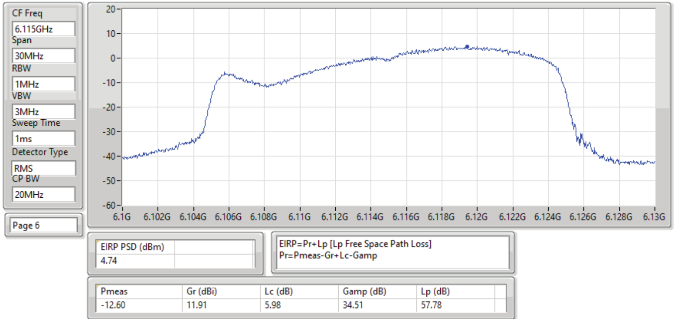
EIRP PSD;Band:6.2G;ax20;BWch:20MHz;Nss:1,(M0);Nant:4;Ch:6115MHz;TX
