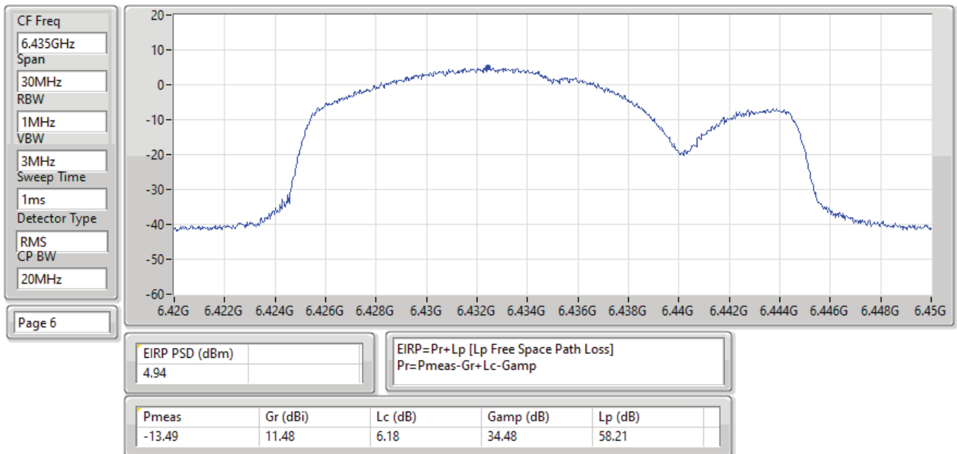
EIRP PSD;Band:6.4G;ax20;BWch:20MHz;Nss:1,(M0);Nant:4;Ch:6435MHz;TX
