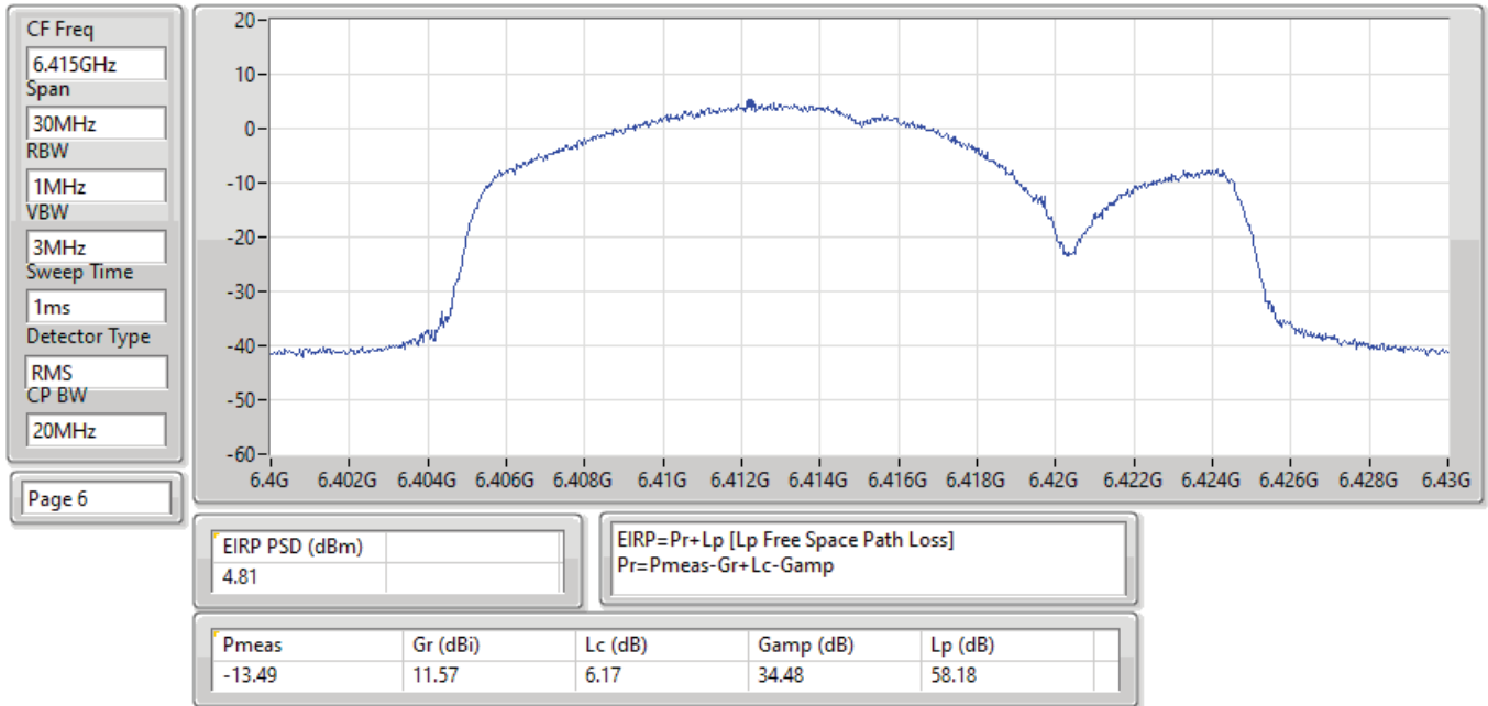
EIRP PSD;Band:6.2G;ax20;BWch:20MHz;Nss:1,(M0);Nant:4;Ch:6415MHz;TX
