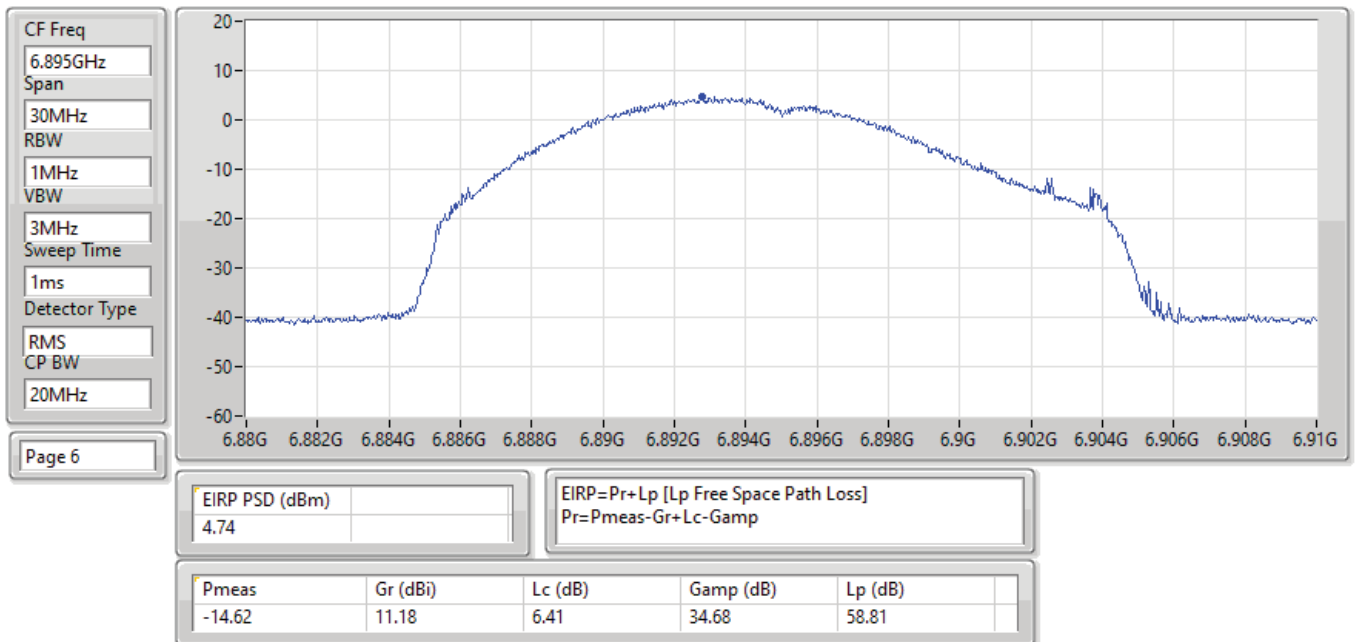
EIRP PSD;Band:7.0G;ax20;BWch:20MHz;Nss:1,(M0);Nant:4;Ch:6895MHz;TX
