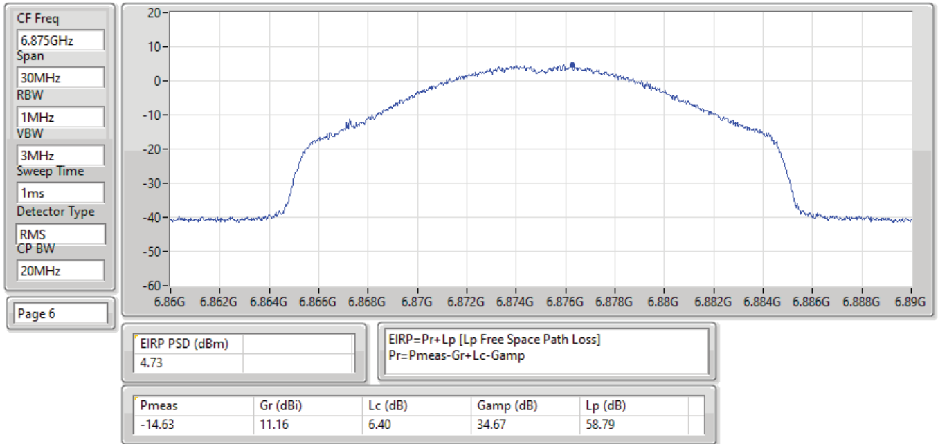
EIRP PSD;Band:6.7G;ax20;BWch:20MHz;Nss:1,(M0);Nant:4;Ch:6875MHz;TX
