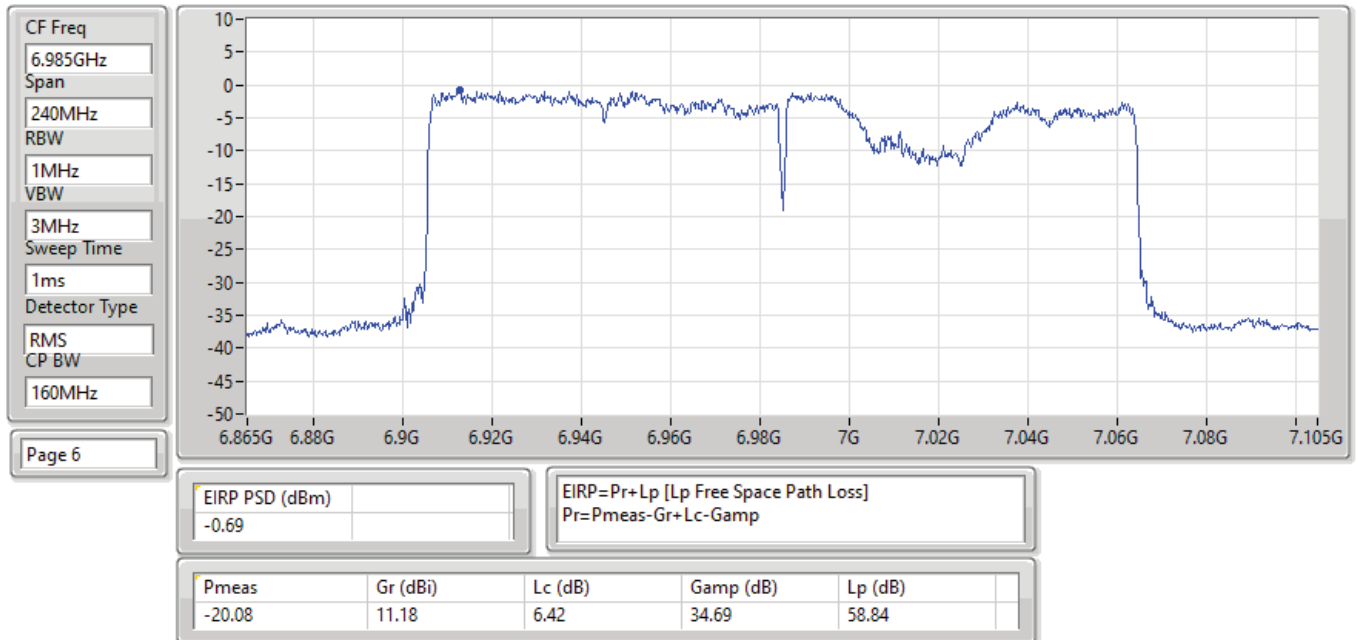
EIRP PSD;Band:7.0G;ax160,BF;BWch:160MHz;Nss:1,(M0);Nant:4;Ch:6985MHz;TX
