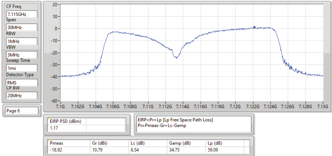
EIRP PSD;Band:7.0G;ax20,BF;BWch:20MHz;Nss:1,(M0);Nant:4;Ch:7115MHz;TX
