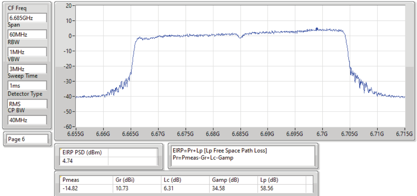
EIRP PSD;Band:6.7G;ax40,BF;BWch:40MHz;Nss:1,(M0);Nant:4;Ch:6685MHz;TX
