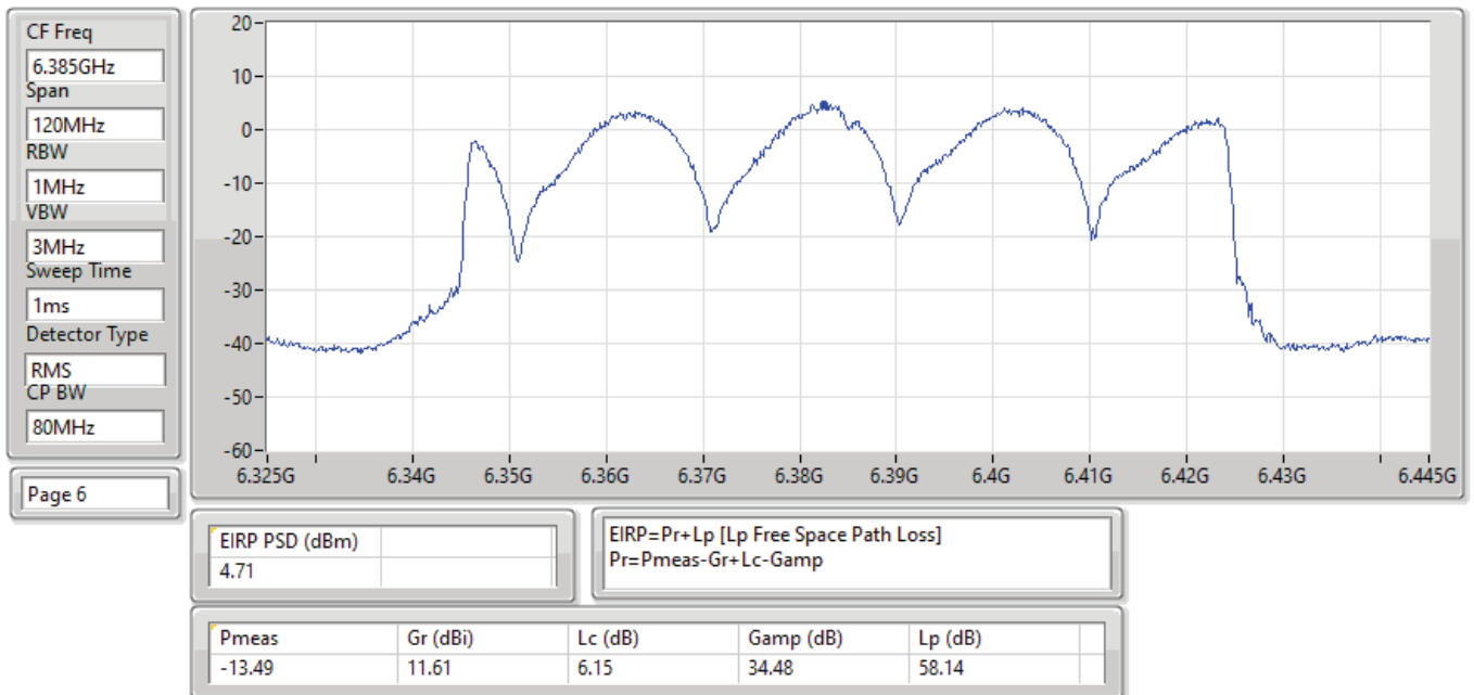
EIRP PSD;Band:6.2G;ax80;BWch:80MHz;Nss:1,(M0);Nant:4;Ch:6385MHz;TX
