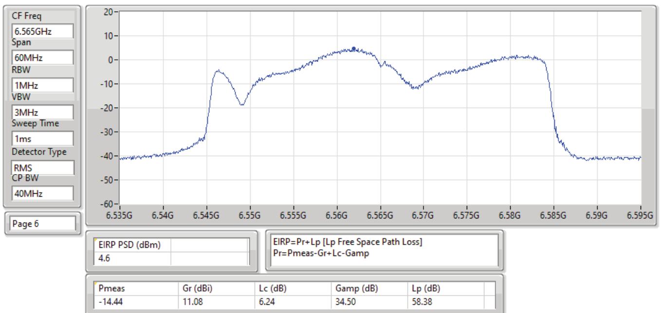
EIRP PSD;Band:6.7G;ax40;BWch:40MHz;Nss:1,(M0);Nant:4;Ch:6565MHz;TX
