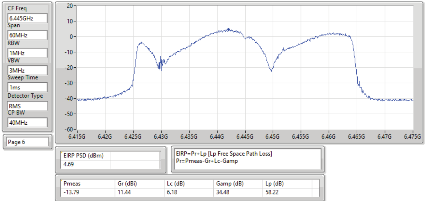
EIRP PSD;Band:6.4G;ax40;BWch:40MHz;Nss:1,(M0);Nant:4;Ch:6445MHz;TX
