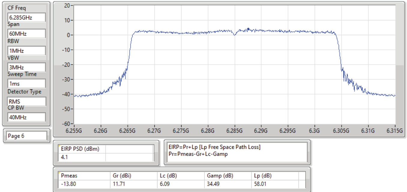
EIRP PSD;Band:6.2G;ax40,BF;BWch:40MHz;Nss:1,(M0);Nant:4;Ch:6285MHz;TX
