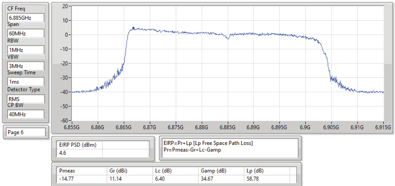
EIRP PSD;Band:6.7G;ax40,BF;BWch:40MHz;Nss:1,(M0);Nant:4;Ch:6885MHz;TX
