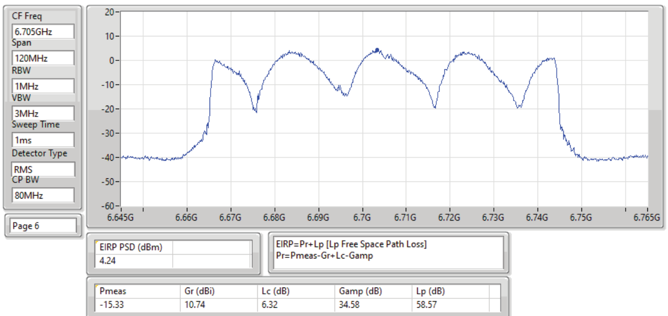
EIRP PSD;Band:6.7G;ax80;BWch:80MHz;Nss:1,(M0);Nant:4;Ch:6705MHz;TX
