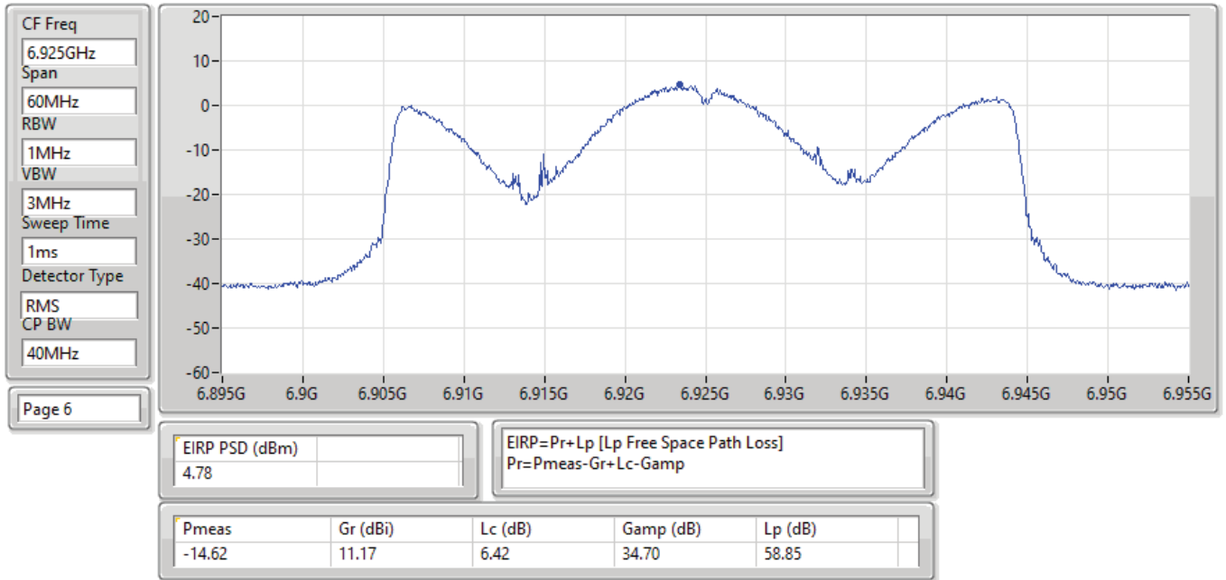
EIRP PSD;Band:7.0G;ax40;BWch:40MHz;Nss:1,(M0);Nant:4;Ch:6925MHz;TX
