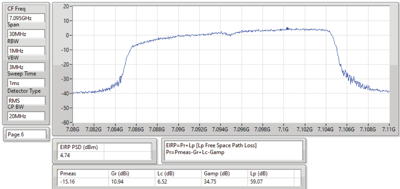
EIRP PSD;Band:7.0G;ax20,BF;BWch:20MHz;Nss:1,(M0);Nant:4;Ch:7095MHz;TX
