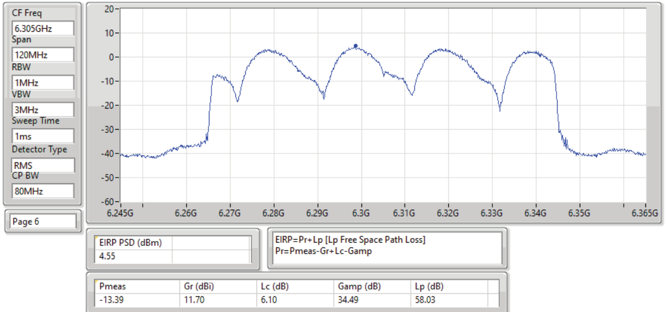
EIRP PSD;Band:6.2G;ax80;BWch:80MHz;Nss:1,(M0);Nant:4;Ch:6305MHz;TX
