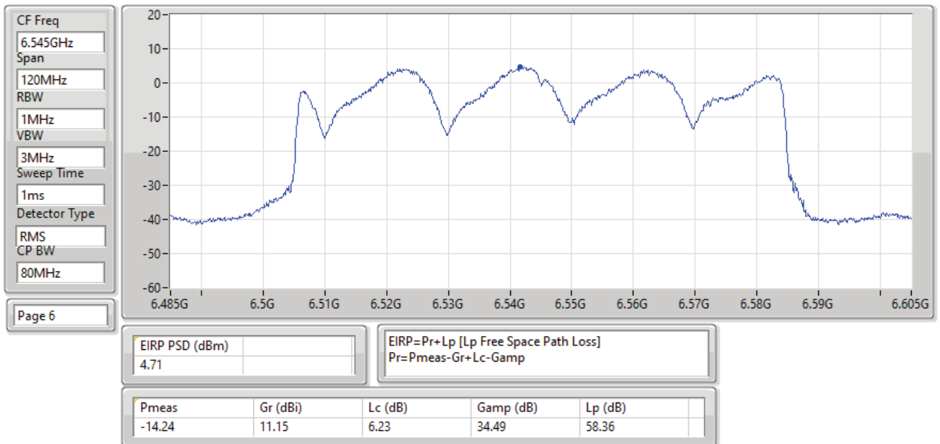
EIRP PSD;Band:6.4G;ax80;BWch:80MHz;Nss:1,(M0);Nant:4;Ch:6545MHz;TX
