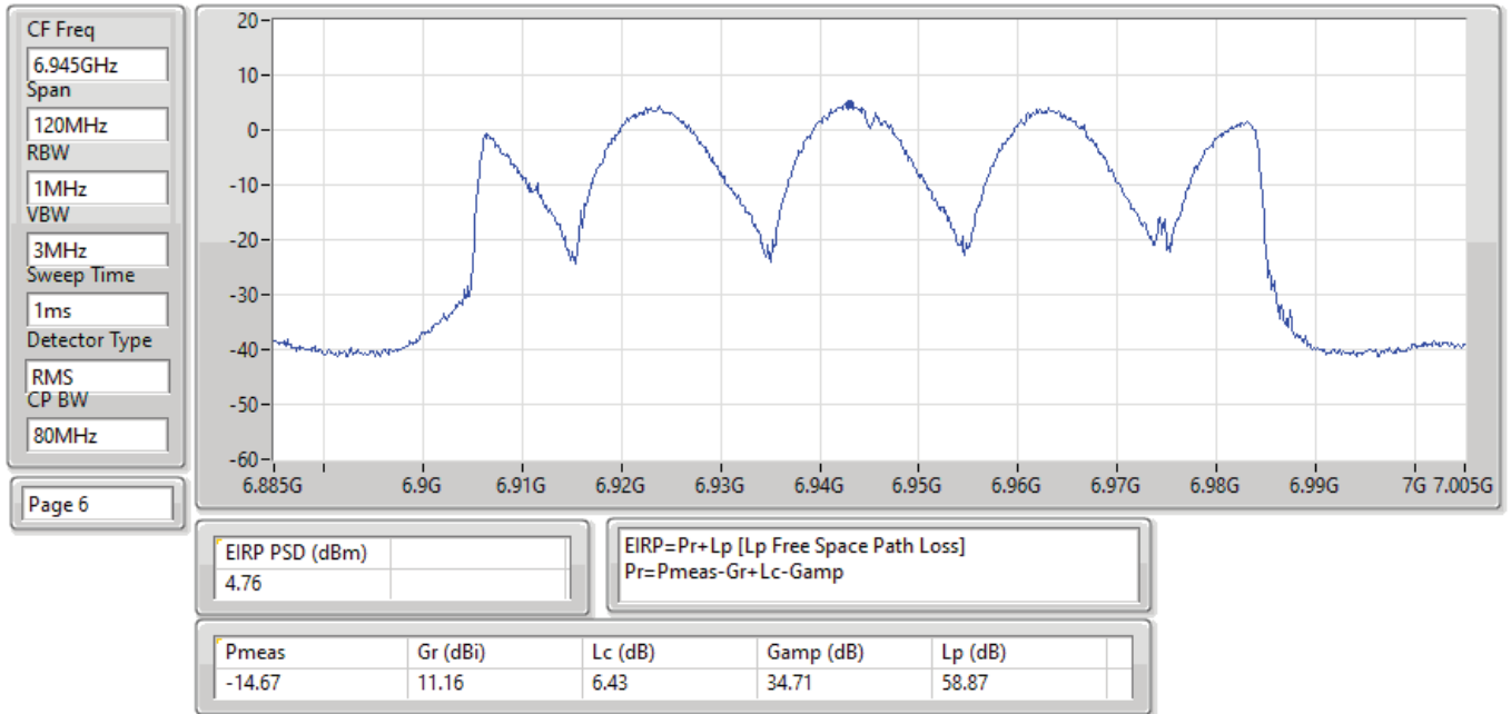
EIRP PSD;Band:7.0G;ax80;BWch:80MHz;Nss:1,(M0);Nant:4;Ch:6945MHz;TX
