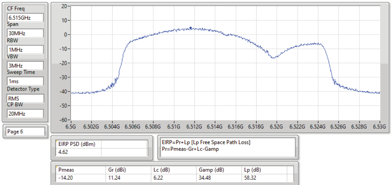
EIRP PSD;Band:6.4G;ax20;BWch:20MHz;Nss:1,(M0);Nant:4;Ch:6515MHz;TX
