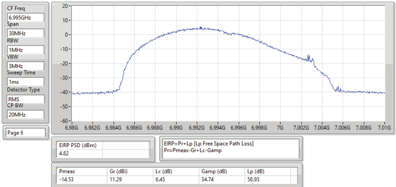
EIRP PSD;Band:7.0G;ax20;BWch:20MHz;Nss:1,(M0);Nant:4;Ch:6995MHz;TX
