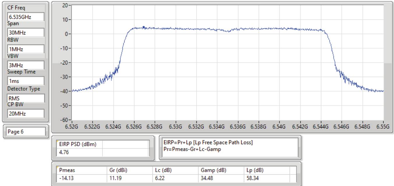
EIRP PSD;Band:6.7G;ax20,BF;BWch:20MHz;Nss:1,(M0);Nant:4;Ch:6535MHz;TX
