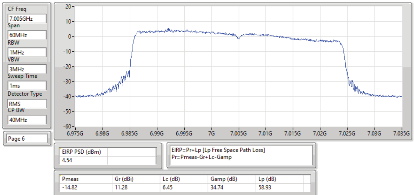
EIRP PSD;Band:7.0G;ax40,BF;BWch:40MHz;Nss:1,(M0);Nant:4;Ch:7005MHz;TX
