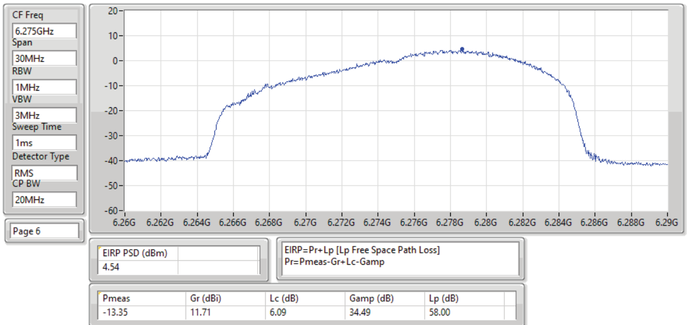
EIRP PSD;Band:6.2G;ax20;BWch:20MHz;Nss:1,(M0);Nant:4;Ch:6275MHz;TX
