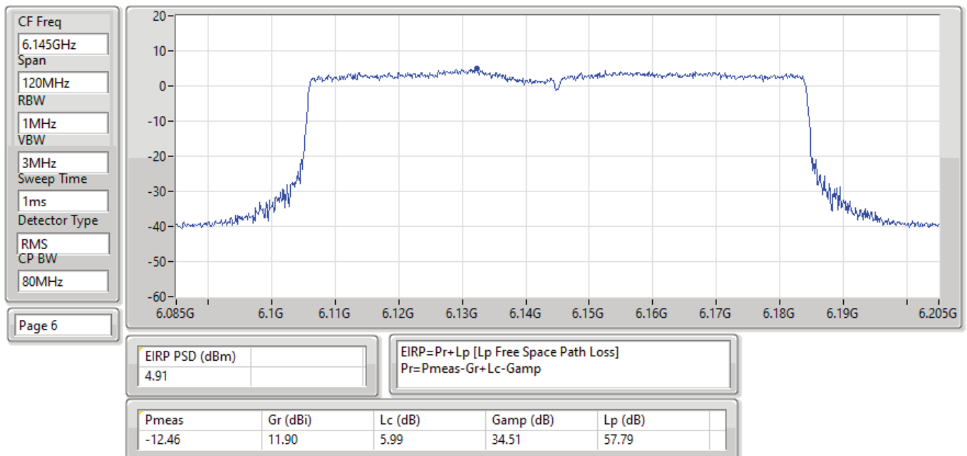
EIRP PSD;Band:6.2G;ax80,BF;BWch:80MHz;Nss:1,(M0);Nant:4;Ch:6145MHz;TX
