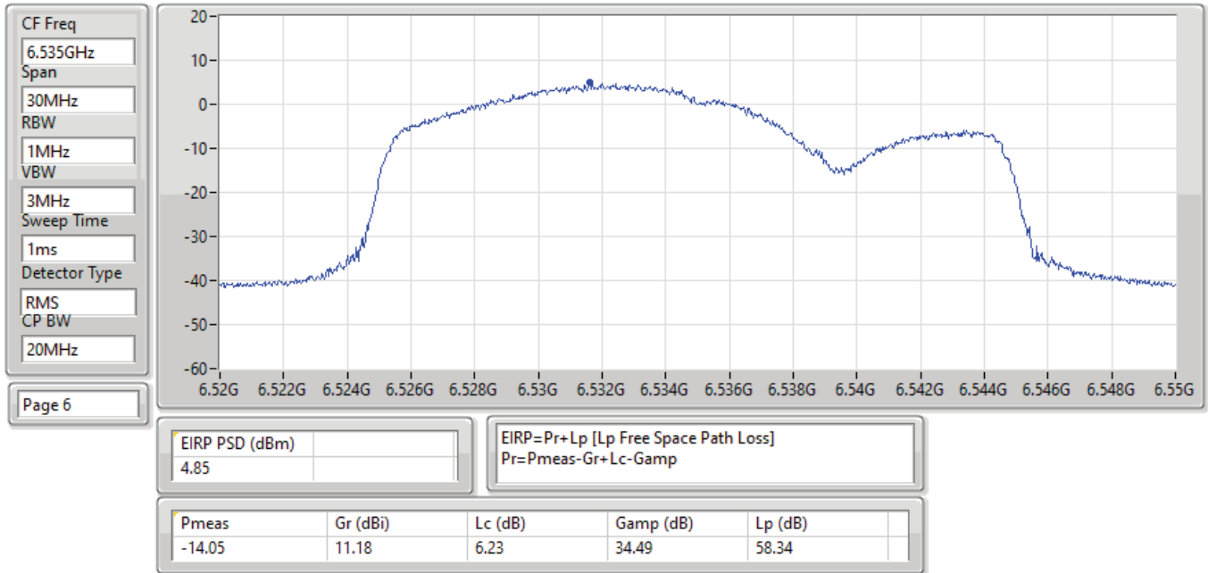
EIRP PSD;Band:6.7G;ax20;BWch:20MHz;Nss:1,(M0);Nant:4;Ch:6535MHz;TX
