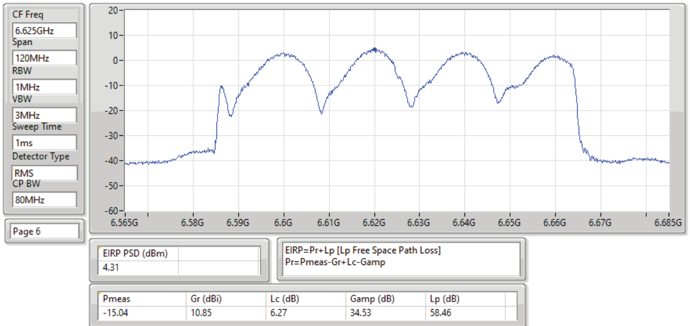
EIRP PSD;Band:6.7G;ax80;BWch:80MHz;Nss:1,(M0);Nant:4;Ch:6625MHz;TX
