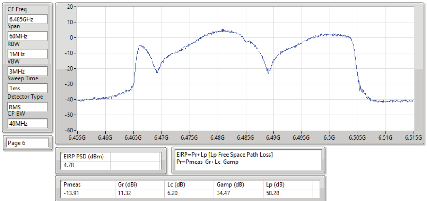
EIRP PSD;Band:6.4G;ax40;BWch:40MHz;Nss:1,(M0);Nant:4;Ch:6485MHz;TX
