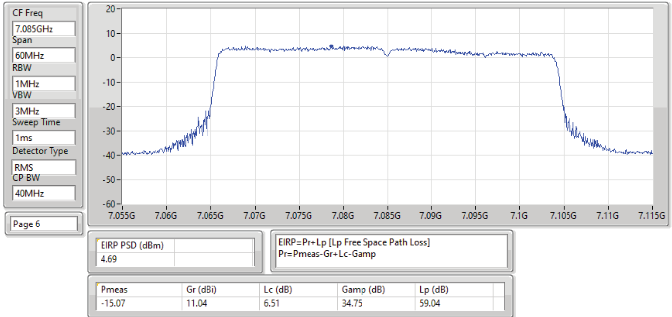
EIRP PSD;Band:7.0G;ax40,BF;BWch:40MHz;Nss:1,(M0);Nant:4;Ch:7085MHz;TX
