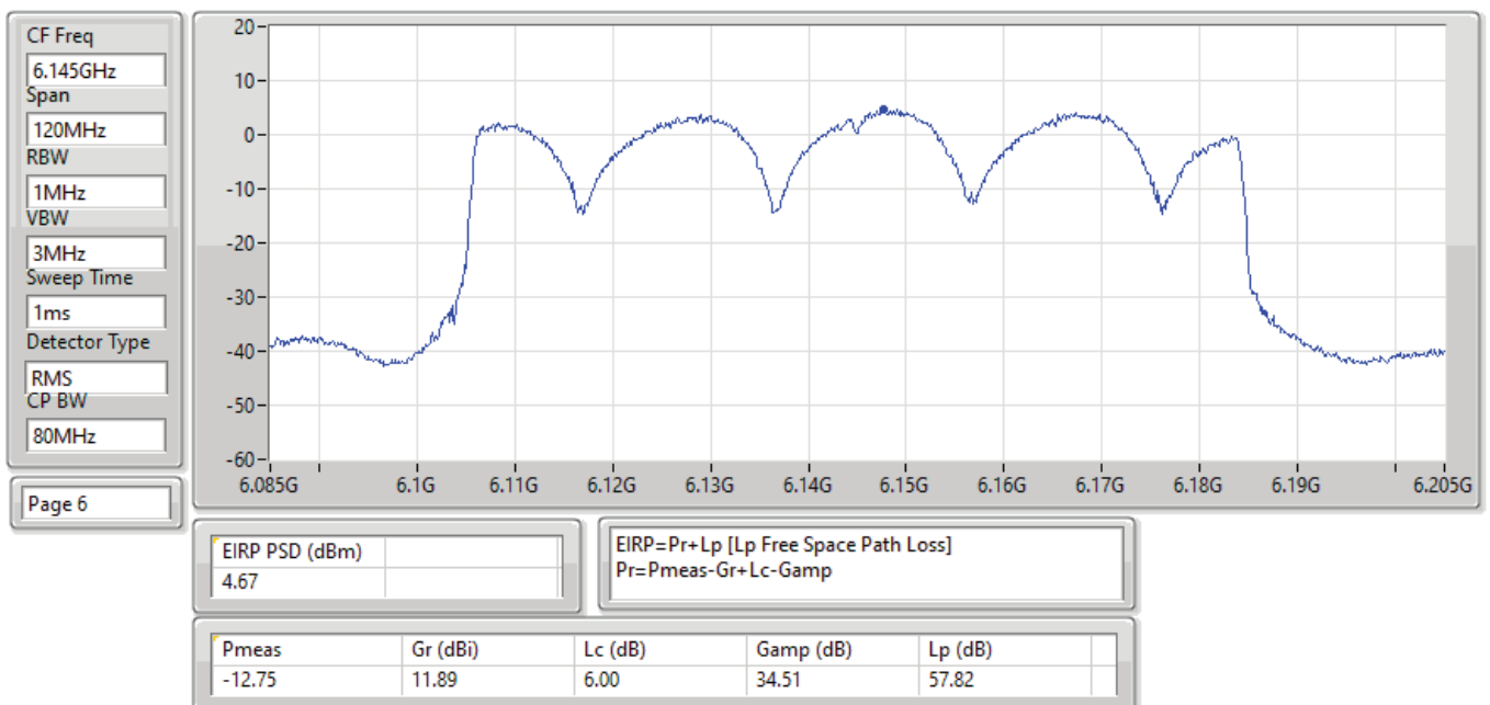
EIRP PSD;Band:6.2G;ax80;BWch:80MHz;Nss:1,(M0);Nant:4;Ch:6145MHz;TX
