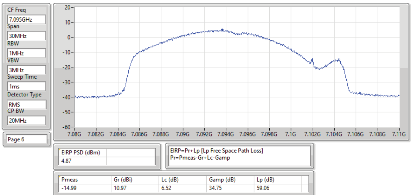
EIRP PSD;Band:7.0G;ax20;BWch:20MHz;Nss:1,(M0);Nant:4;Ch:7095MHz;TX
