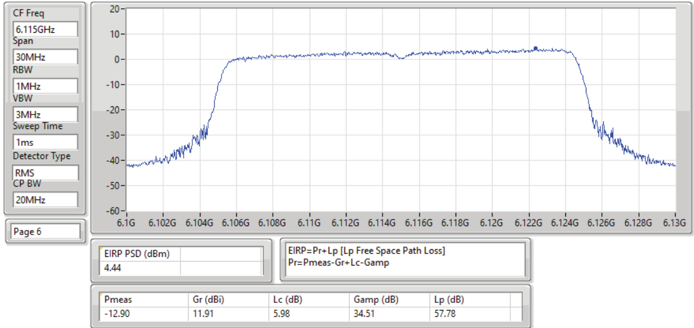
EIRP PSD;Band:6.2G;ax20,BF;BWch:20MHz;Nss:1,(M0);Nant:4;Ch:6115MHz;TX
