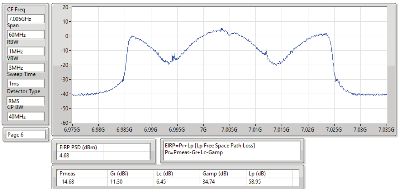
EIRP PSD;Band:7.0G;ax40;BWch:40MHz;Nss:1,(M0);Nant:4;Ch:7005MHz;TX
