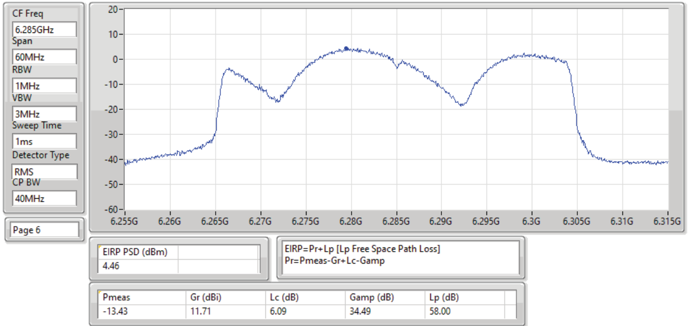
EIRP PSD;Band:6.2G;ax40;BWch:40MHz;Nss:1,(M0);Nant:4;Ch:6285MHz;TX
