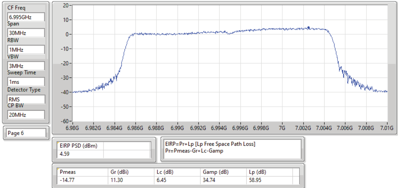
EIRP PSD;Band:7.0G;ax20,BF;BWch:20MHz;Nss:1,(M0);Nant:4;Ch:6995MHz;TX
