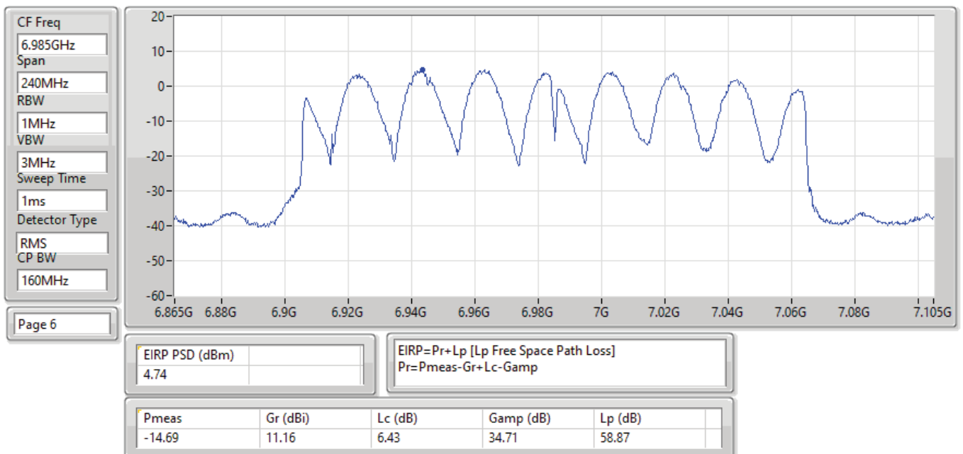
EIRP PSD;Band:7.0G;ax160;BWch:160MHz;Nss:1,(M0);Nant:4;Ch:6985MHz;TX
