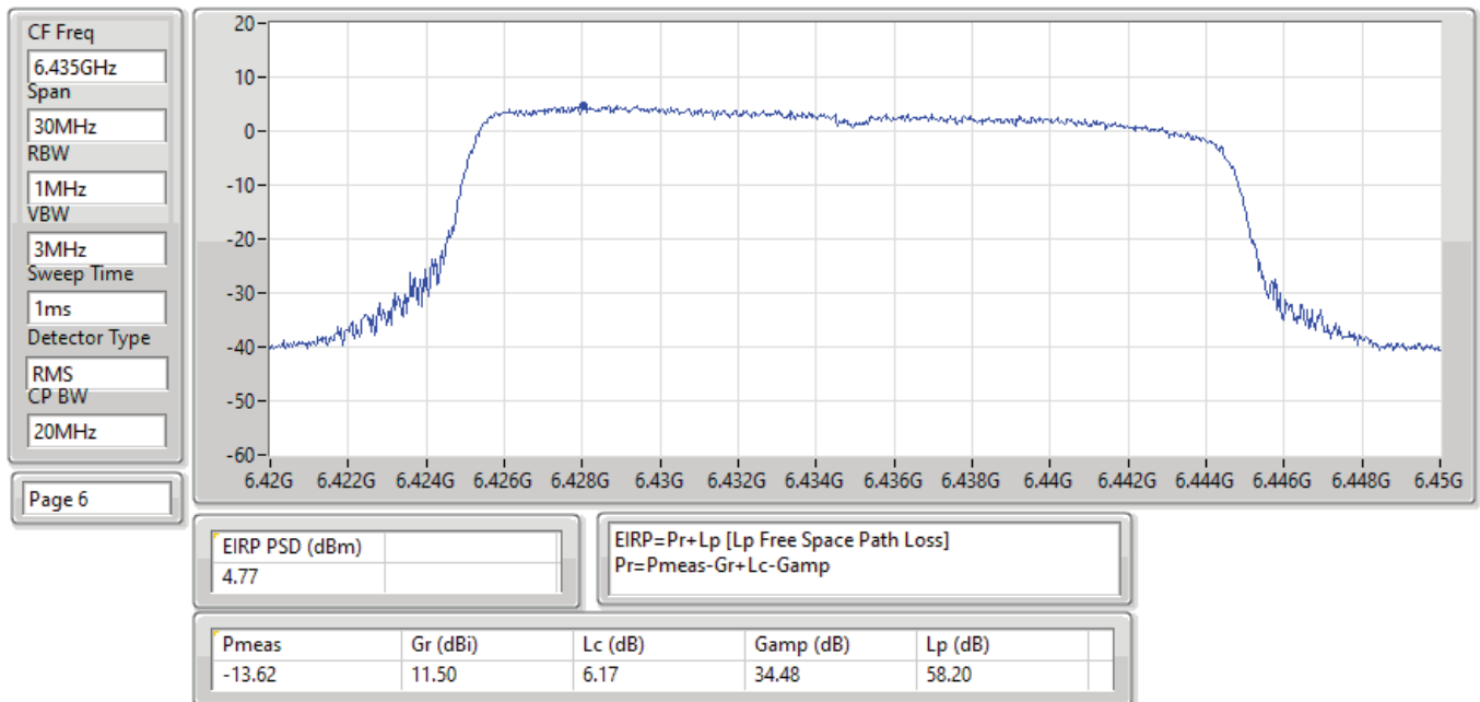
EIRP PSD;Band:6.4G;ax20,BF;BWch:20MHz;Nss:1,(M0);Nant:4;Ch:6435MHz;TX
