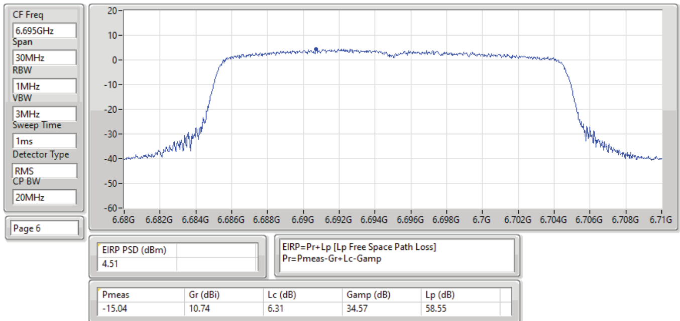
EIRP PSD;Band:6.7G;ax20,BF;BWch:20MHz;Nss:1,(M0);Nant:4;Ch:6695MHz;TX
