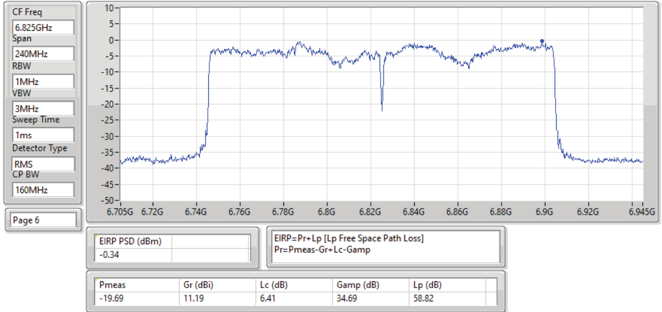
EIRP PSD;Band:6.7G;ax160,BF;BWch:160MHz;Nss:1,(M0);Nant:4;Ch:6825MHz;TX
