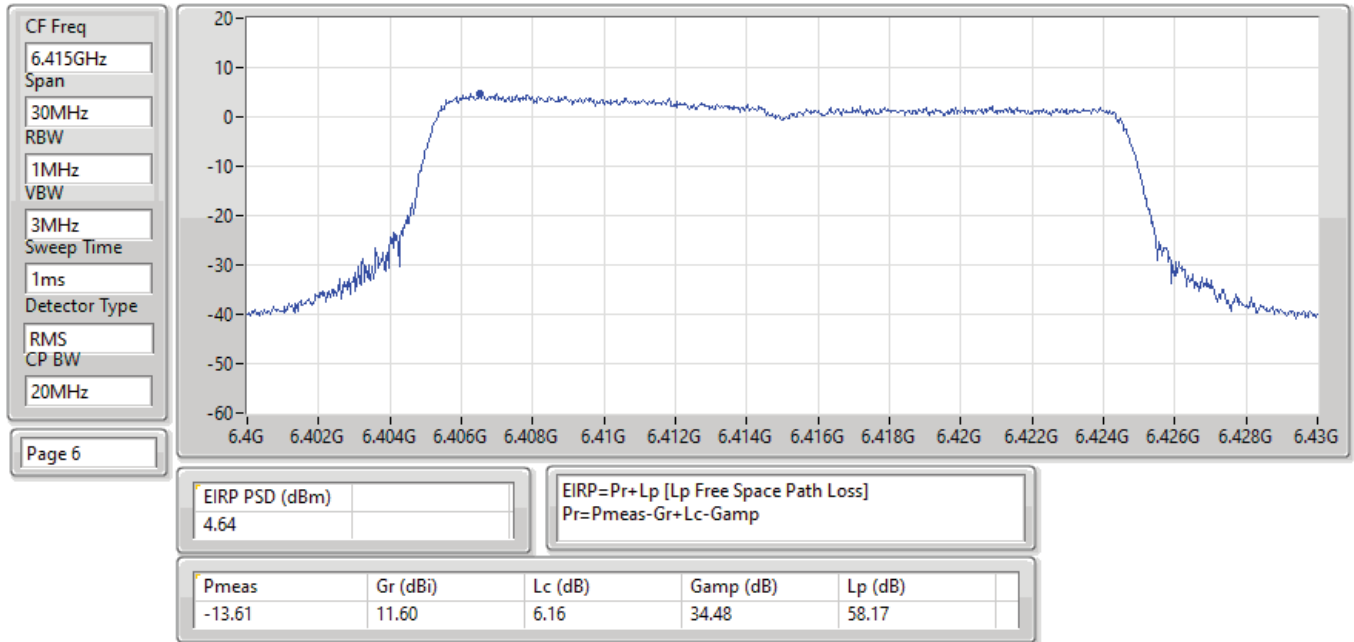
EIRP PSD;Band:6.2G;ax20,BF;BWch:20MHz;Nss:1,(M0);Nant:4;Ch:6415MHz;TX
