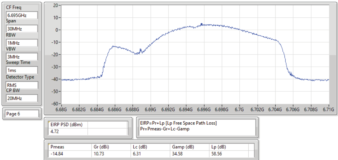
EIRP PSD;Band:6.7G;ax20;BWch:20MHz;Nss:1,(M0);Nant:4;Ch:6695MHz;TX
