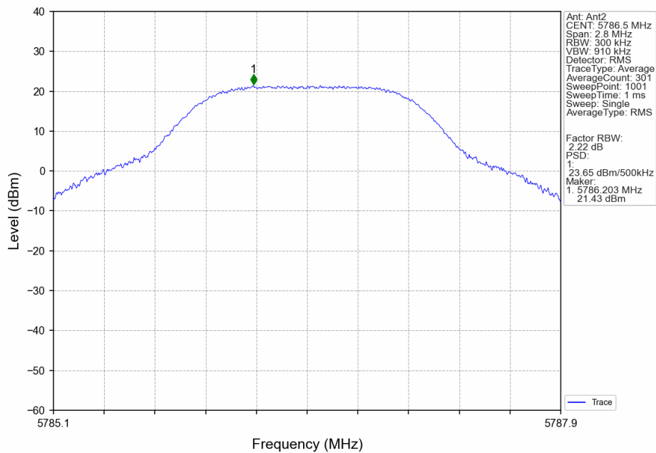
1.4M_MCH_5786.5MHz_Ant2_NTNV
