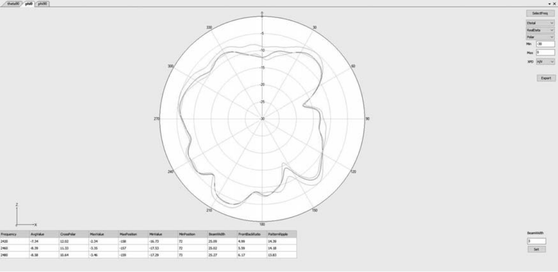
GPS(L1)/WIFI2.4 Phi=0deg
