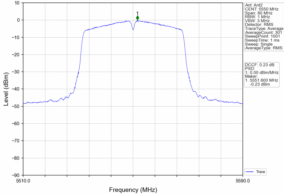
802.11n(HT40)_MCH_5550MHz_MIMO_NTNV
