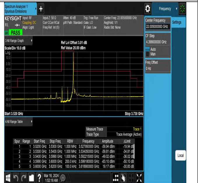
Band43_20MHz_QPSK_43690_1RB#99
