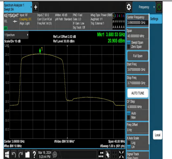
43(3600-3700)-20MHz-16QAM-44490-1RB#0-PASS
