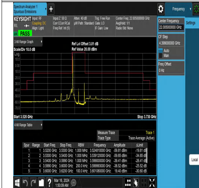
Band43_20MHz_QPSK_43690_1RB#0
