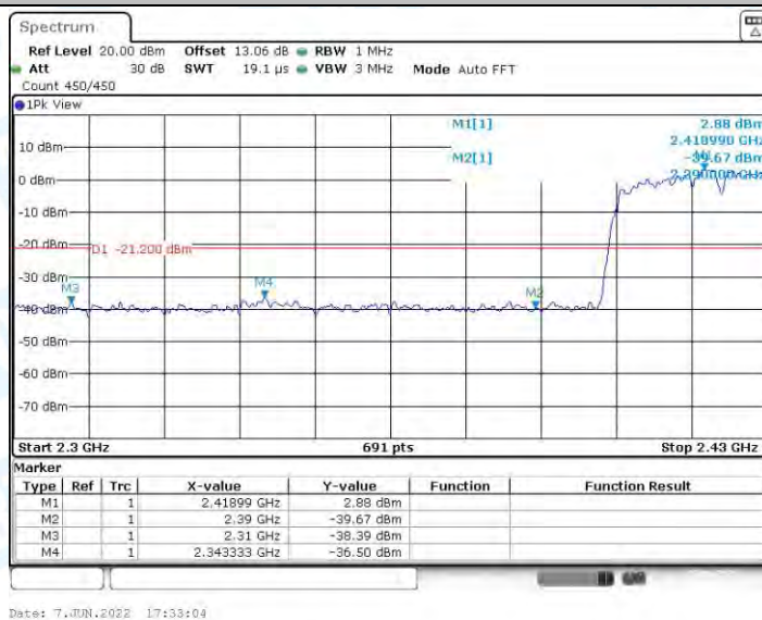
11AX40MIMO_Ant1_Low_2422_Peak
