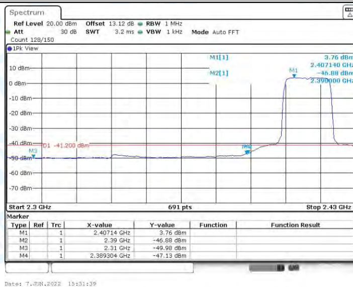
11G_Ant1_Low_2412_AV
