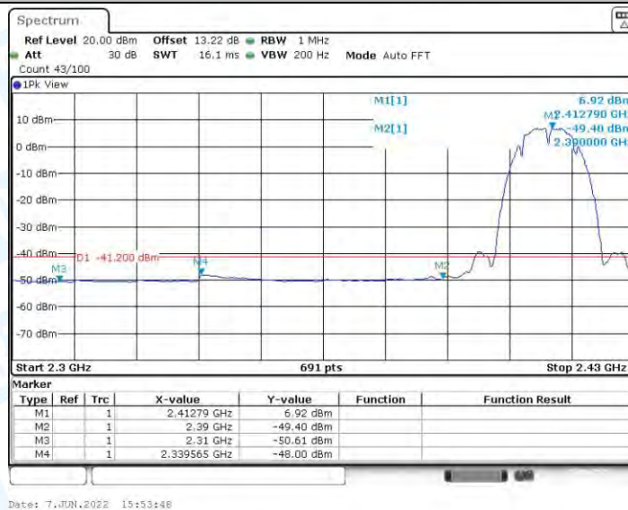
11B_Ant2_Low_2412_AV
