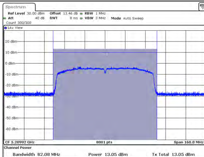
11AC80SISO_Ant2_5210
