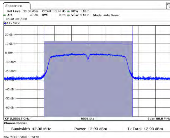
11AC40SISO_Ant2_5550
