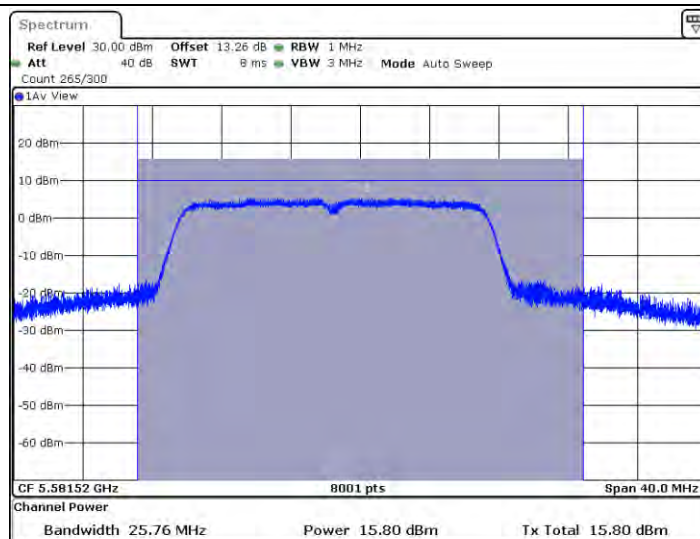
11N20SISO_Ant2_5580
