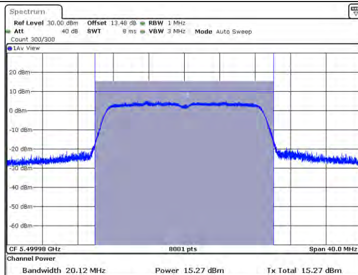
11N20MIMO_Ant2_5500
