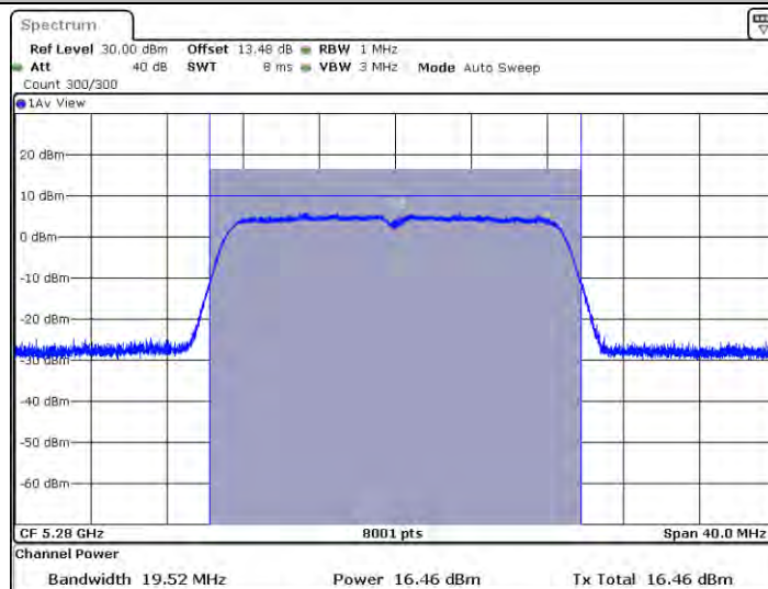
11N20SISO_Ant2_5280
