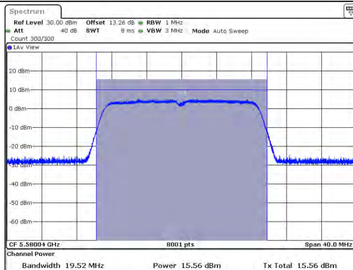
11N20SISO_Ant2_5580
