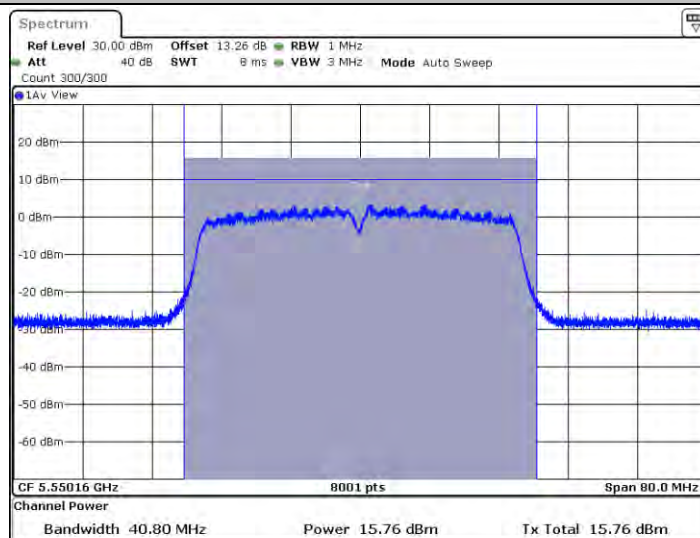
11N40MIMO_Ant2_5550
