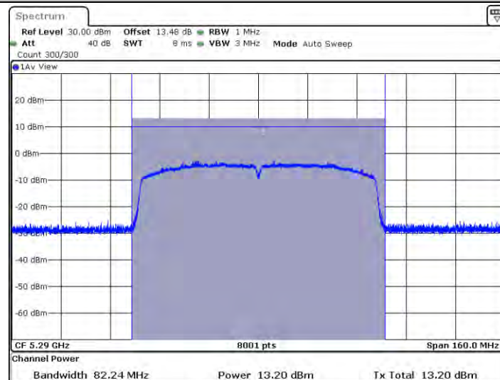
11AC80SISO_Ant2_5290
