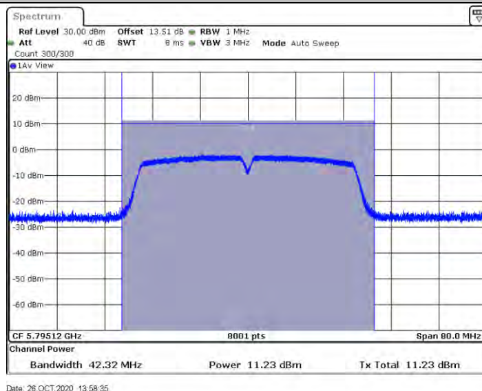
11AC40SISO_Ant2_5795
