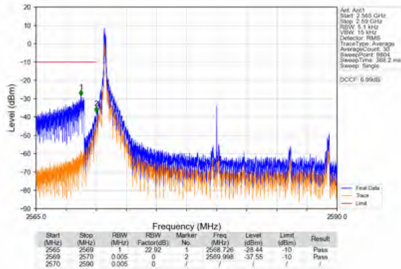
n38_15kHz_SISO_NTNV_20MHz_DFT-s-OFDM QPSK_2580MHz_Inner_1RB_Left
