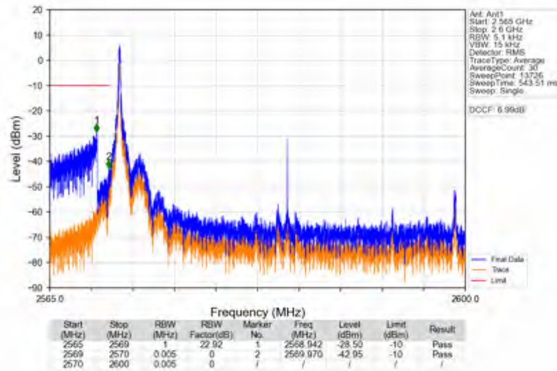
n38_15kHz_SISO_NTNV_30MHz_DFT-s-OFDM_QPSK_2585MHz_Inner_1RB_Left
