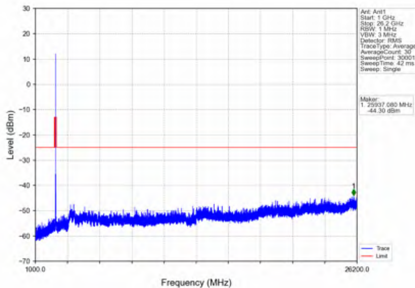
n38 15kHz SISO NTN 25MHz CP-OFDM QPSK 2607.5MHz Edge 1RB Right
