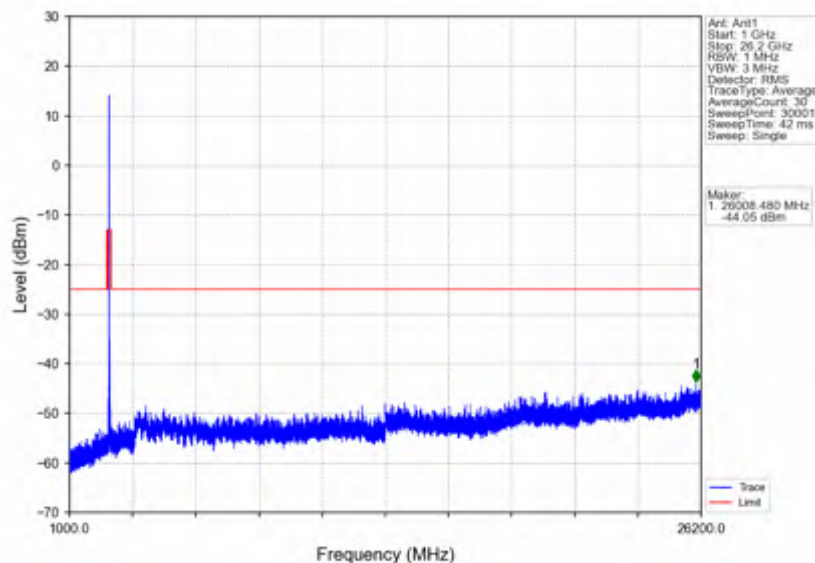
n38 15kHz SISO NTNv 40MHz DFT-s-OFDM QPSK 2600MHz Edge 1RB Right
