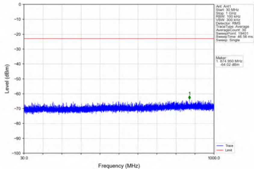
n38_15kHz_SISO_NTNV_20MHz_DFT-s-OFDM QPSK_2580MHz_Edge_1RB_Left
