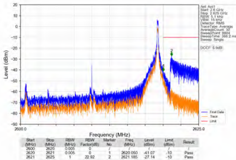
n38_15kHz_SISO_NTNV_20MHz_DFT-s-OFDM_PI/2_BPSK_2610MHz_Inner_1RB_Right
