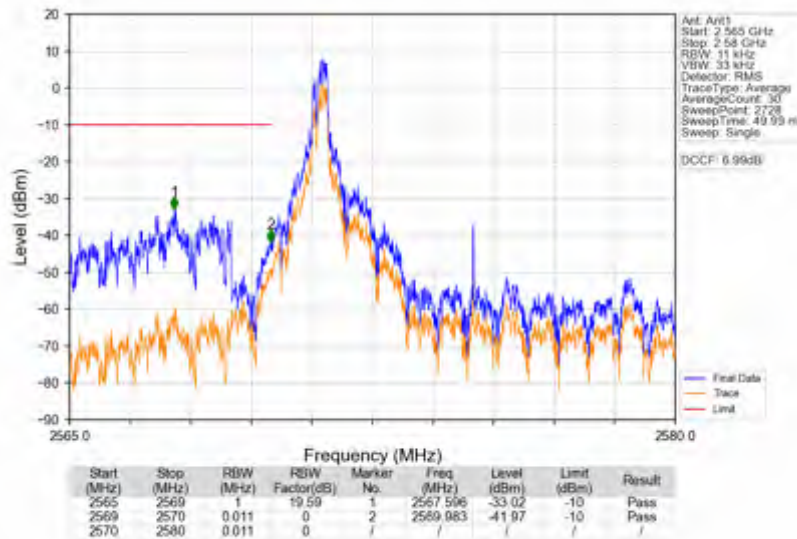
n38_30kHz_SISO_NTNV_10MHz_DFT-s-OFDM QPSK_2575MHz_Inner_1RB_Left
