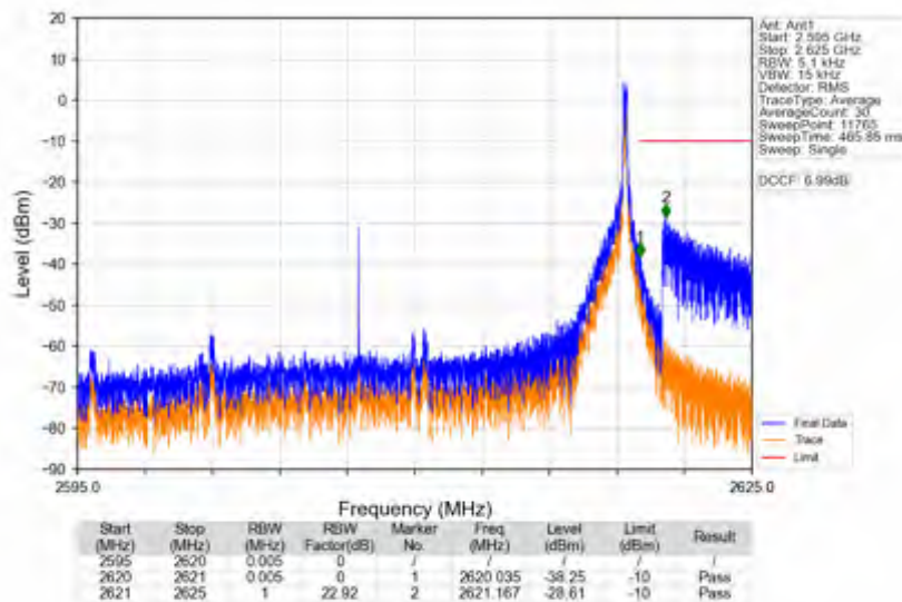
n38 15kHz SISO NTN 25MHz CP-OFDM QPSK 2607.5MHz Edge 1RB Right
