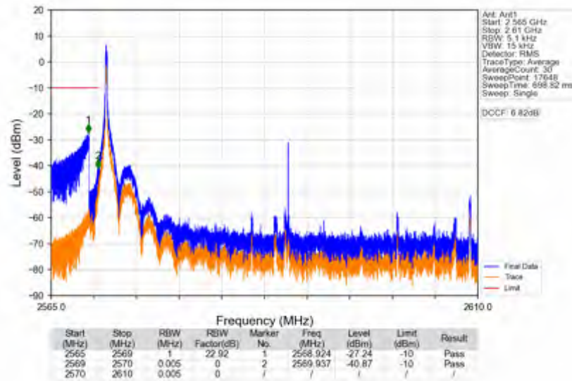
n38_15kHz_SISO_NTNV_40MHz_DFT-s-OFDM_PI/2_BPSK_2590MHz_Inner_1RB_Left
