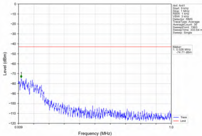
n38_15kHz_SISO_NTNV_40MHz_CP-OFDM_QPSK_2590MHz_Edge_1RB_Left
