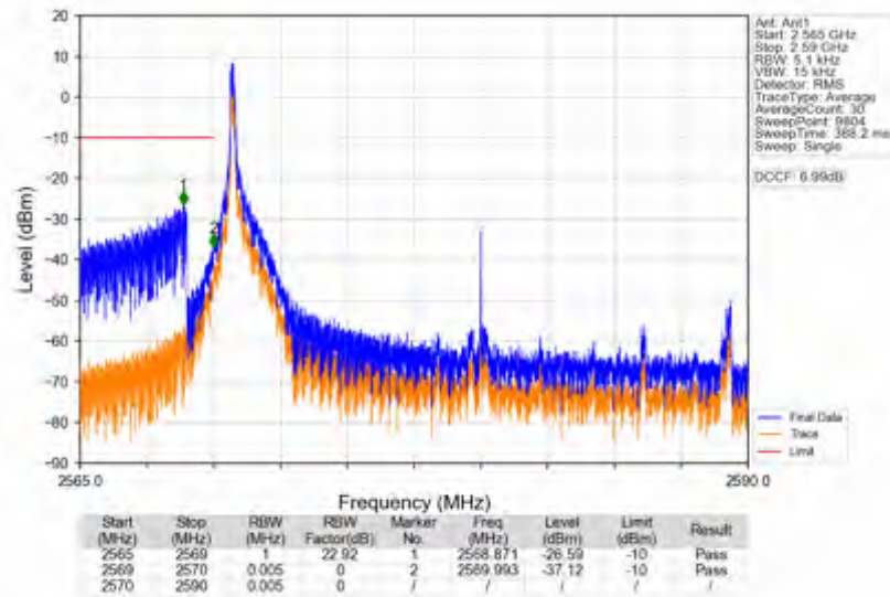
n38_15kHz_SISO_NTNV_20MHz_DFT-s-OFDM_PI/2_BPSK_2580MHz_Inner_1RB_Left
