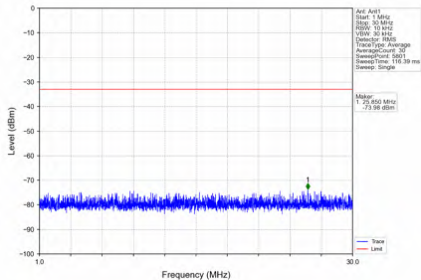
n38_30kHz_SISO_NTNV_10MHz_DFT-s-OFDM QPSK_2595MHz_Edge_1RB_Left
