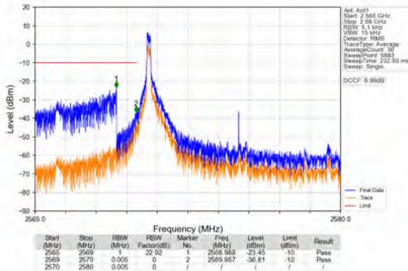
n38_15kHz_SISO_NTNV_10MHz_DFT-s-OFDM_QPSK_2575MHz_Inner_1RB_Left
