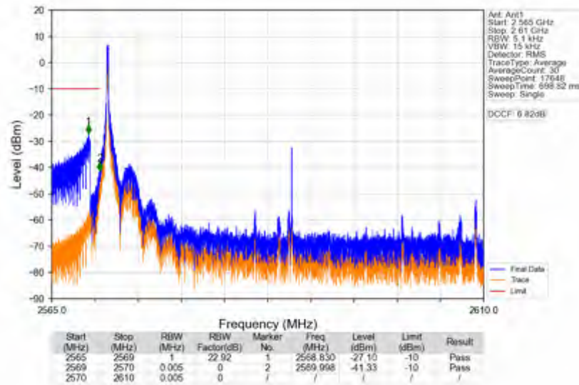
n38_15kHz_SISO_NTNV_40MHz_DFT-s-OFDM QPSK_2590MHz_Inner_1RB_Left
