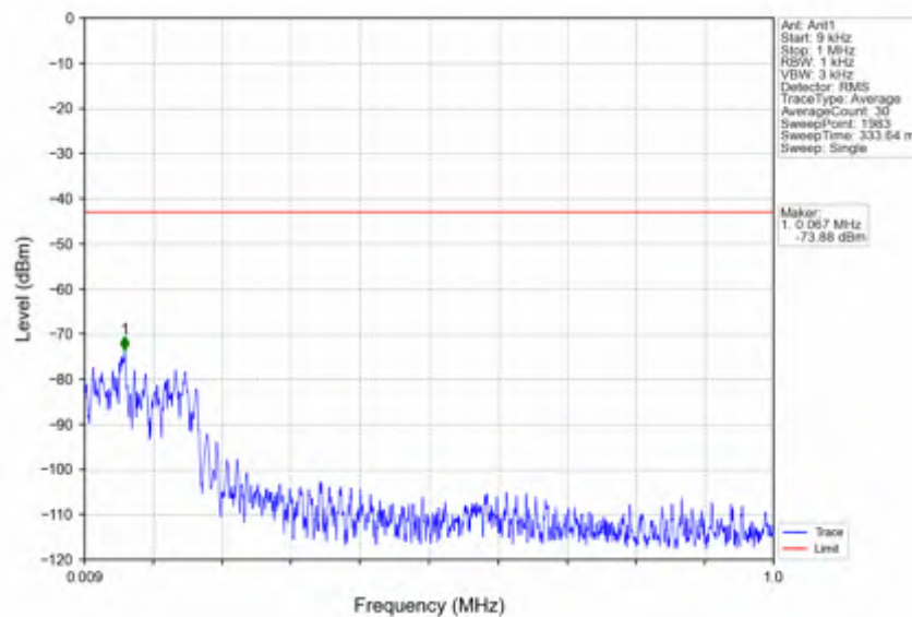
n38_15kHz_SISO_NTNV_20MHz_DFT-s-OFDM_PI/2_BPSK_2595MHz_Edge_1RB_Left
