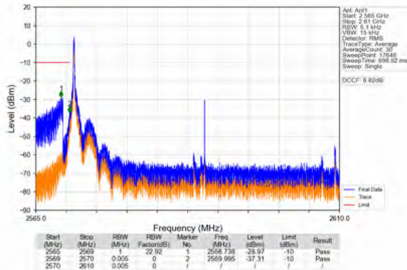
n38_15kHz_SISO_NTNV_40MHz_CP-OFDM_QPSK_2590MHz_Edge_1RB_Left
