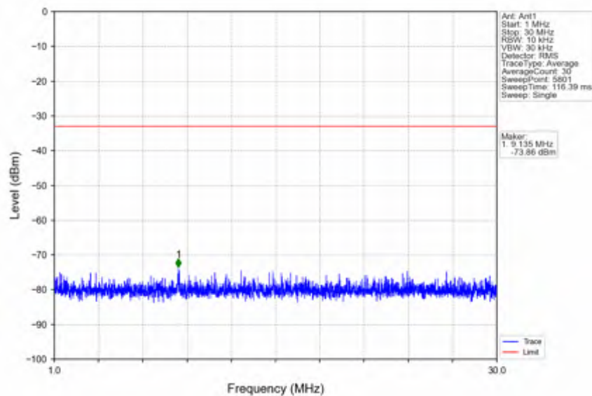
n38 15kHz SISO NTN 10MHz CP-OFDM QPSK 2575MHz Edge 1RB Left
