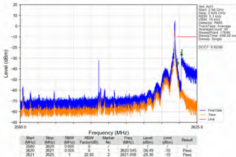
n38 15kHz SISO NTNv 40MHz DFT-s-OFDM QPSK 2600MHz Edge 1RB Right
