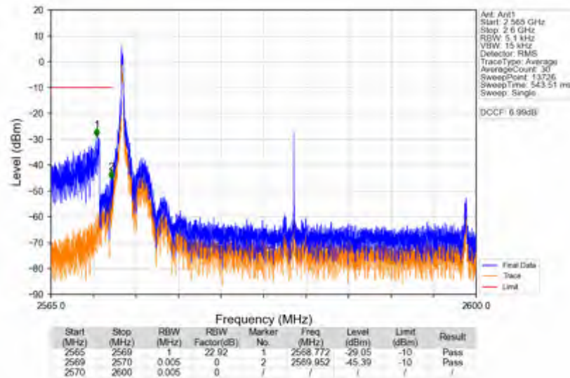
n38_15kHz_SISO_NTNV_30MHz_CP-OFDM_QPSK_2585MHz_Inner_1RB_Left
