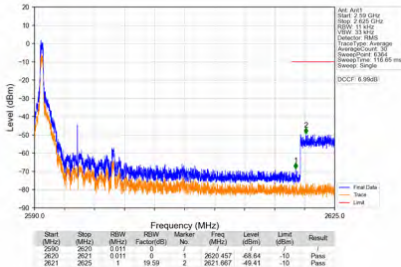
n38_30kHz_SISO_NTNV_10MHz_DFT-s-OFDM QPSK_2595MHz_Edge_1RB_Left
