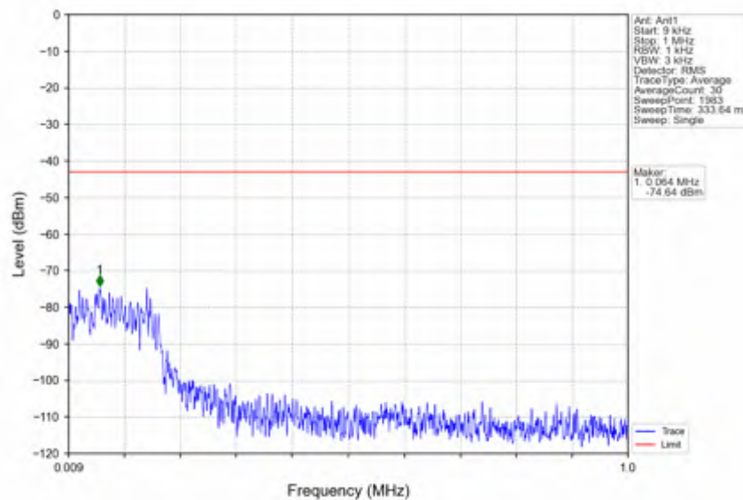
n38_15kHz_SISO_NTNV_20MHz_DFT-s-OFDM QPSK_2595MHz_Edge_1RB_Left
