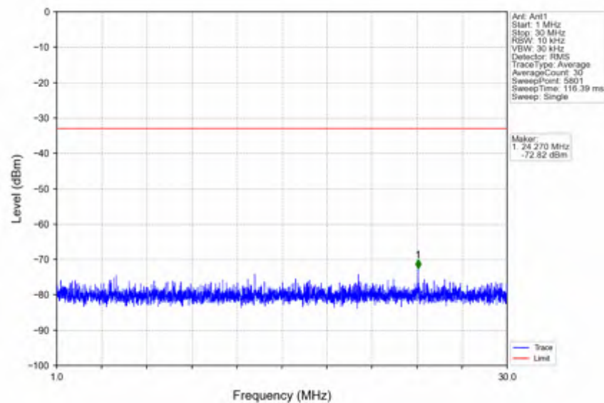
n38_15kHz_SISO_NTNV_20MHz_CP-OFDM QPSK_2595MHz_Edge_1RB_Left
