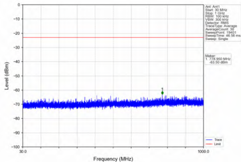
n38 15kHz SISO NTNV 40MHz DFT-s-OFDM PI/2 BPSK 2600MHz Edge 1RB Right
