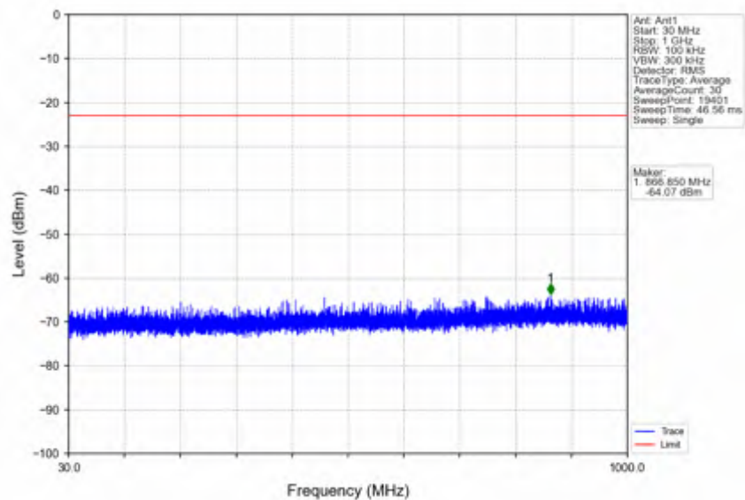
n38_15kHz_SISO_NTNV_40MHz_CP-OFDM QPSK_2595MHz_Edge_1RB_Left
