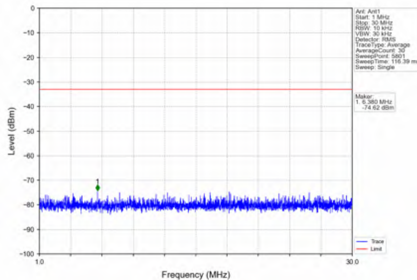
n38_15kHz_SISO_NTNV_40MHz_CP-OFDM QPSK_2590MHz_Edge_1RB_Left
