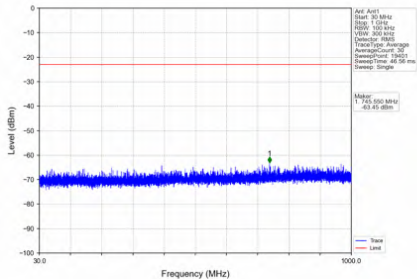
n38_15kHz_SISO_NTNV_20MHz_DFT-s-OFDM QPSK_2595MHz_Edge_1RB_Left
