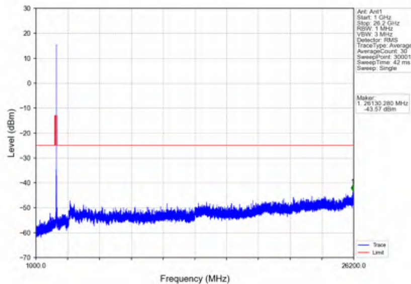
n38 15kHz SISO NTV 30MHz DFT-s-OFDM QPSK 2605MHz Edge 1RB Right
