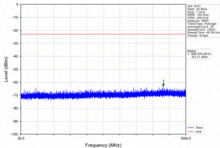
n38 15kHz SISO NTN 40MHz CP-OFDM QPSK 2600MHz Edge 1RB Right
