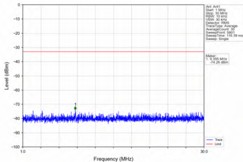
n38_15kHz_SISO_NTNV_40MHz_DFT-s-OFDM QPSK_2590MHz_Edge_1RB_Left
