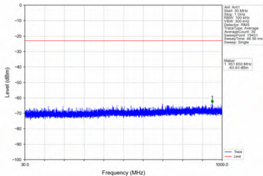
n38 15kHz SISO NTNV 20MHz DFT-s-OFDM QPSK 2610MHz Edge 1RB Right
