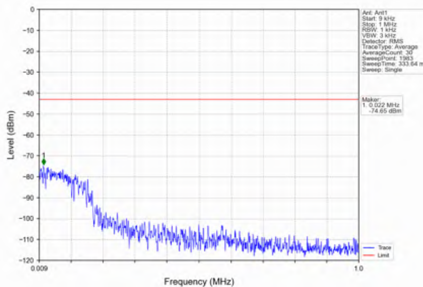
n38 15kHz SISO NTN 15MHz CP-OFDM QPSK 2595MHz Edge 1RB Left
