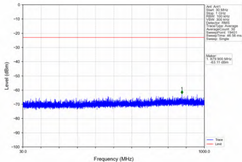
n38_15kHz_SISO_NTNV_20MHz_CP-OFDM QPSK_2595MHz_Edge_1RB_Left
