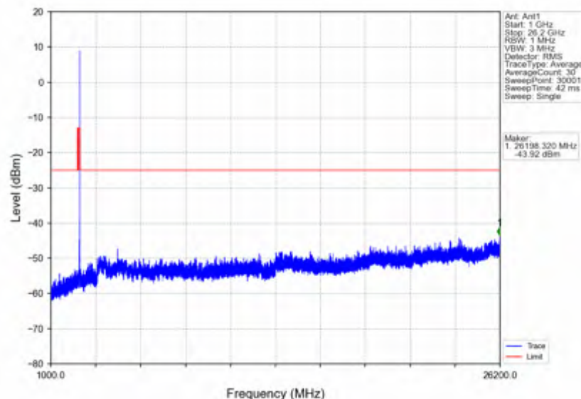
n38 15kHz SISO NTN 15MHz CP-OFDM QPSK 2612.5MHz Edge 1RB Right
