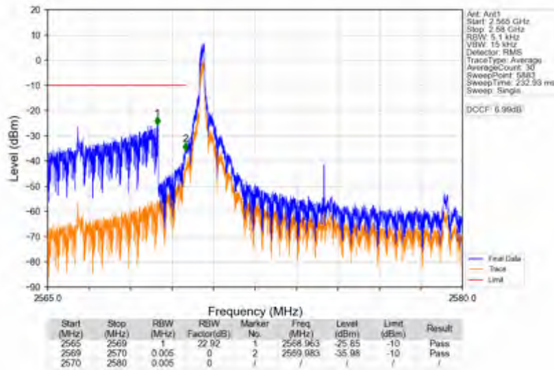
n38_15kHz_SISO_NTNV_10MHz_DFT-s-OFDM PI/2 BPSK_2575MHz_Inner_1RB_Left
