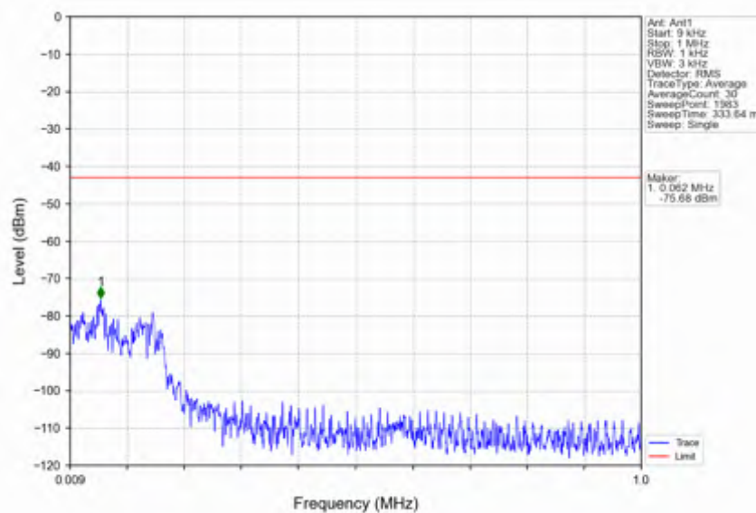
n38_15kHz_SISO_NTNV_40MHz_DFT-s-OFDM_PI/2_BPSK_2595MHz_Edge_1RB_Left
