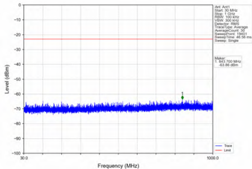
n38 15kHz SISO NTN 15MHz CP-OFDM QPSK 2612.5MHz Edge 1RB Right
