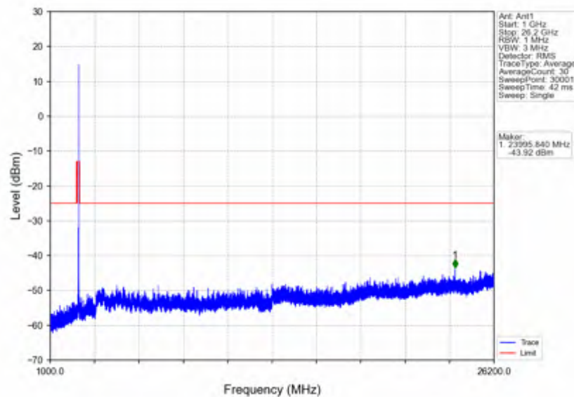
n38 15kHz SISO NTN 40MHz CP-OFDM QPSK 2600MHz Edge 1RB Right
