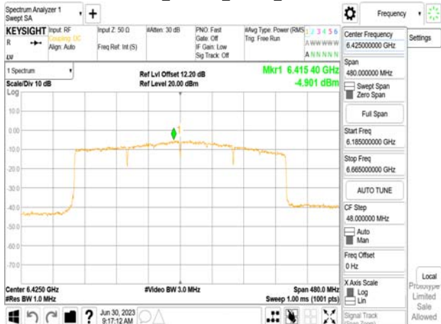
802.11be_320MHz_Chain0_6425MHz
