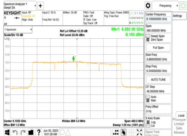
802.11be_320MHz_Chain1_6105MHz_2x996+484 MRU6
