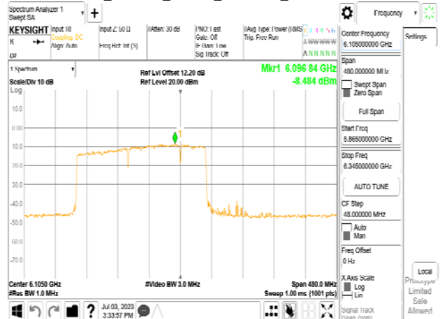
802.11be_320MHz_Chain1_6105MHz_2x996+484 MRU6
