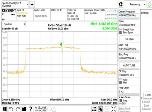
802.11be_160MHz_Chain1_6665MHz_RU996+484_Punc40
