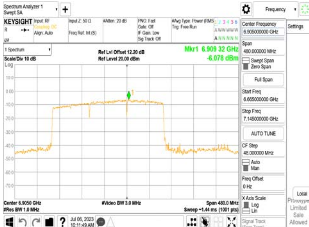
802.11be_320MHz_Chain1_6905MHz_3x996_MRU4
