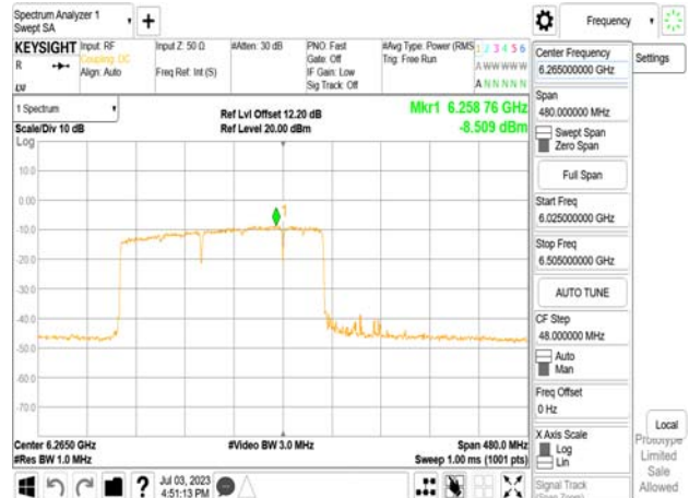
802.11be_320MHz_Chain1_6265MHz_3x996 MRU4
