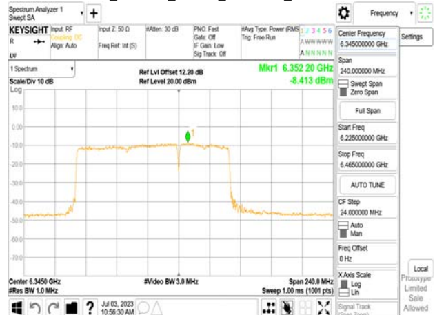
802.11be_160MHz_Chain1_6345MHz_996+484 MRU4
