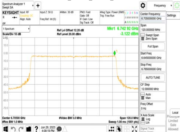
802.11be_80MHz_Chain0_6705MHz
