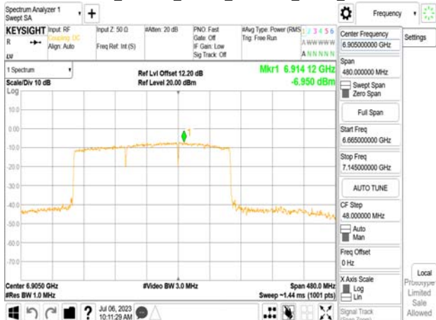
802.11be_320MHz_Chain0_6905MHz_3x996_MRU4
