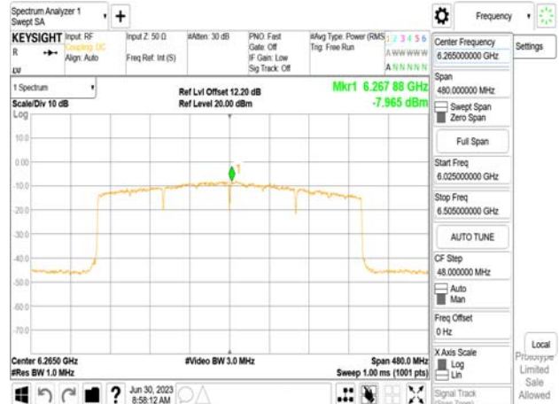
802.11be_320MHz_Chain1_6265MHz_2x996+484 MRU6
