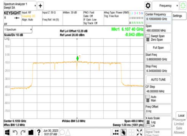
802.11be_320MHz_Chain0_6105MHz_2x996+484 MRU6
