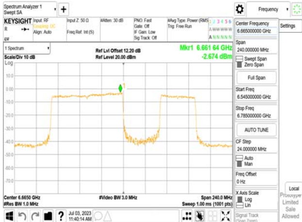
802.11be_160MHz_Chain1_6665MHz_RU996_67
