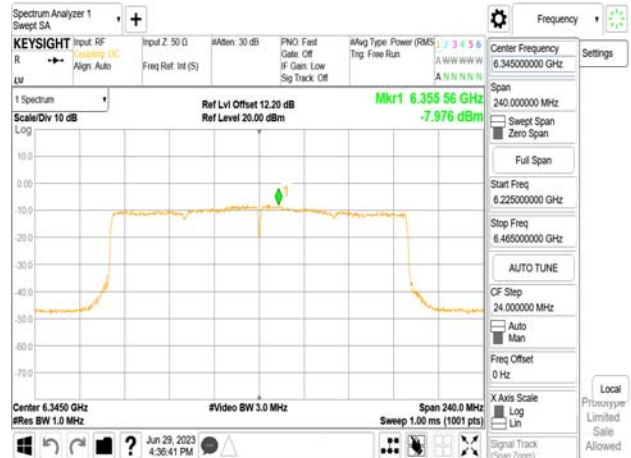
802.11be_160MHz_Chain1_6345MHz_996+484 MRU4
