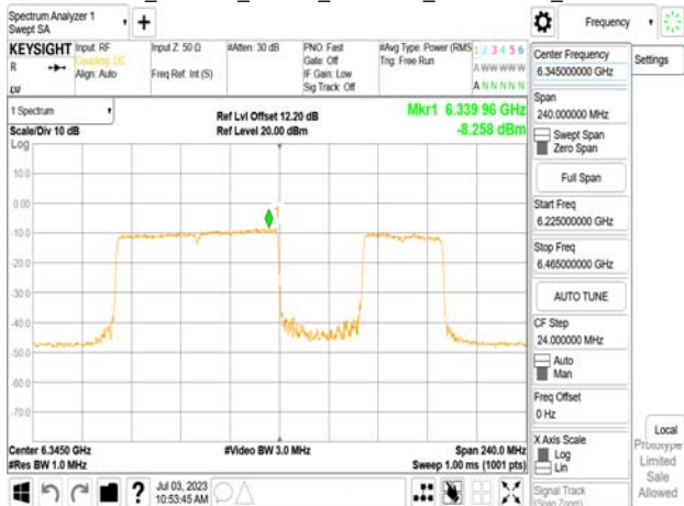
802.11be_160MHz_Chain1_6345MHz_RU996_67
