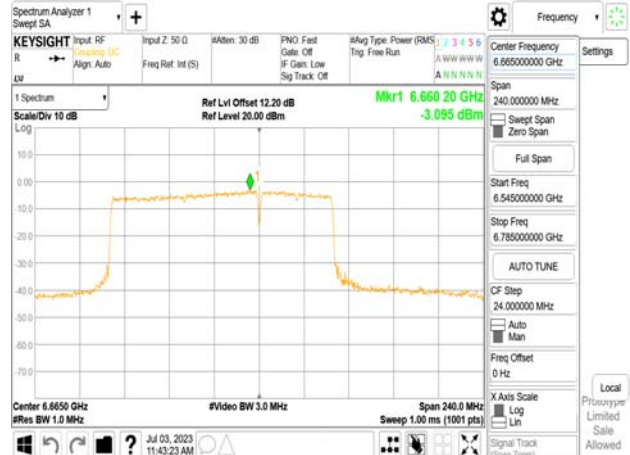
802.11be_160MHz_Chain0_6665MHz_996+484_MRU4
