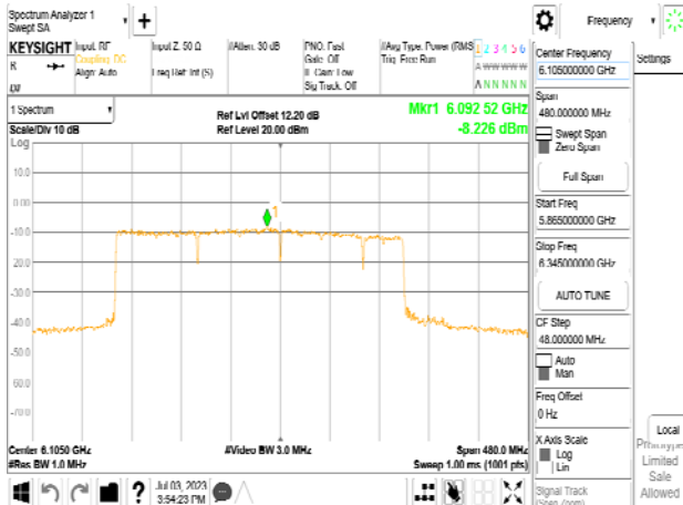
802.11be_320MHz_Chain1_6105MHz_RU996x2+484_Punc40
