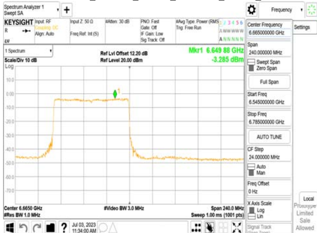
802.11be_160MHz_Chain1_6665MHz_RU996_67
