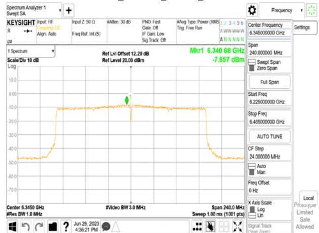
802.11be_160MHz_Chain0_6345MHz_996+484 MRU4
