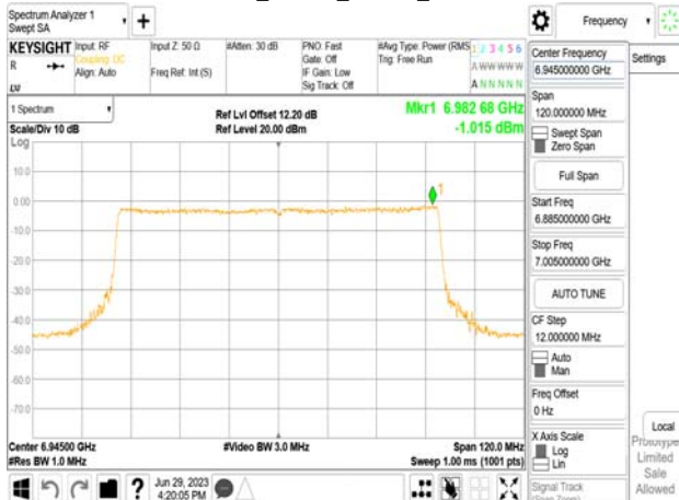
802.11be_80MHz_Chain1_6945MHz
