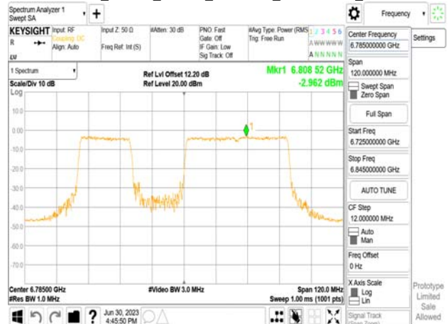
802.11be_80MHz_Chain1_6785MHz_RU484+242_Punc20
