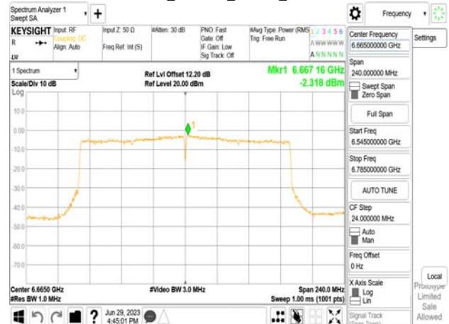
802.11be_160MHz_Chain1_6665MHz
