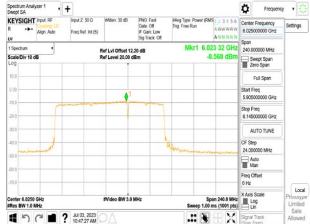
802.11be_160MHz_Chain0_6025MHz_RU996+484_Punc40
