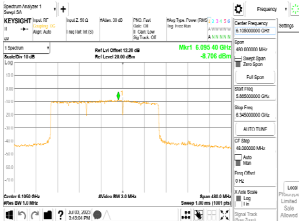
802.11be_320MHz_Chain1_6105MHz_3x996+484 MRU8
