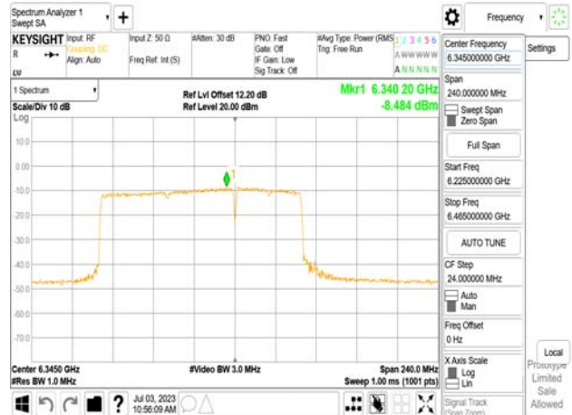
802.11be_160MHz_Chain0_6345MHz_RU996+484_Punc40
