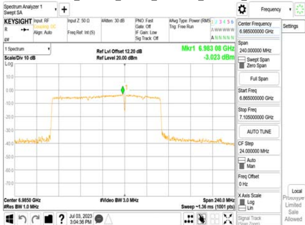
802.11be_160MHz_Chain0_6985MHz_996+484_MRU4
