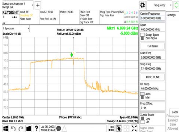
802.11be_320MHz_Chain1_6905MHz_3x996+484 MRU8
