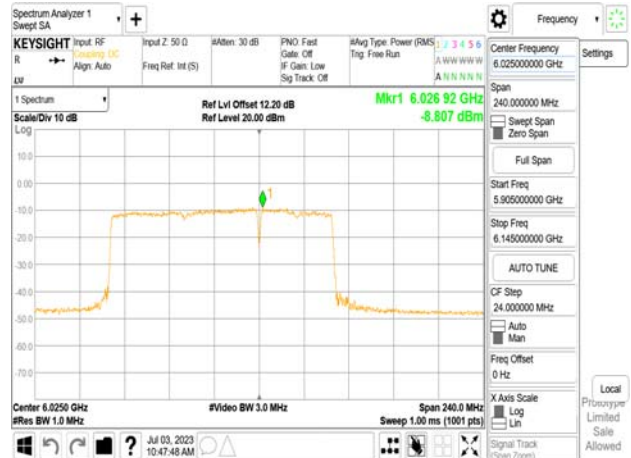
802.11be_160MHz_Chain1_6025MHz_RU996+484_Punc40
