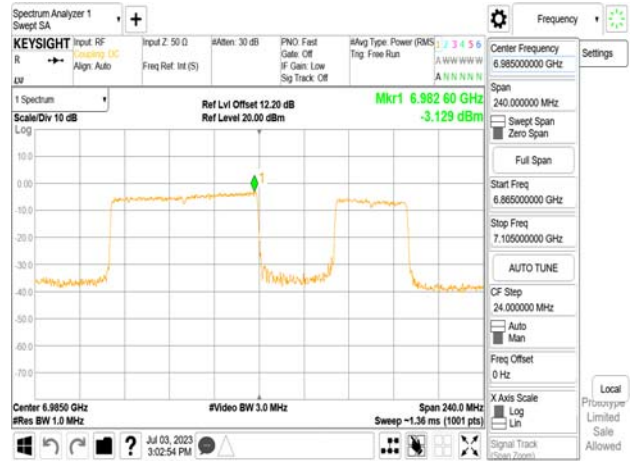
802.11be_160MHz_Chain0_6985MHz_RU996_67
