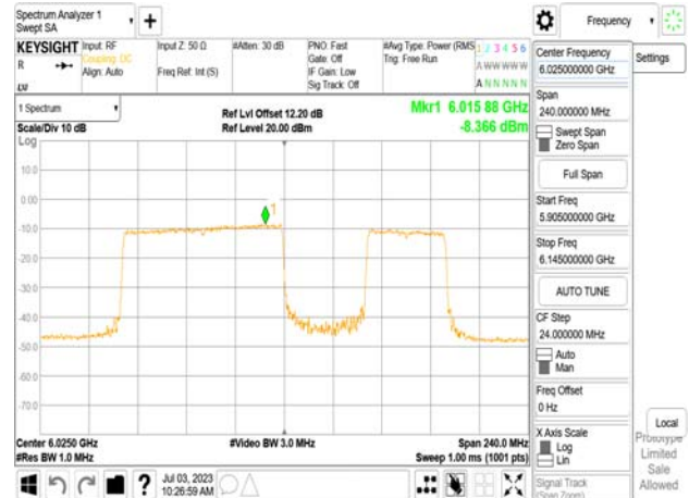
802.11be_160MHz_Chain0_6025MHz_RU996_67
