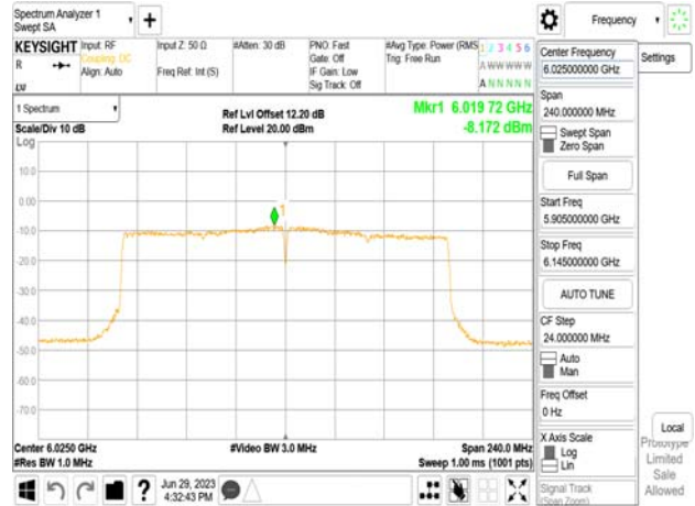
802.11be_160MHz_Chain1_6025MHz_996+484_MR44
