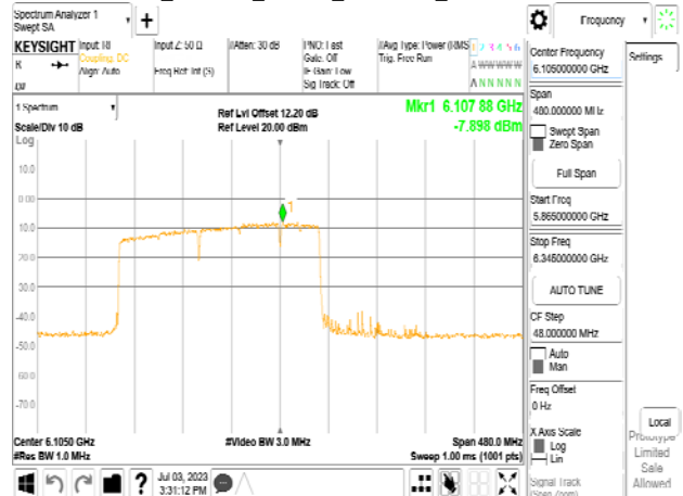
802.11be_320MHz_Chain0_6105MHz_2x996+484 MRU6
