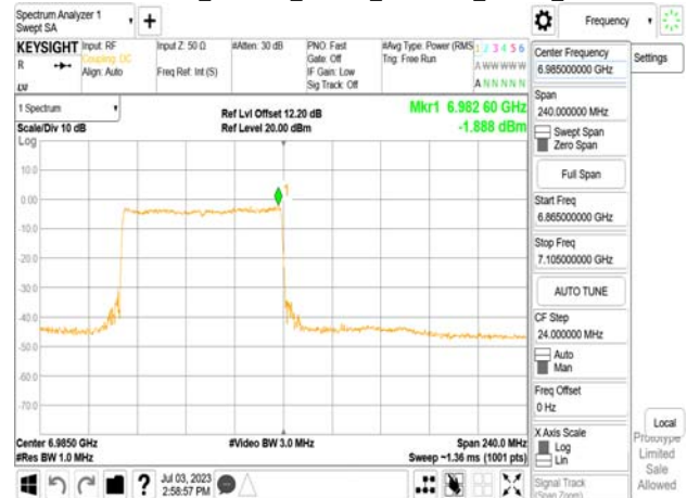
802.11be_160MHz_Chain1_6985MHz_RU996_67
