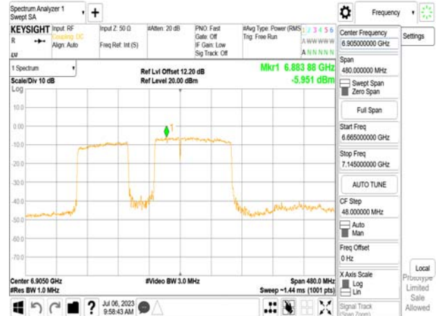
802.11be_320MHz_Chain1_6905MHz_RU996x2+484_Punc40
