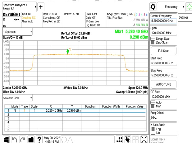
802.11ax_80MHz_Chain0_5290MHz_RU484_66
