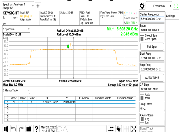
802.11ax_80MHz_Chain2_5610MHz
