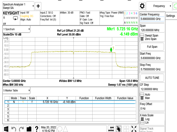
802.11ax_80MHz_Chain2_5690MHz_UNII_3
