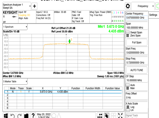
802.11ax_40MHz_Chain2_5670MHz_RU242_62
