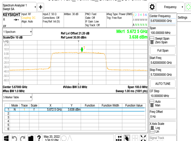
802.11ax_40MHz_Chain3_5670MHz
