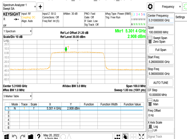
802.11ax_40MHz_Chain3_5310MHz_RU242_62
