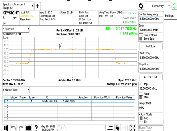
802.11ax_80MHz_Chain3_5530MHz
