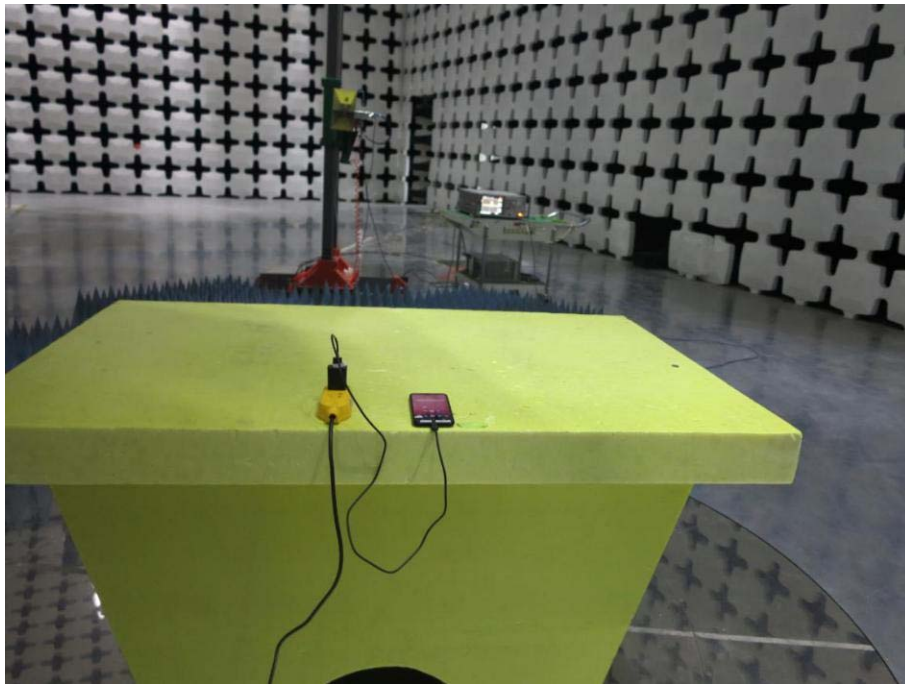
USB 1GHz-18GHz
