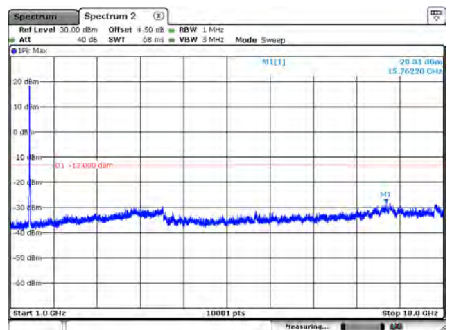
B66_CH132322_15M_1RB0_QPSK_Above 1G
