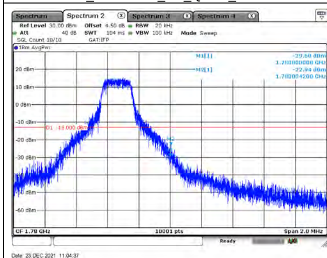
B66_CH132647_5M_QPSK_1RB24
