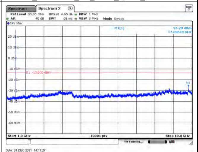
B66_CH132647_5M_1RB0_QPSK_Above 1G
