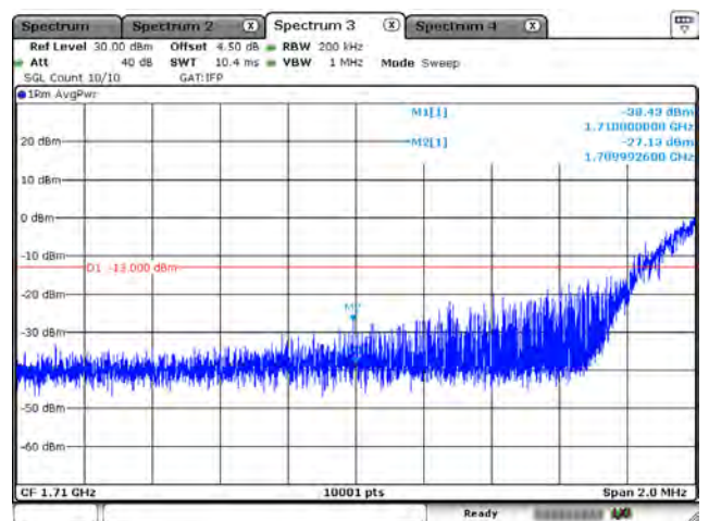
B66_CH132072_20M_QPSK_100RB0
