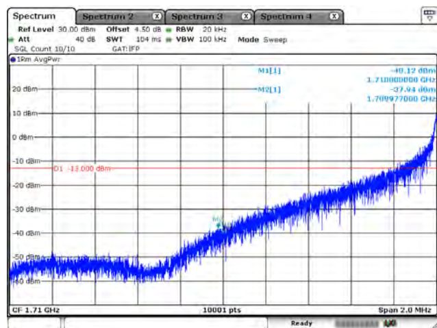
B66_CH132072_20M_QPSK_1RB0
