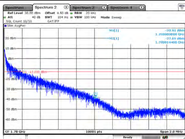
B66_CH132572_20M_QPSK_1RB99
