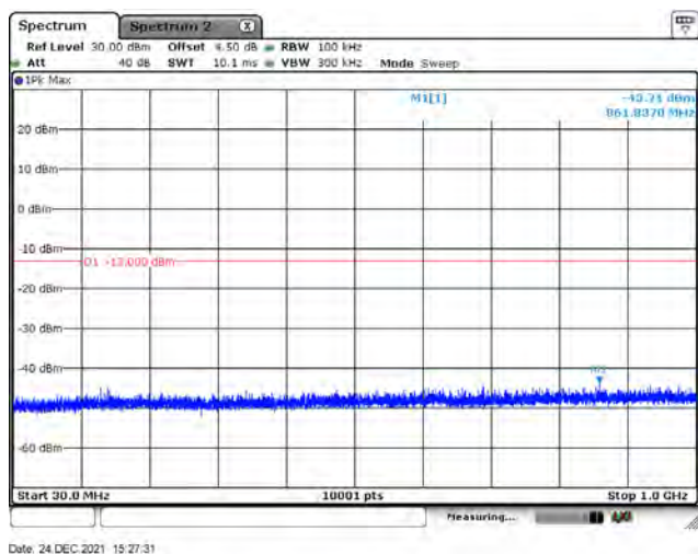
B66_CH132572_20M_1RB0_QPSK_Below 1G
