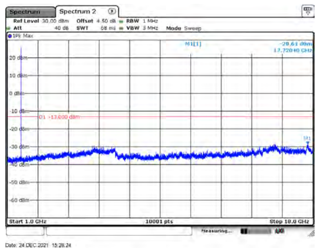
B66_CH132572_20M_1RB0_QPSK_Above 1G
