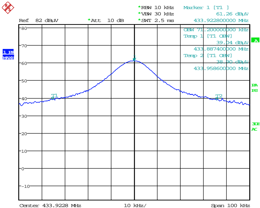
IC 99% OBW
