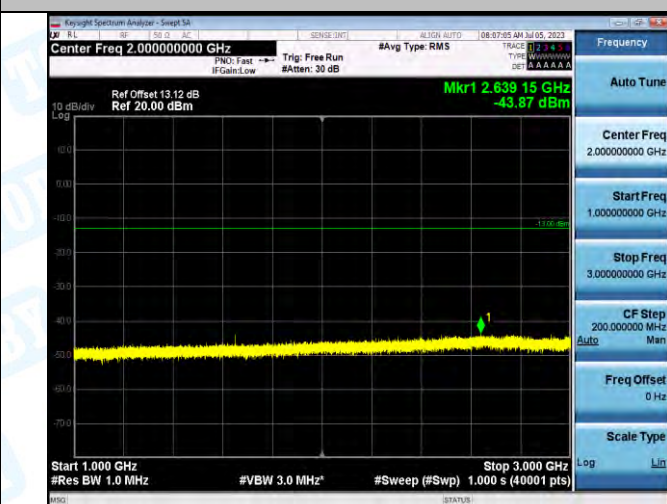
Band5 Band5 5MHz QPSK 20425 1RB#0 1000~3000 1000~3000
