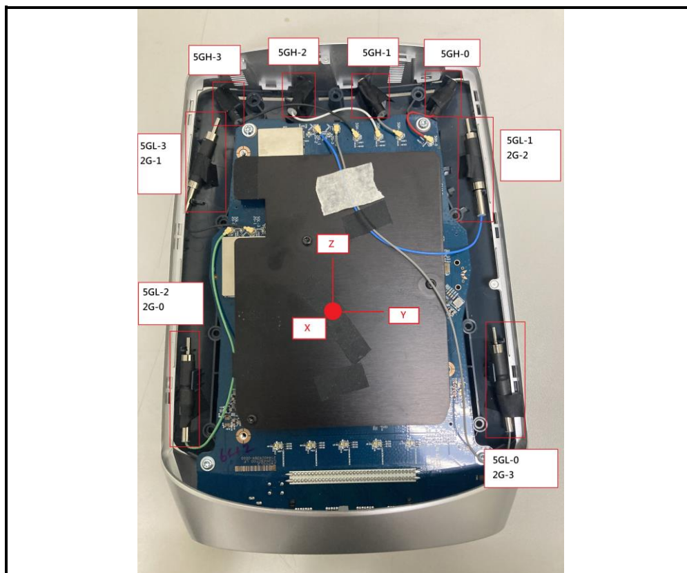
Antenna
