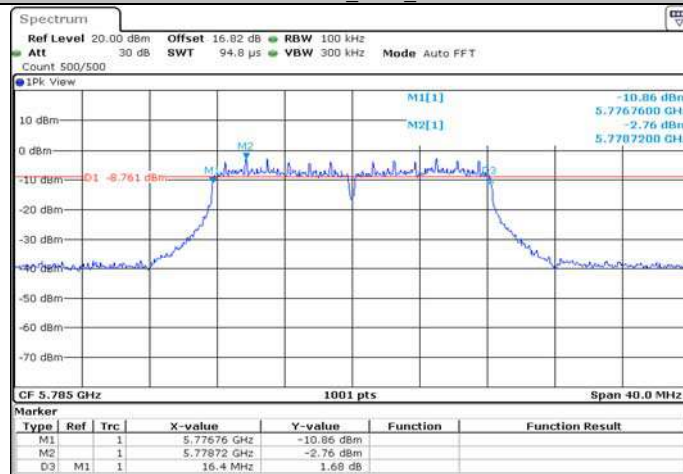
11AMIMO Ant1_5785
