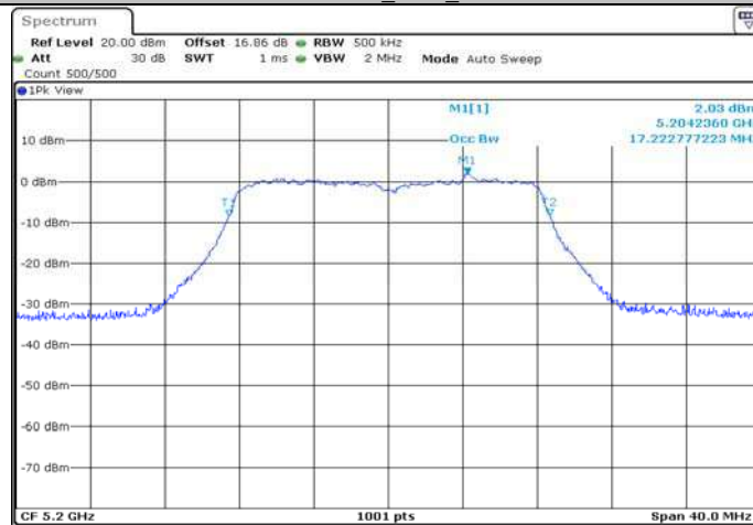
11AMIMO_Ant1_5200
