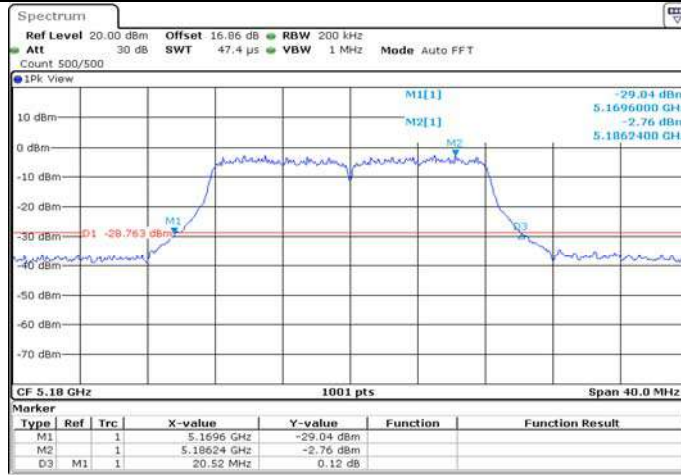
11AMIMO Ant1_5180
