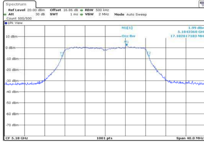
11AMIMO_Ant1_5180
