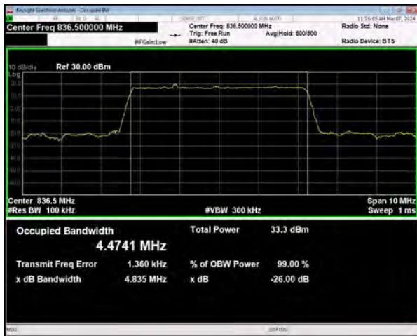
n5 SCS=15kHz DFT_BPSK BW=5MHz Channel=167300 RB=25@0
