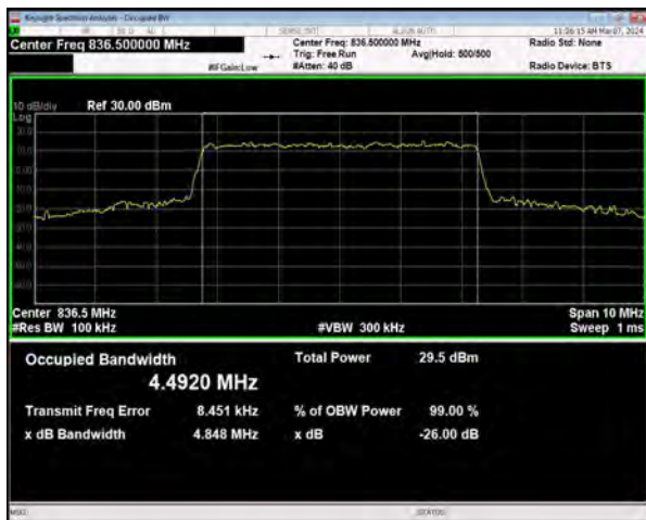
n5 SCS=15kHz CP_16QAM BW=5MHz Channel=167300 RB=25@0
