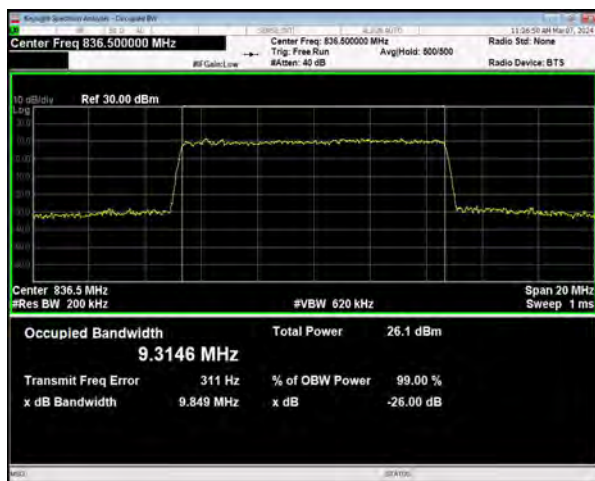
n5 SCS=15kHz CP_256QAM BW=10MHz Channel=167300 RB=52@0
