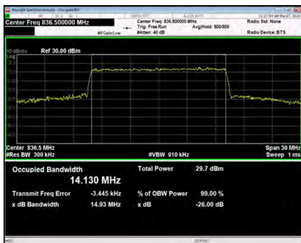
n5 SCS=15kHz CP_QPSK BW=15MHz Channel=167300 RB=79@0
