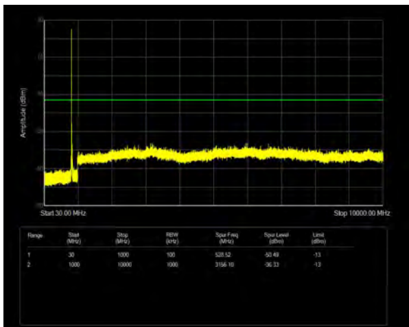
n5 SCS=15kHz DFT_BPSK BW=20MHz Channel=166800 RB=1@0
