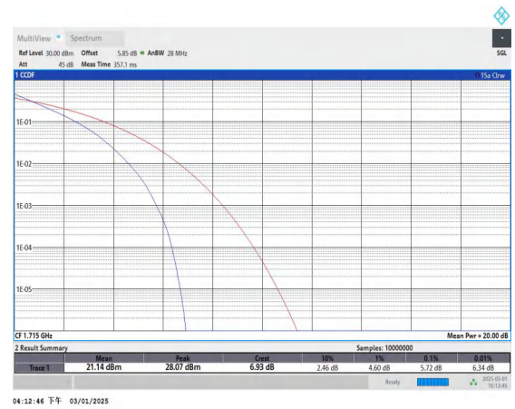
Band4-10MHz-QPSK-20000-50RB#0-PASS
