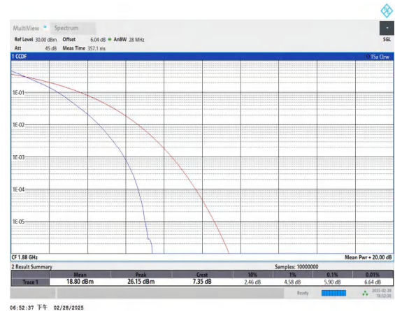
Band2-5MHz-QPSK-18900-25RB#0-PASS
