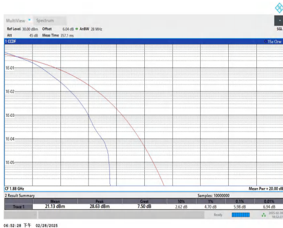
Band2-5MHz-QPSK-18900-1RB#0-PASS
