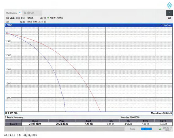
Band2-10MHz-QPSK-18650-50RB#0-PASS
