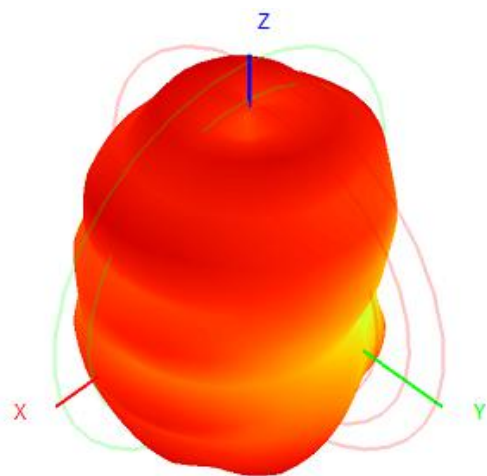
远场方向图
