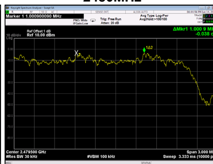
2480MHz
