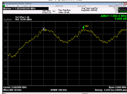
2402MHz
