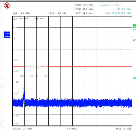
11G-Ant1-2437-30~1000-PASS
