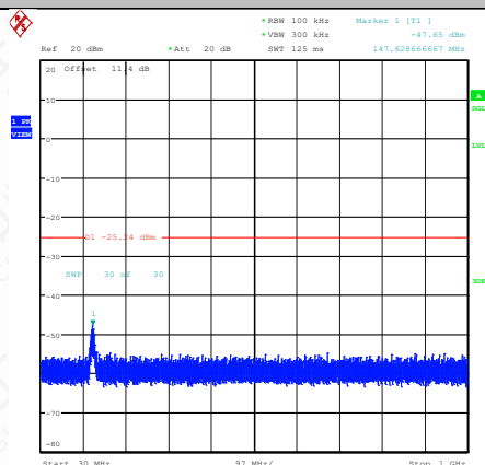
11G-Ant1-2462-30~1000-PASS
