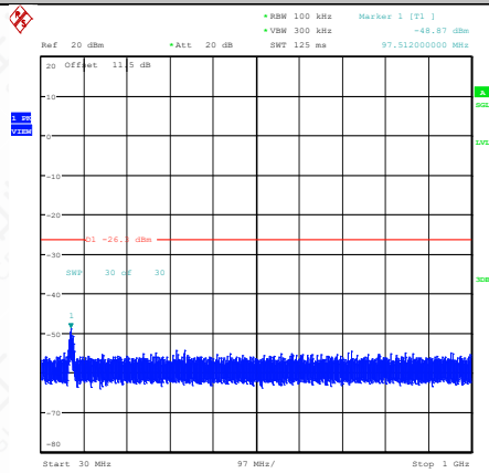
11G-Ant1-2412-30~1000-PASS
