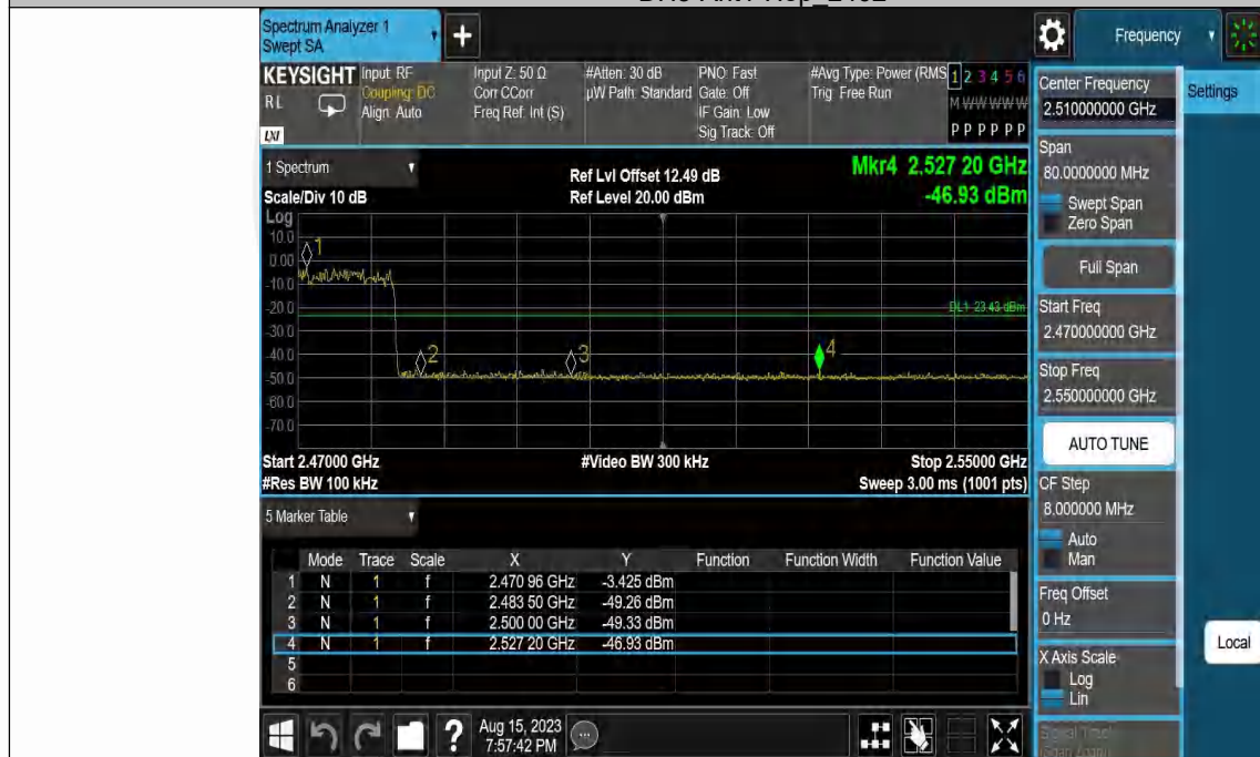
DH5-Ant1-Hop_2480
